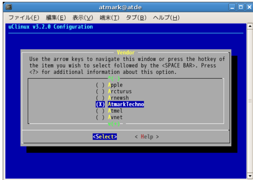
図 4-4 Vendor に AtmarkTechno を選択
