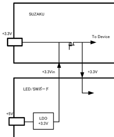
図 5.4. 電源系統
