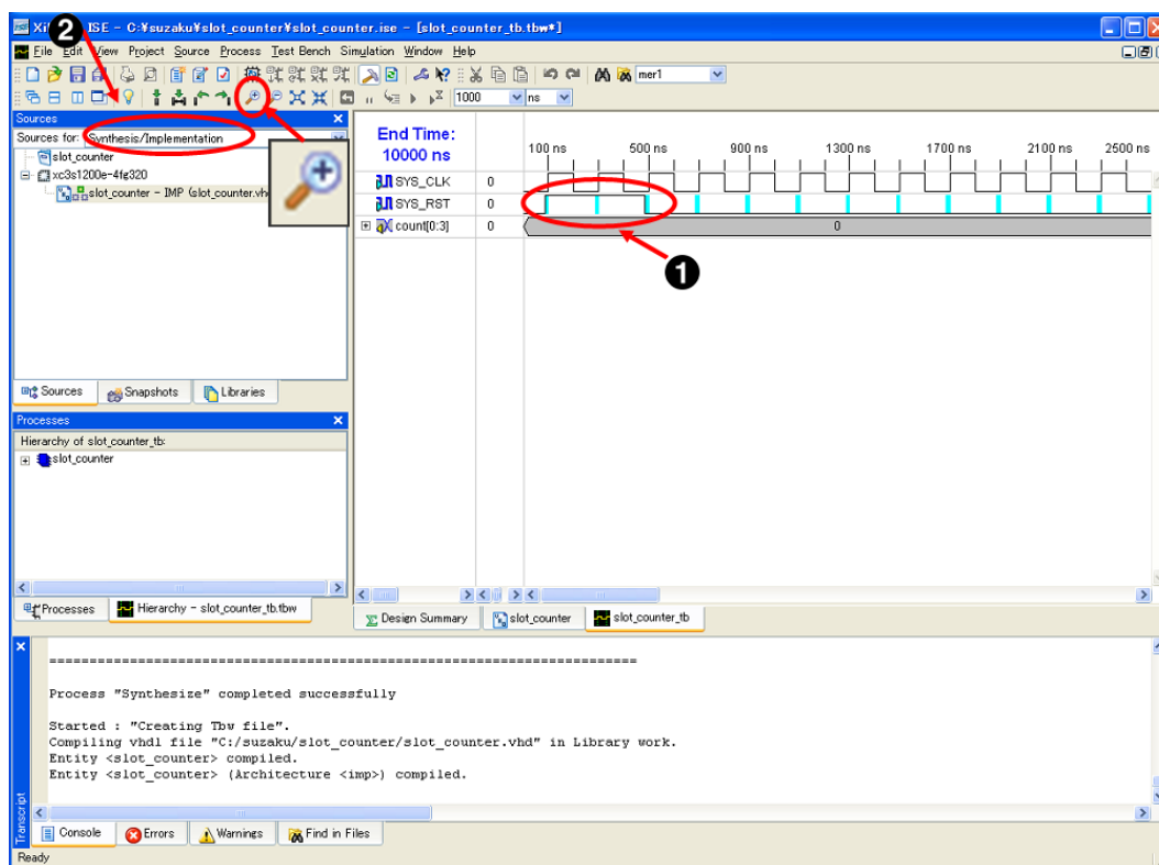
図 8.10. リセット波形生成
