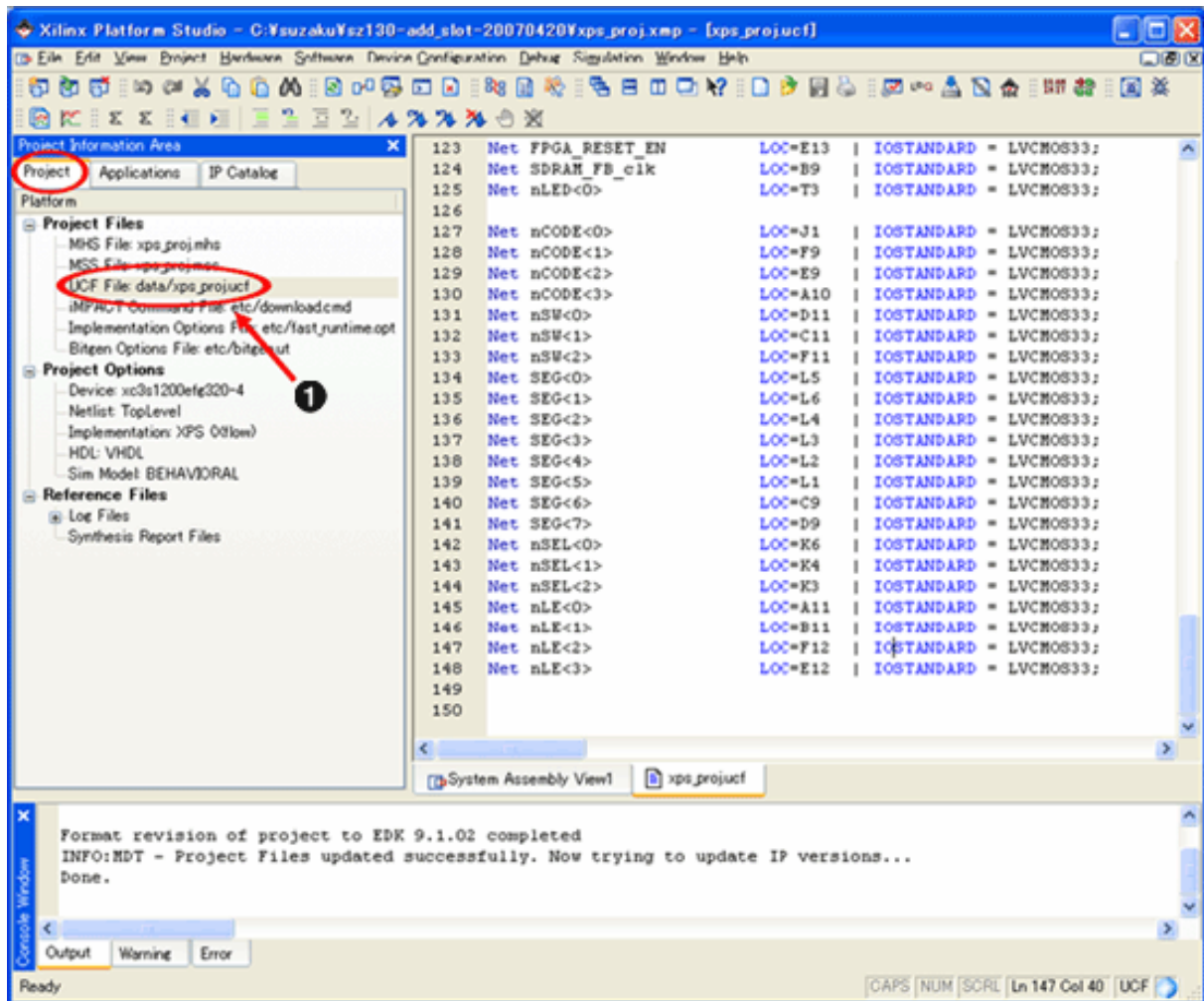
図 11.64. 自作 IP コア(xps_proj.ucf)
