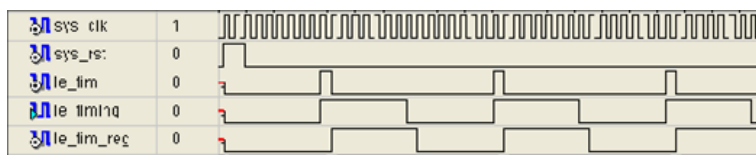
図 9.10. エッジ検出の波形
