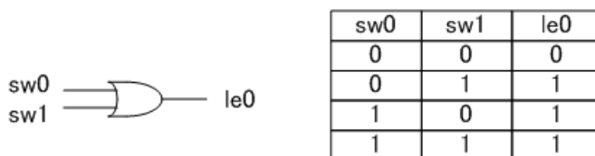
図 8.5. or 回路と真理値表
