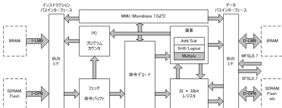
図 1.2. MicroBlaze ブロック図
