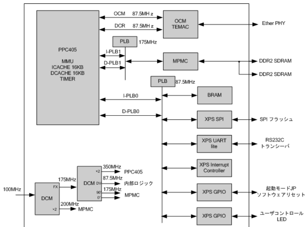
図 10.39. SZ410 デフォルトのブロック図(2008/1/18 以降)
