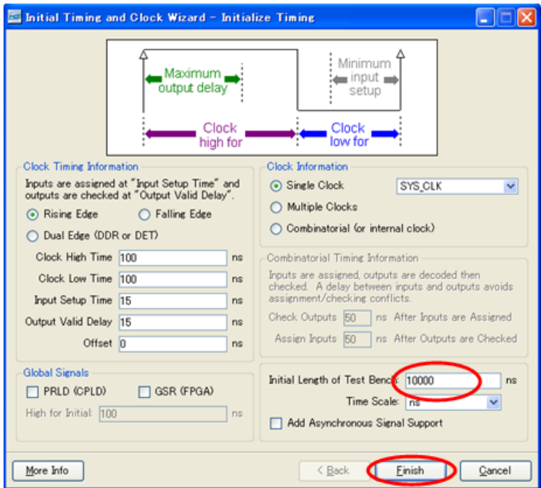
図 8.9. クロック波形作成
