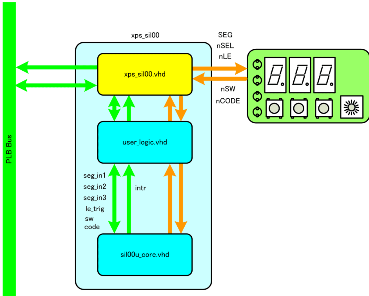
図 11.20. 自作 IP コア
