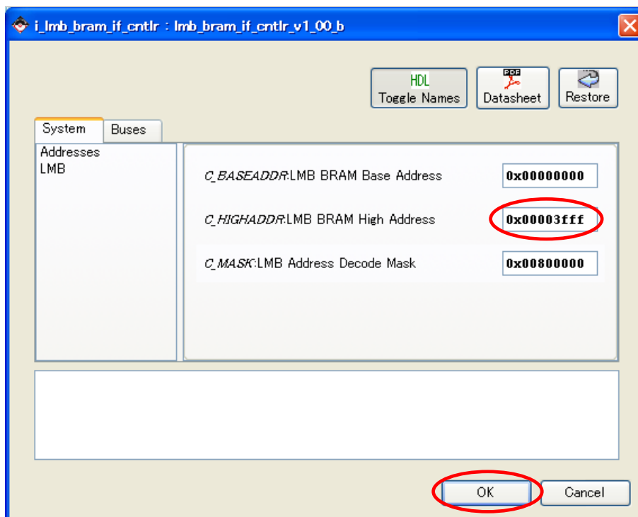
図 11-48 8kByte 16kByte に変更(i_lmb_bram_if_cntlr)
