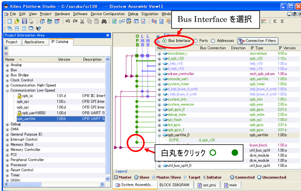
図 10-105 OPB バスに接続
