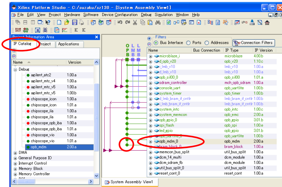
図 11-55 opb-mdm を追加してバスに接続
