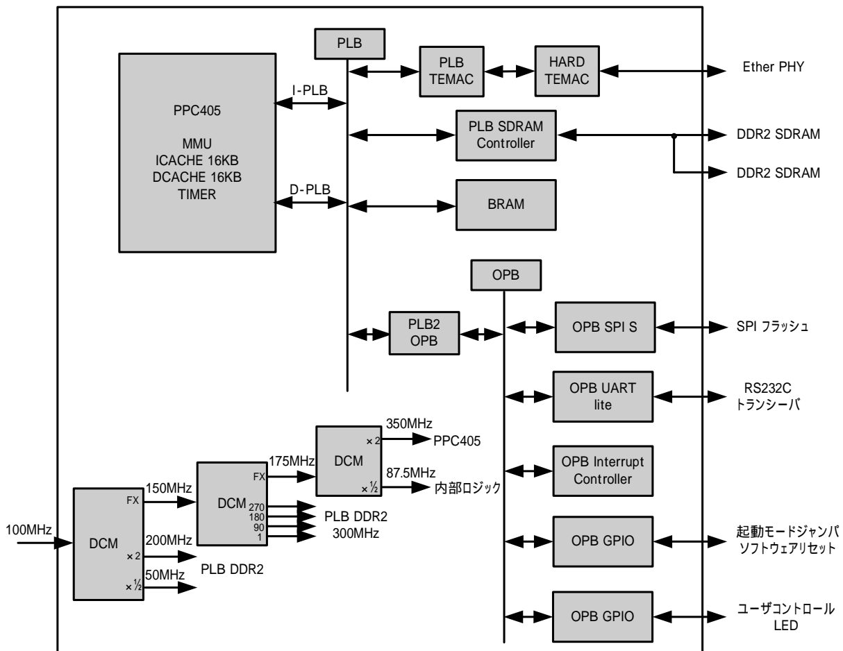
図 10-67 SZ410 デフォルトのブロック図
