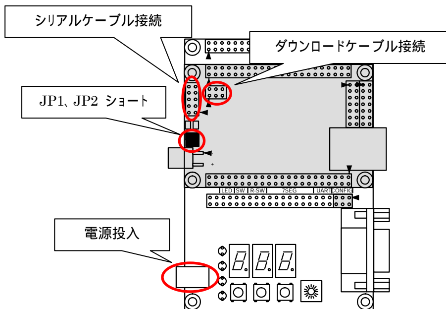
図 11-50 ジャンパの設定等
