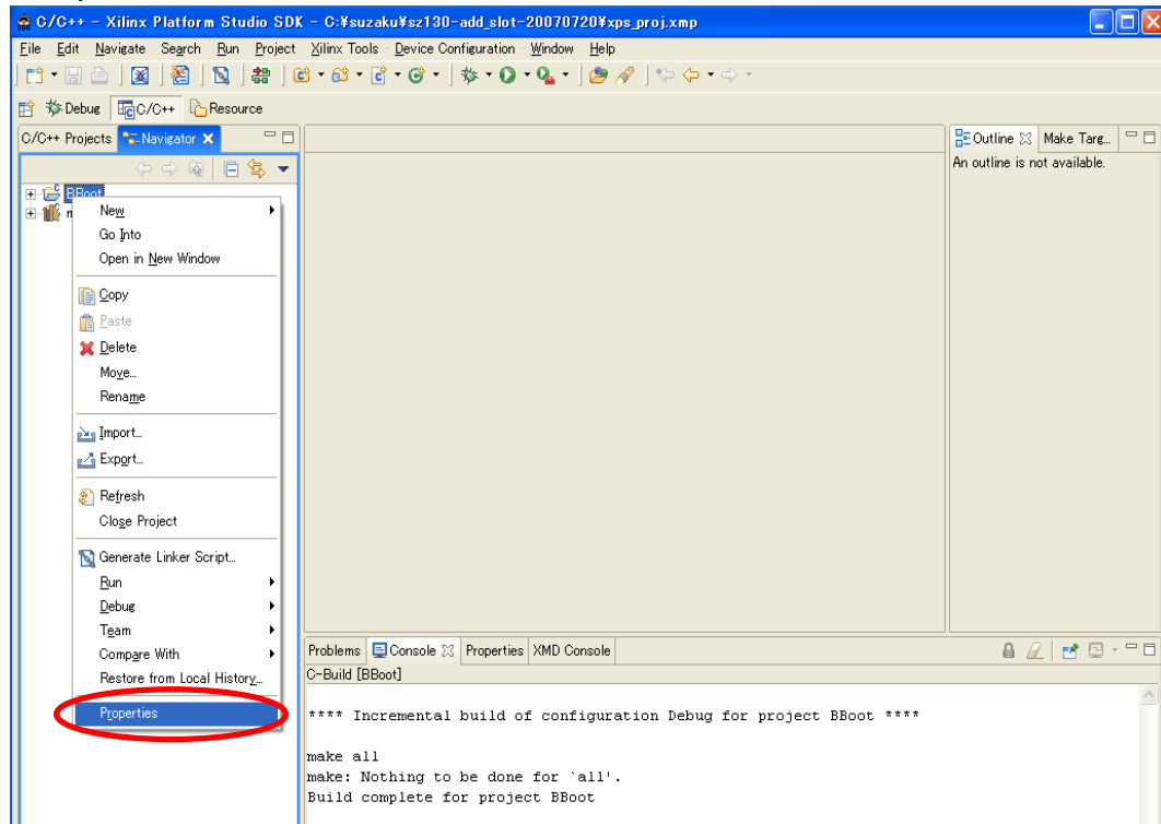
図 12-21 Build 設定
