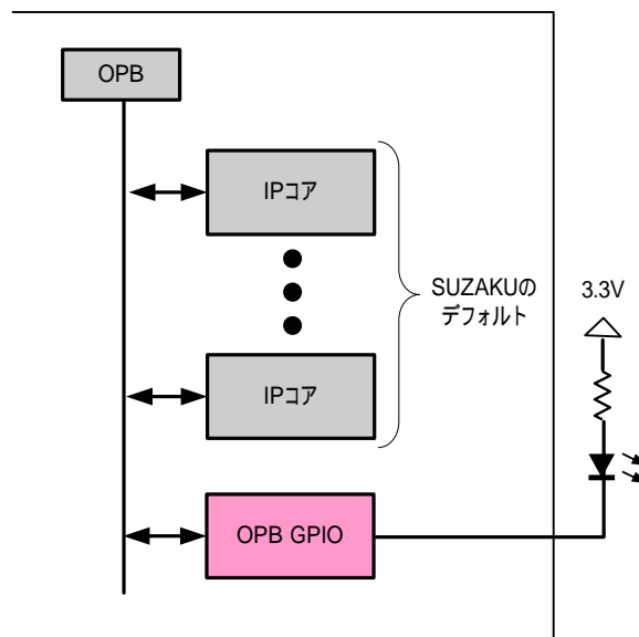
図 10-69 GPIO を追加して LED を点灯
