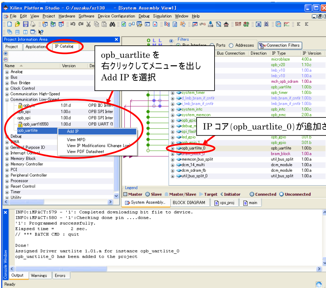
図 10-104 opb_uartlite の追加
