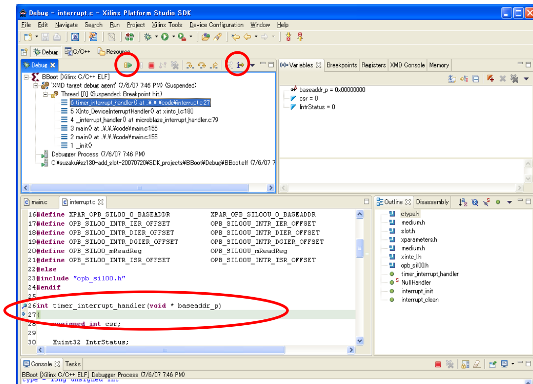
図 12-32 timer_interrupt_handler で Break
