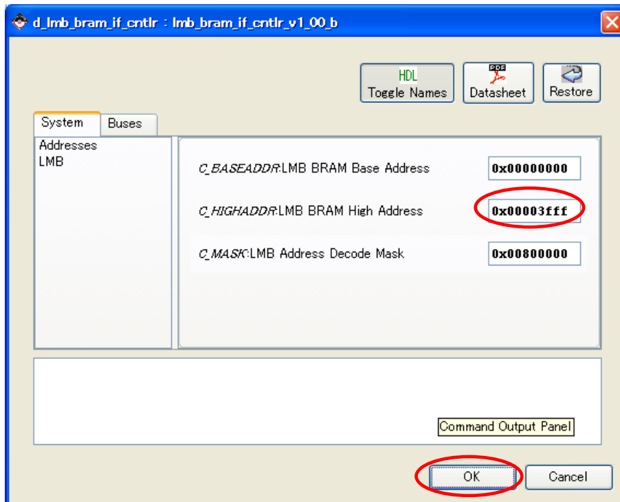
図 11-47 8kByte 16kByte に変更(d_lmb_bram_if_cntlr)
