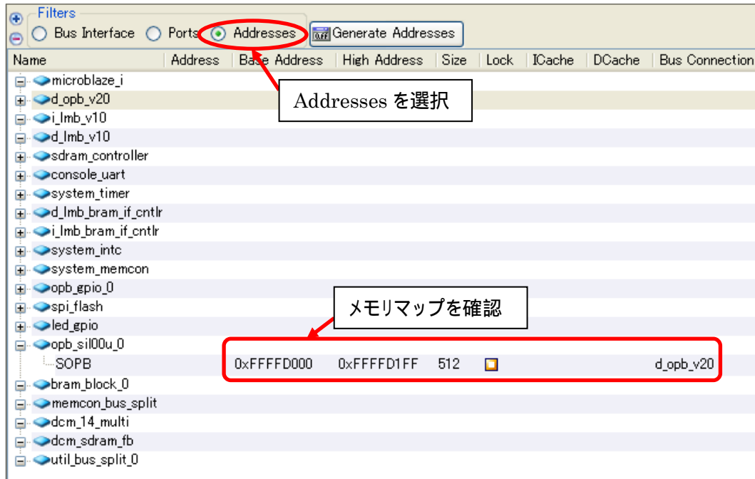
図 11-29 メモリマップ確認
