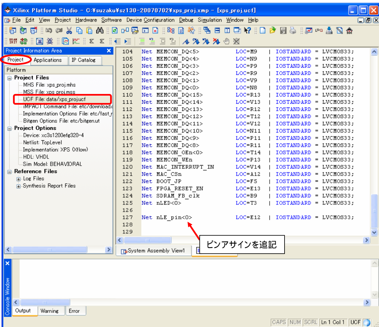
図 10-54 GPIO(xps_proj.ucf)
