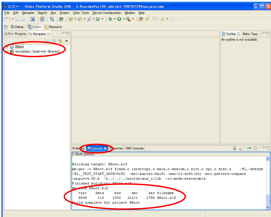
図 12-23 BBoot.elf 作成
