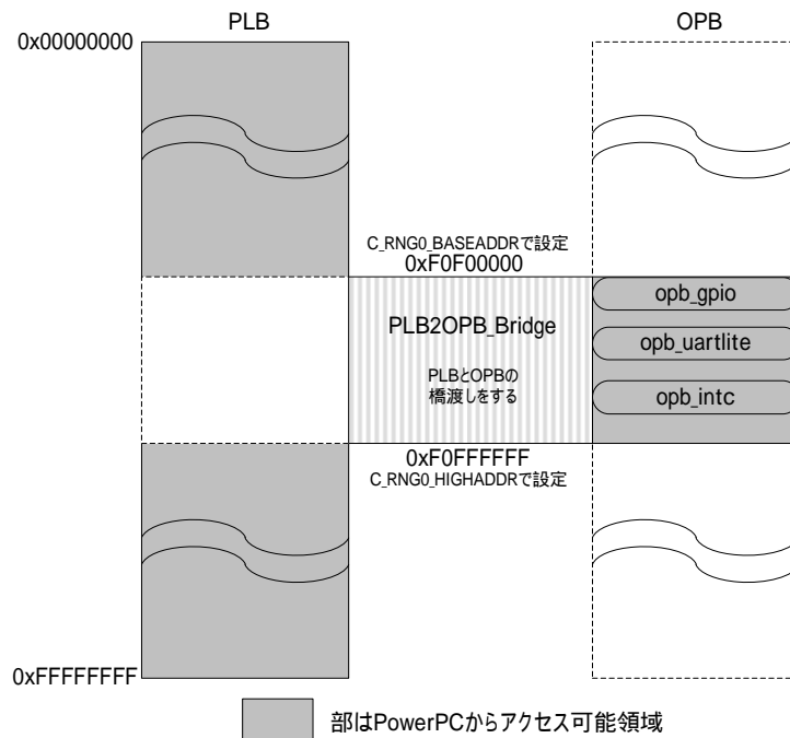
図 10-41 ブリッジ
