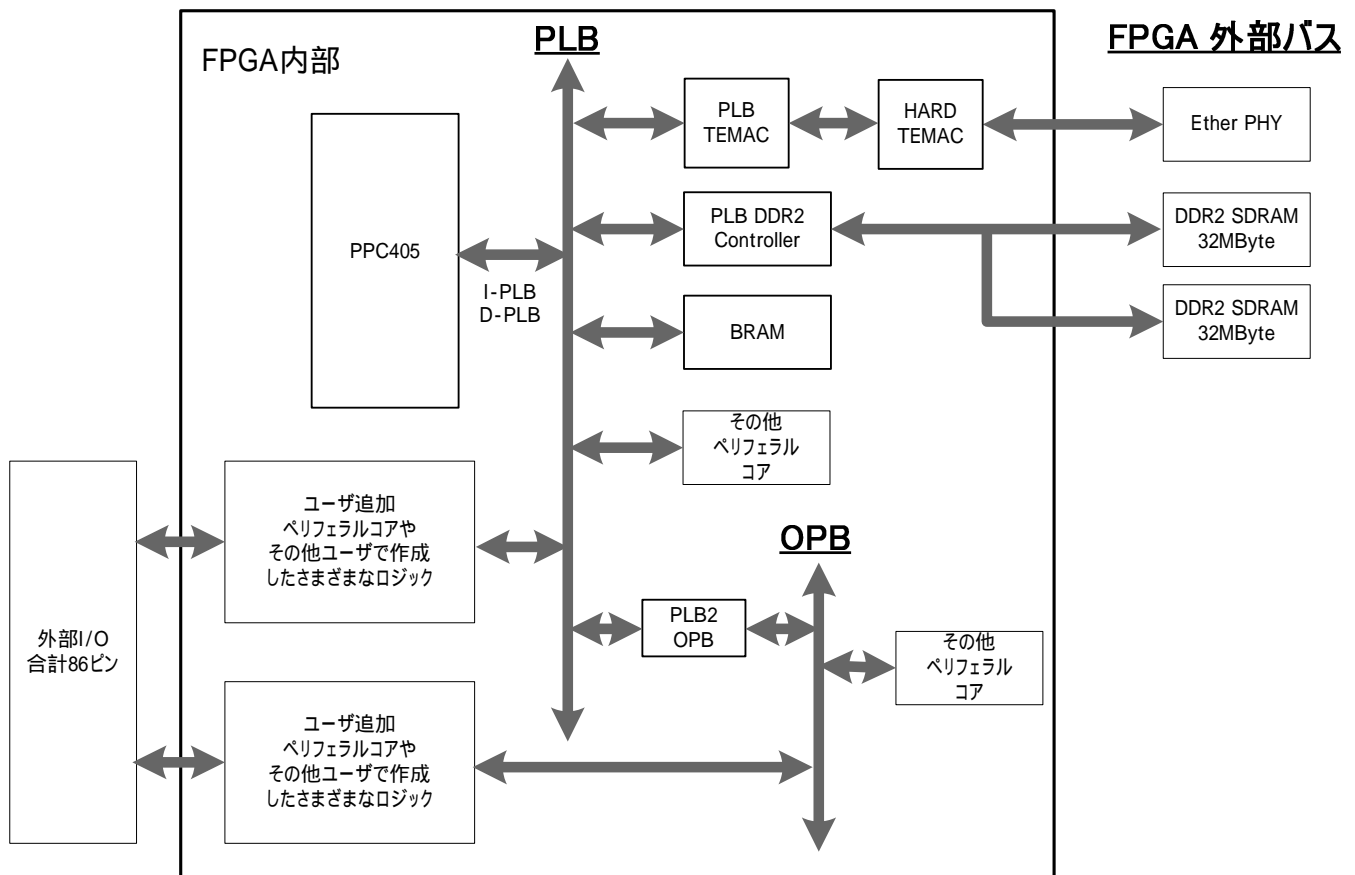
図 1-13 SZ410 のバス
