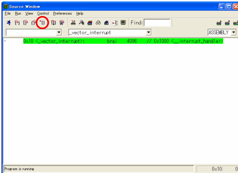
図 11-61 0x10 で Break
