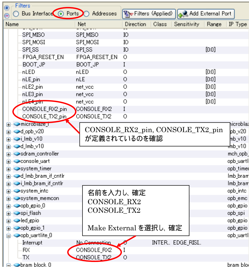
図 10-84 信号の定義
