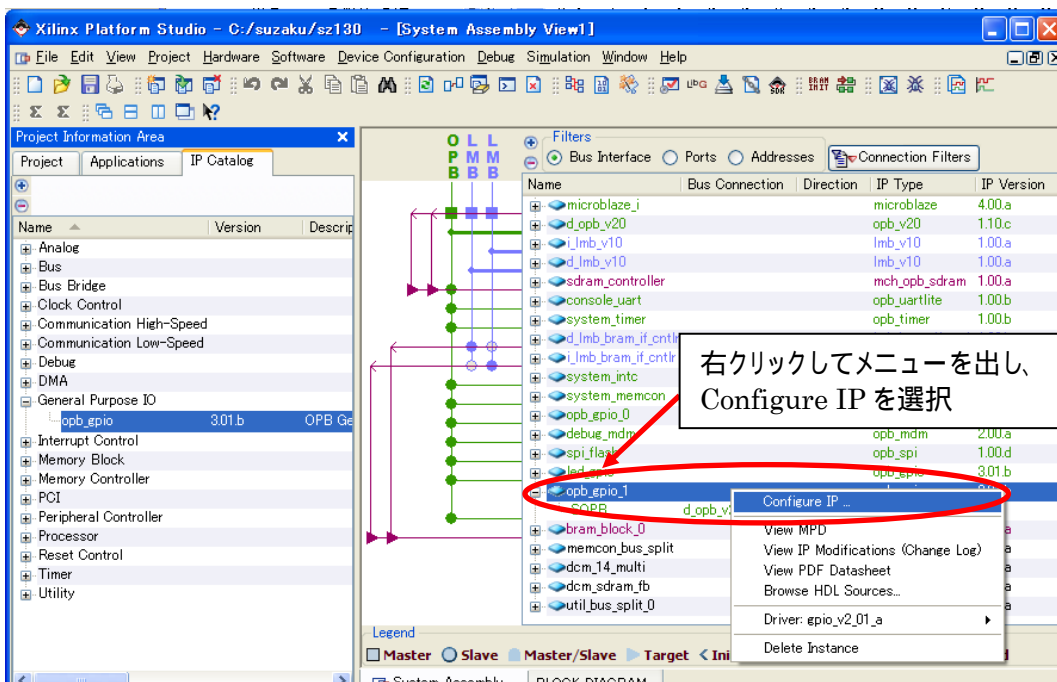
図 10-45 Configure IP
