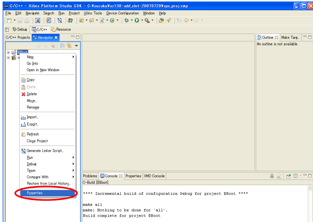
図 12-21 Build 設定
