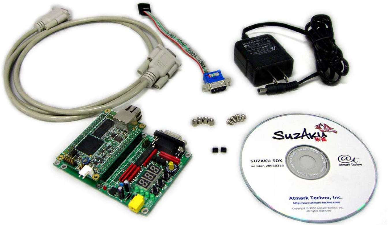
図 4-1 SUZAKU スターターキット(SZ130)
