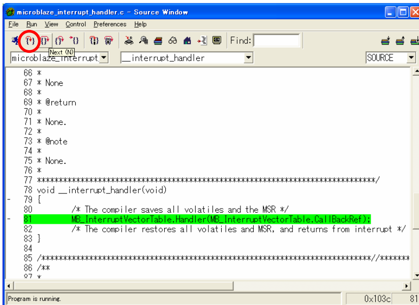
図 11-62 __interrupt_handler() で Break
