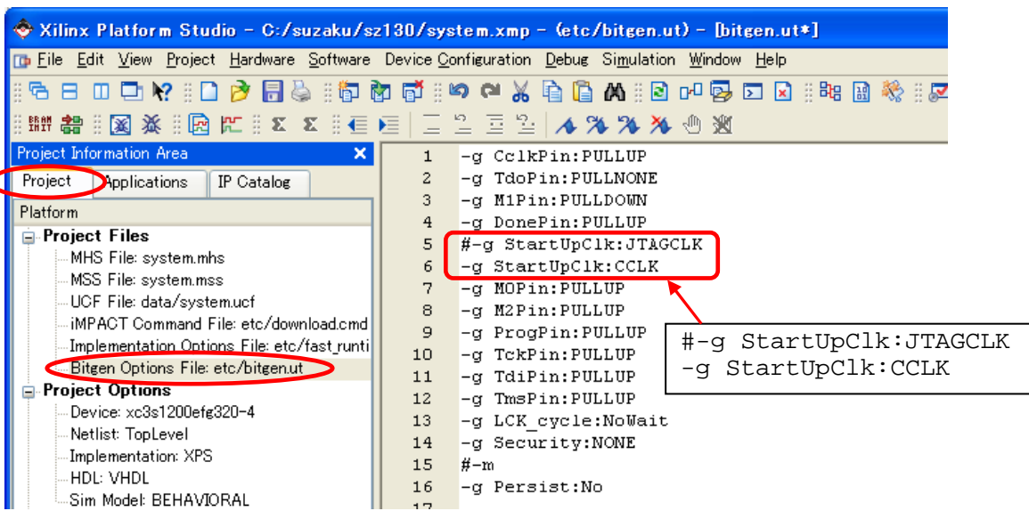
図 10-31 bitgen.ut の変更
