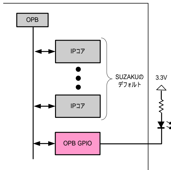
図 10-42 GPIO を追加して LED を点灯
