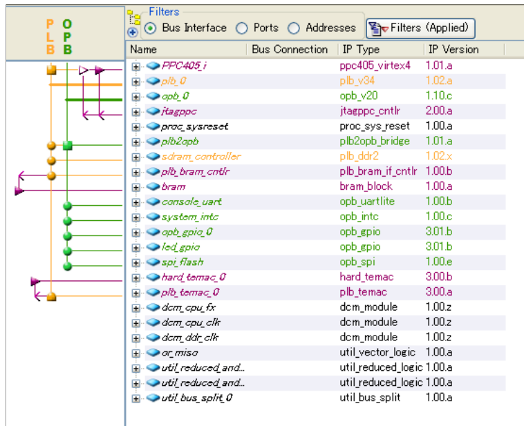
図 10-39 SZ410 のデフォルト(EDK)
