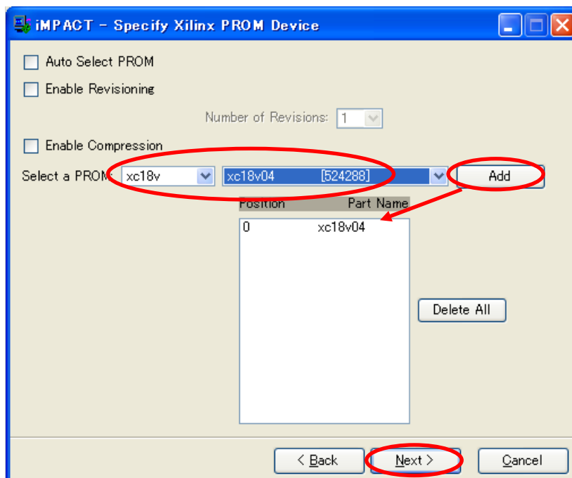
図 6-16 PROM の選択
