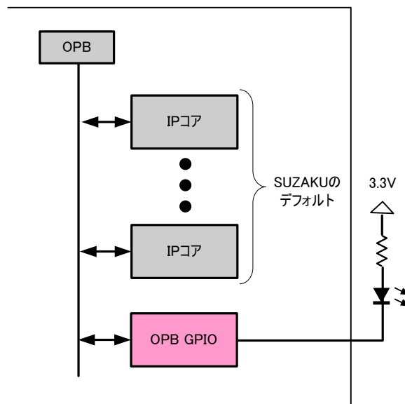
図 10-40 GPIO を追加して LED を点灯
