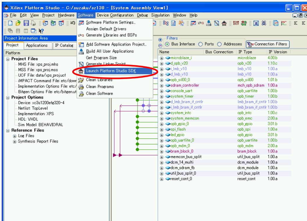
図 12-17 SDK 起動
