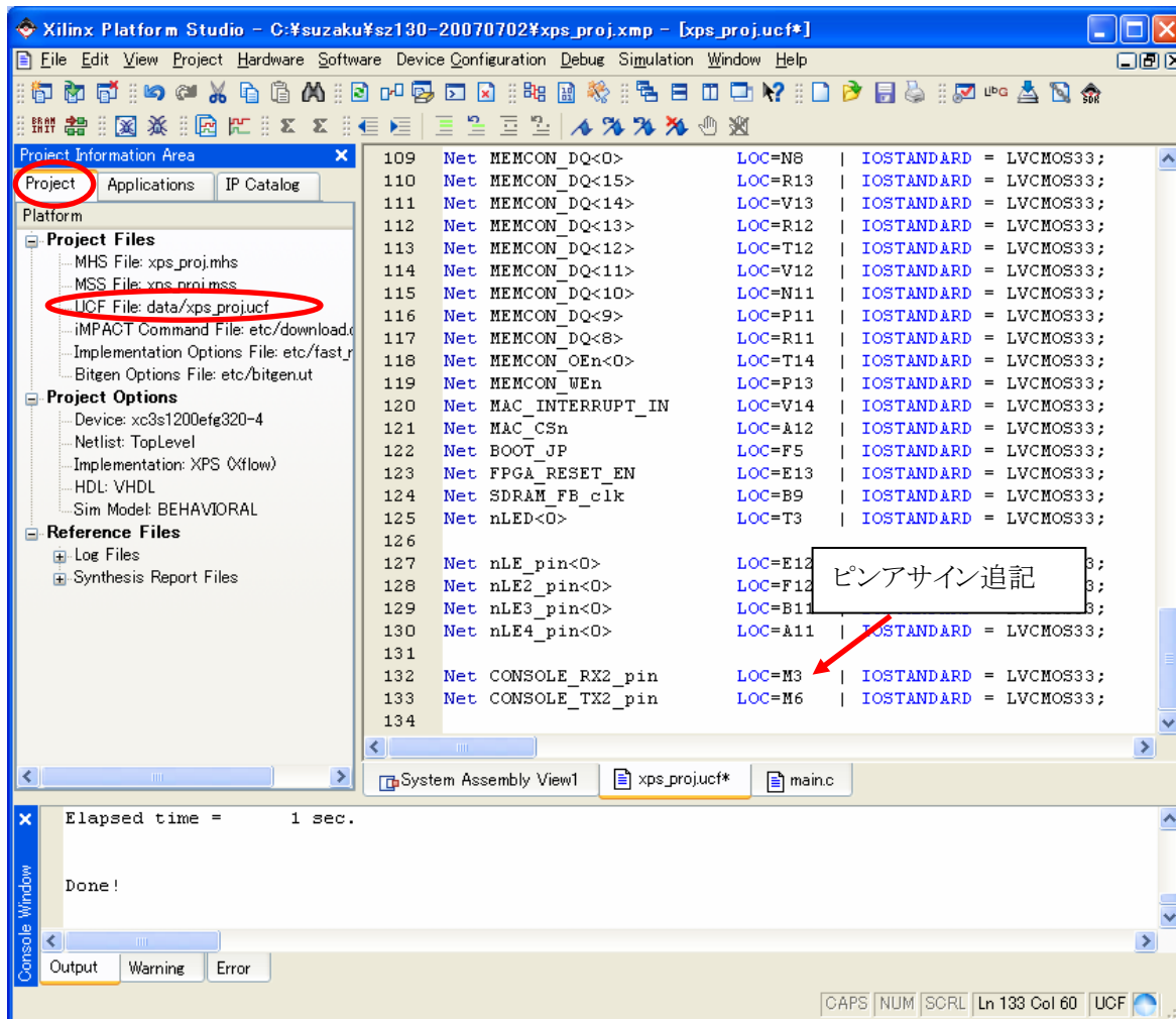
図 10-83 UART(xps_prj.ucf)
