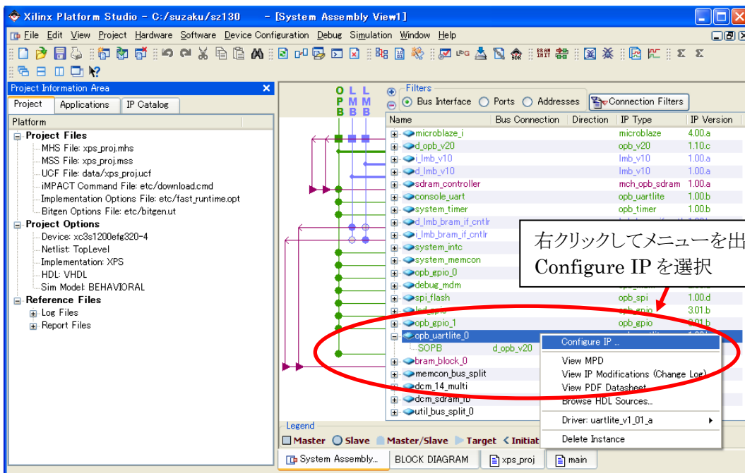
図 10-77 Configure IP
