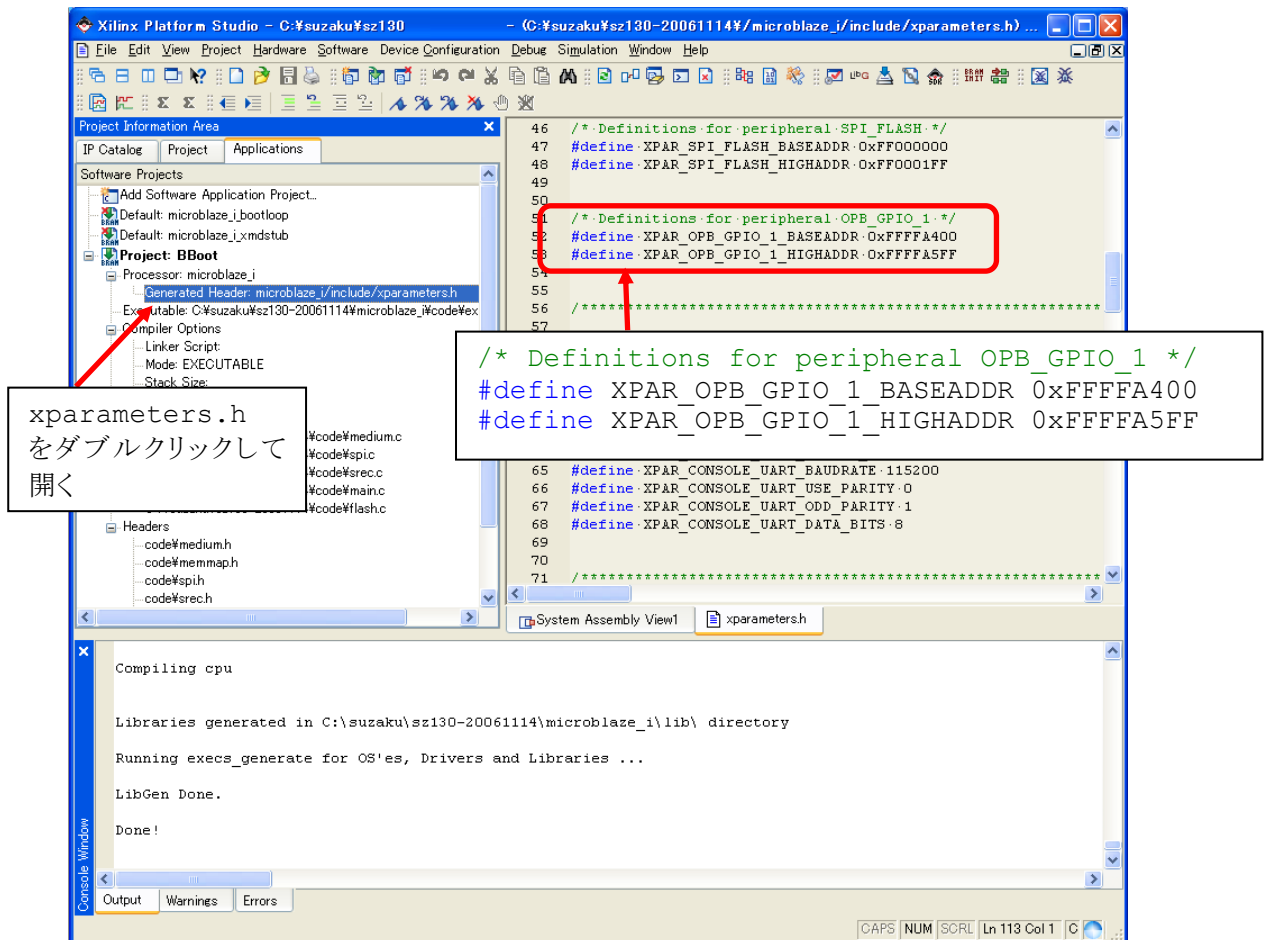
図 10-56 xparameters.h
