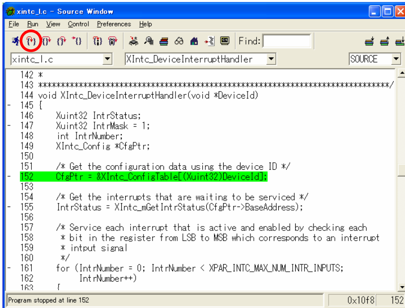
図 11-62 XIntc_DeviceInterruptHandler( )で Break
