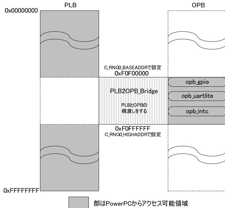
図 10-39 ブリッジ
