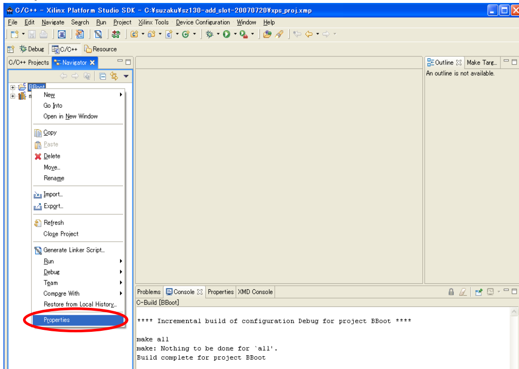
図 12-21 Build 設定
