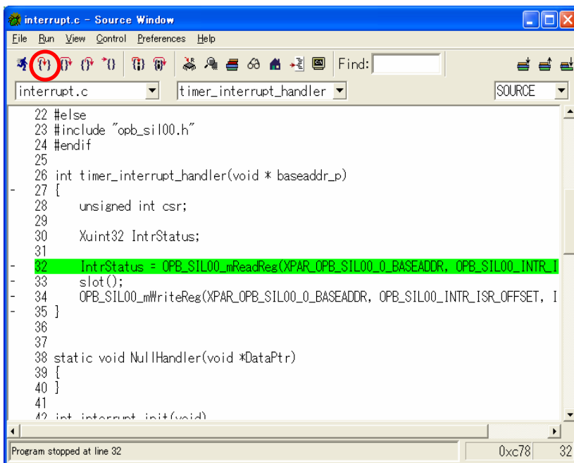
図 11-63 timer_interrupt_handler()で Break
