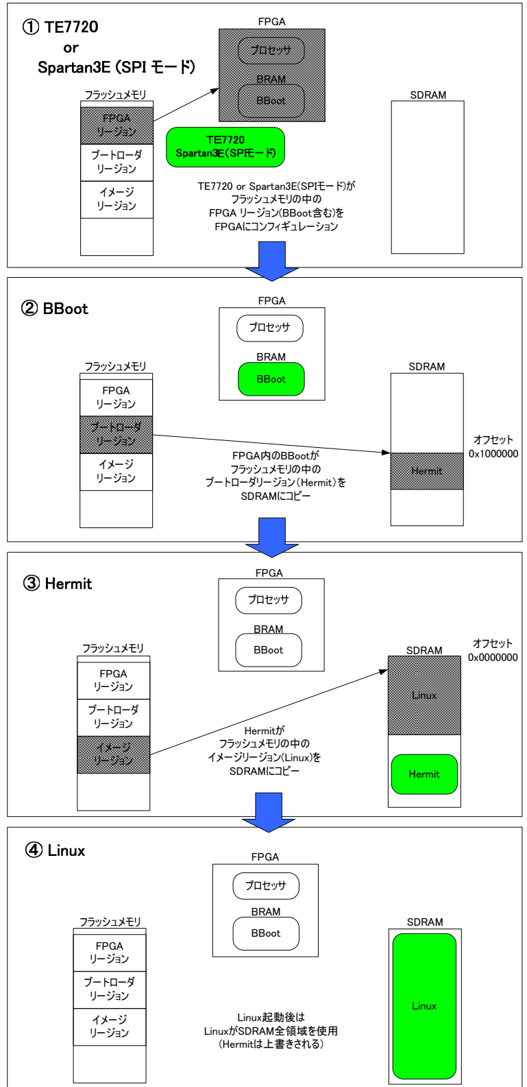
図 5-11 2 段階ブート
