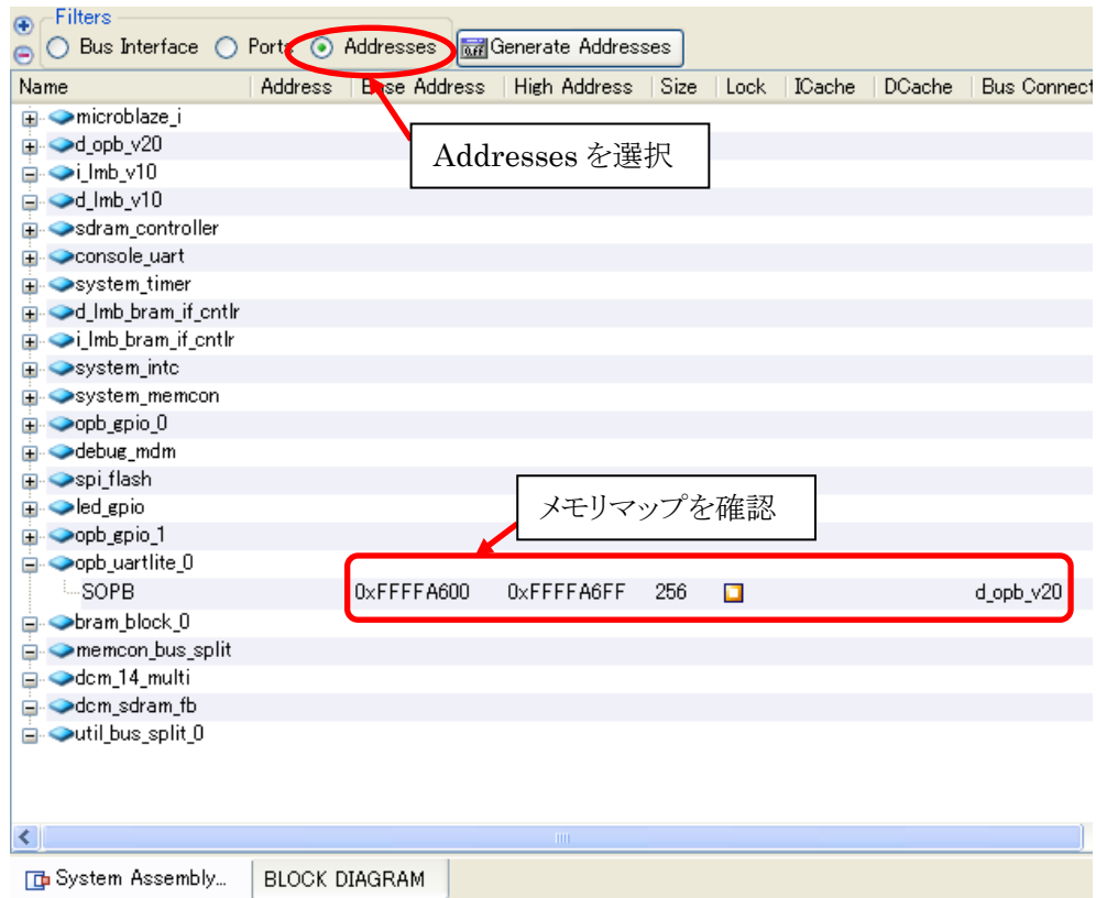
図 10-81 メモリマップ確認
