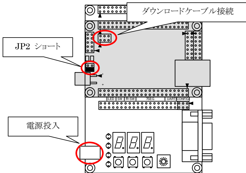
図 10-69 ジャンパの設定等
