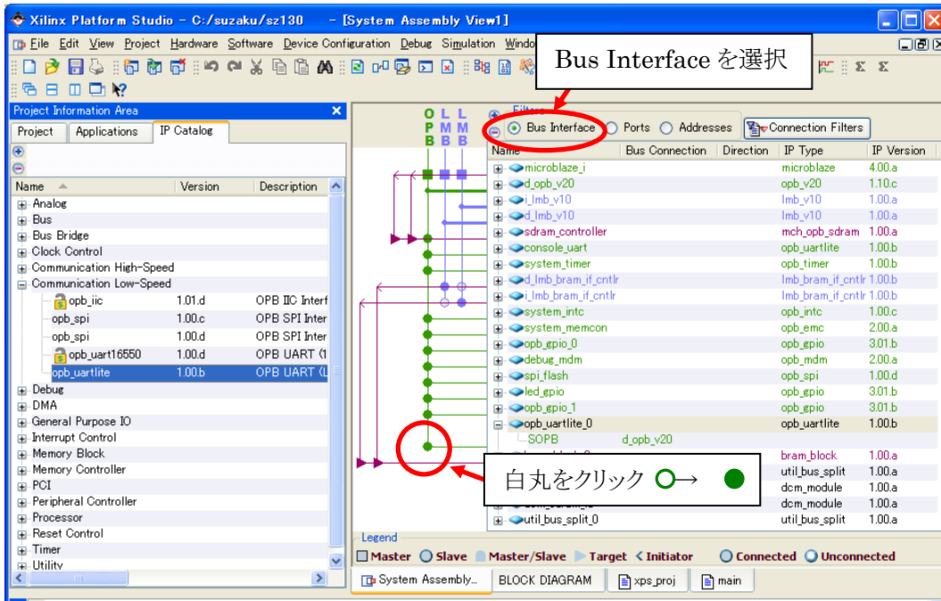
図 10-76 OPB バスに接続
