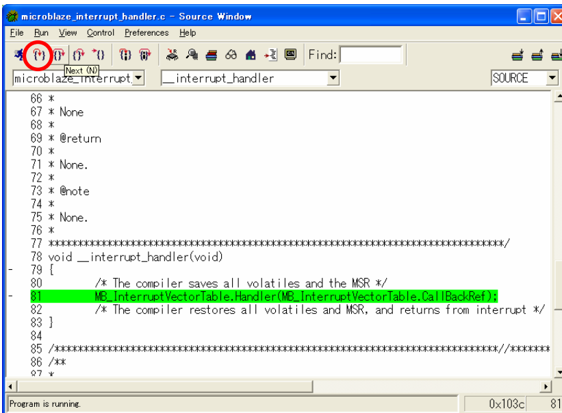
図 11-61 __interrupt_handler()で Break
