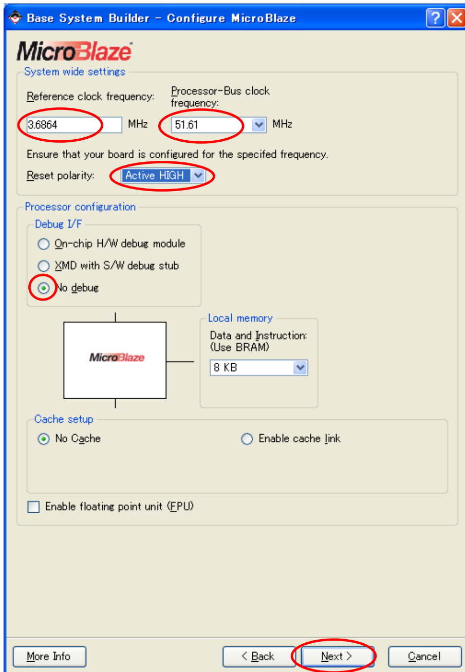
図 10-9 MicroBlaze の設定
