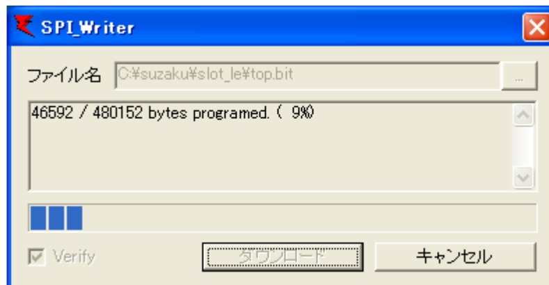
図 6-33 書き込み中
