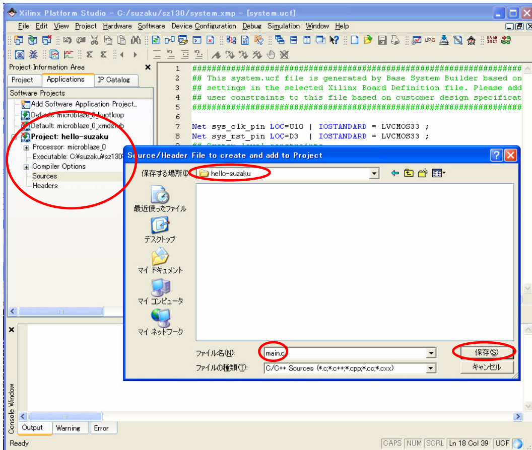
図 10-25 main.c 作成
