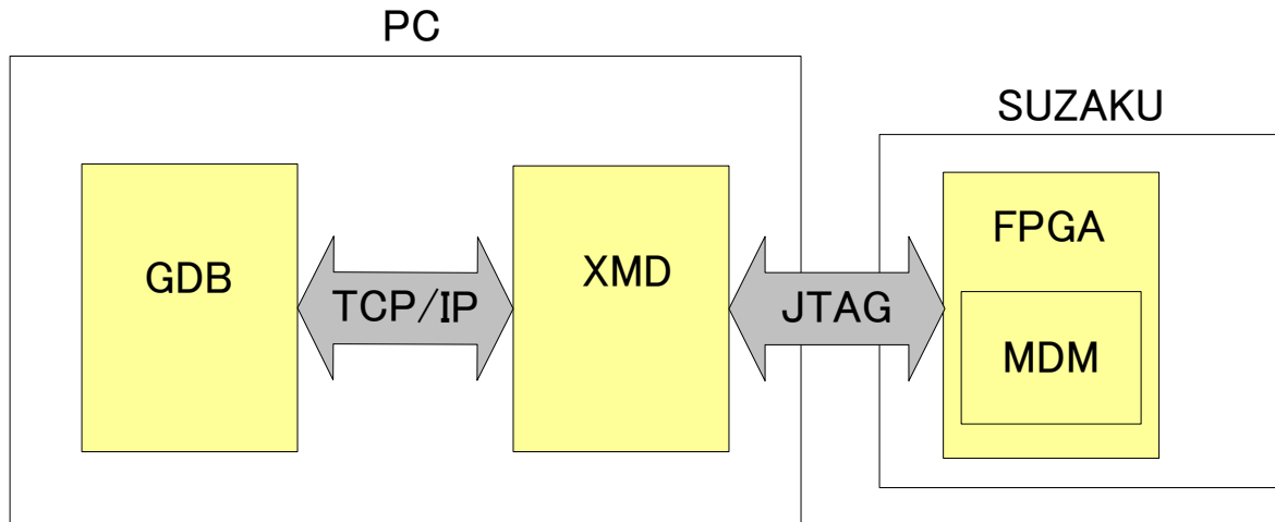
図 11-57 XMD の接続
