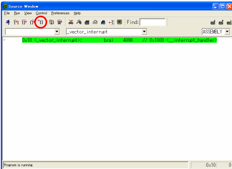
図 11-60 0x10 で Break
