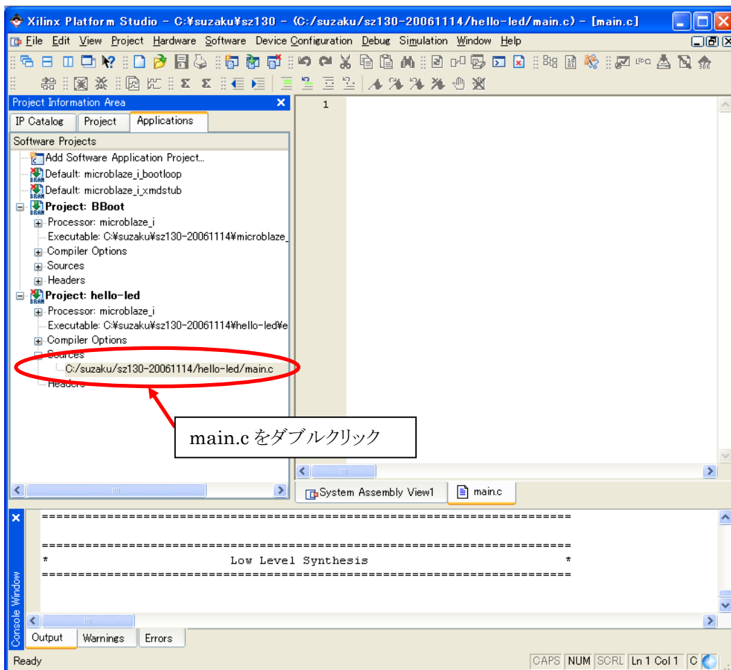
図 10-61 main.c を開く
