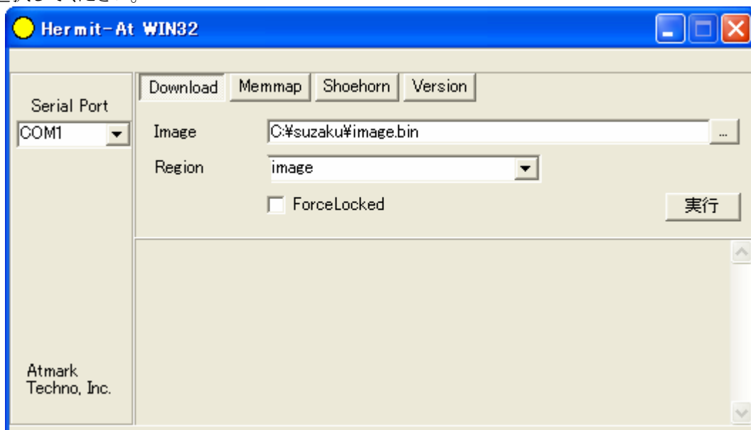
図 6-41 Download 画面
