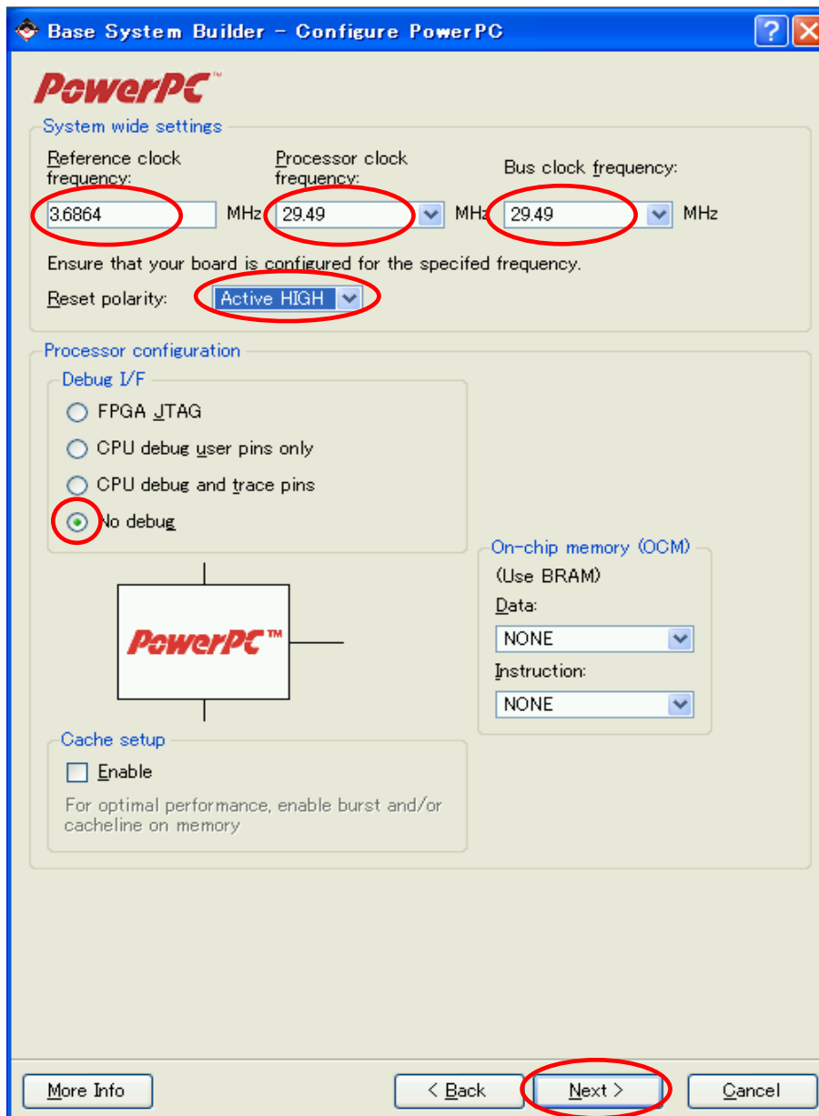
図 10-10 PowerPC の設定
