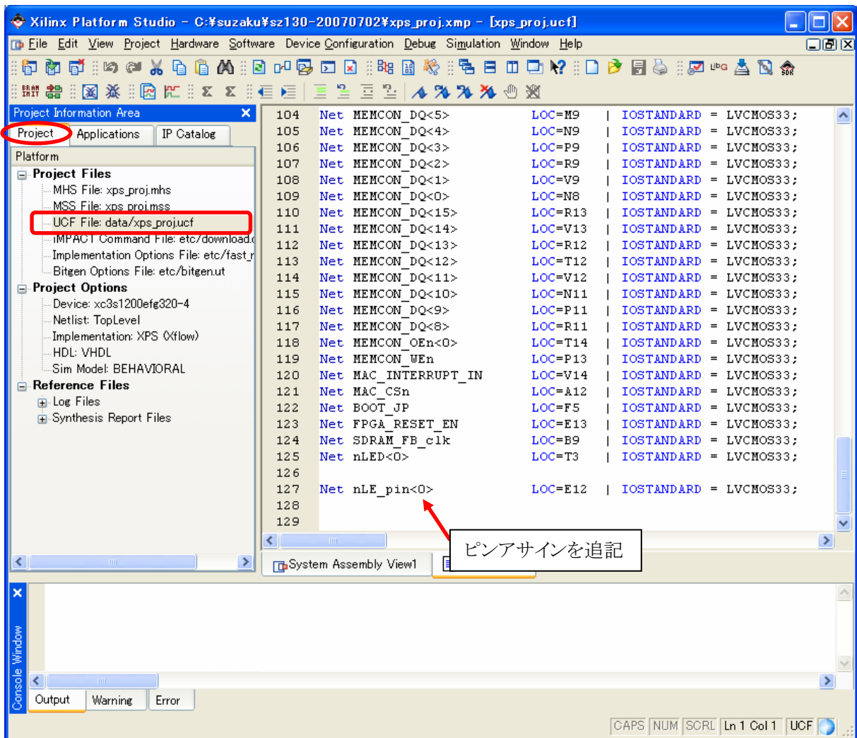
図 10-52 GPIO(xps_proj.ucf)
