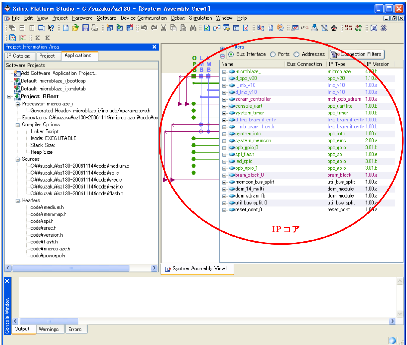
図 10-32 XPS 起動
