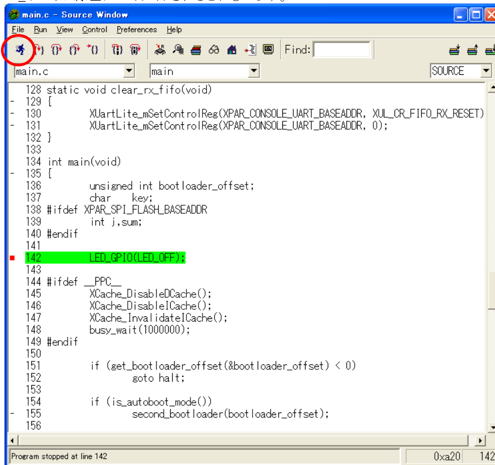
図 11-59 main で Break
