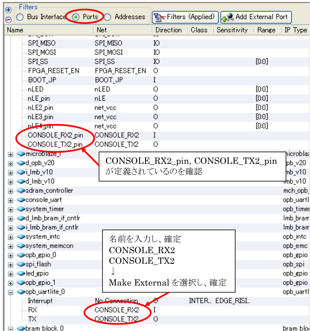
図 10-82 信号の定義
