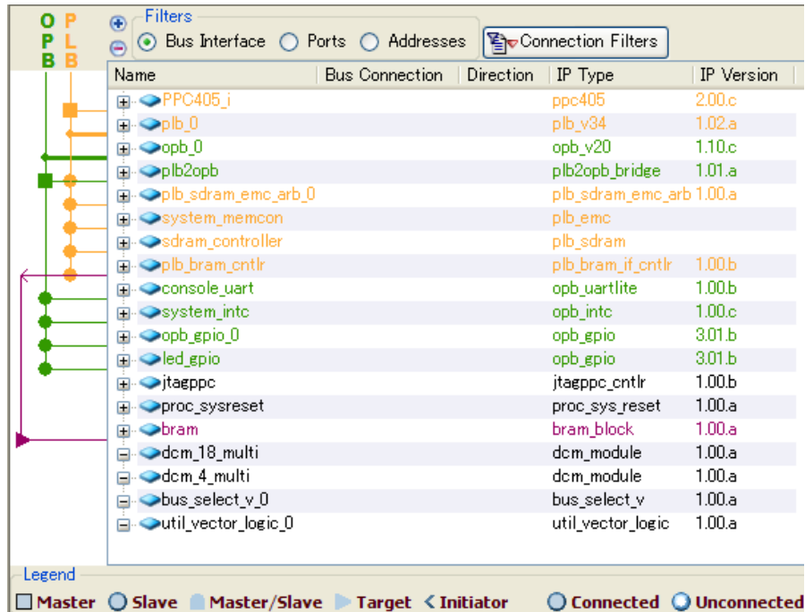
図 10-37 SZ310 のデフォルト(EDK)
