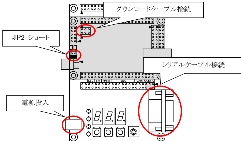
図 10-87 ジャンパの設定等
