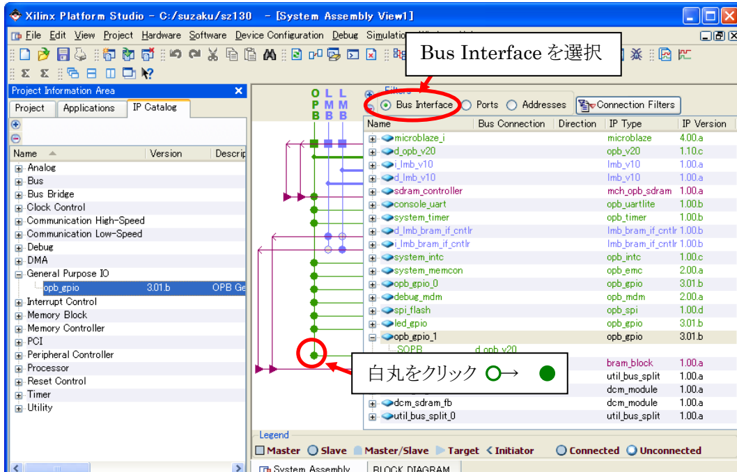
図 10-42 OPB バスに接続
