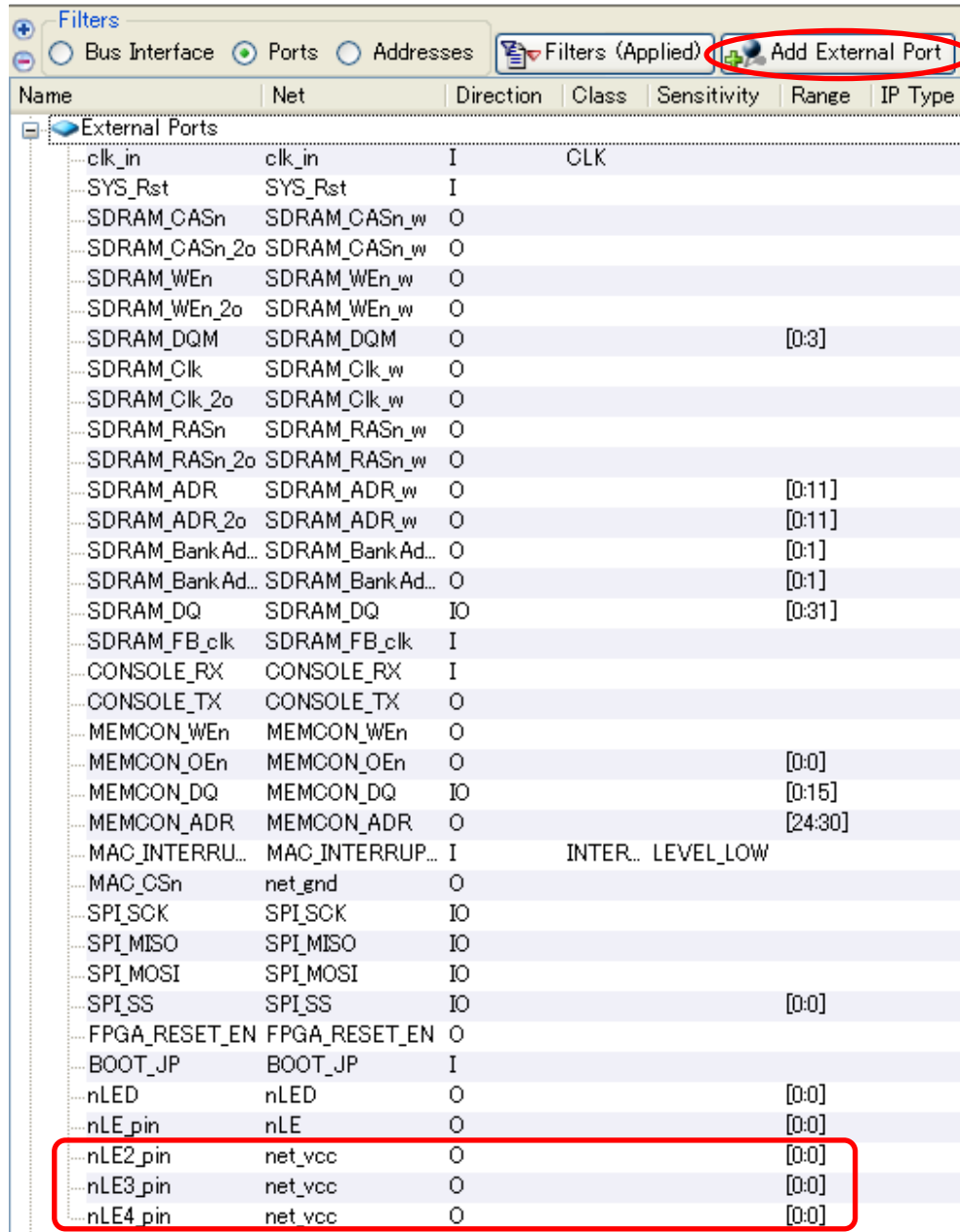
図 10-73 EDK での空きピンの処理
