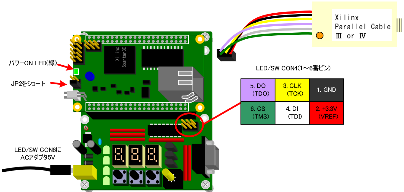
図 6-27 SPI Writer 書き込み準備
