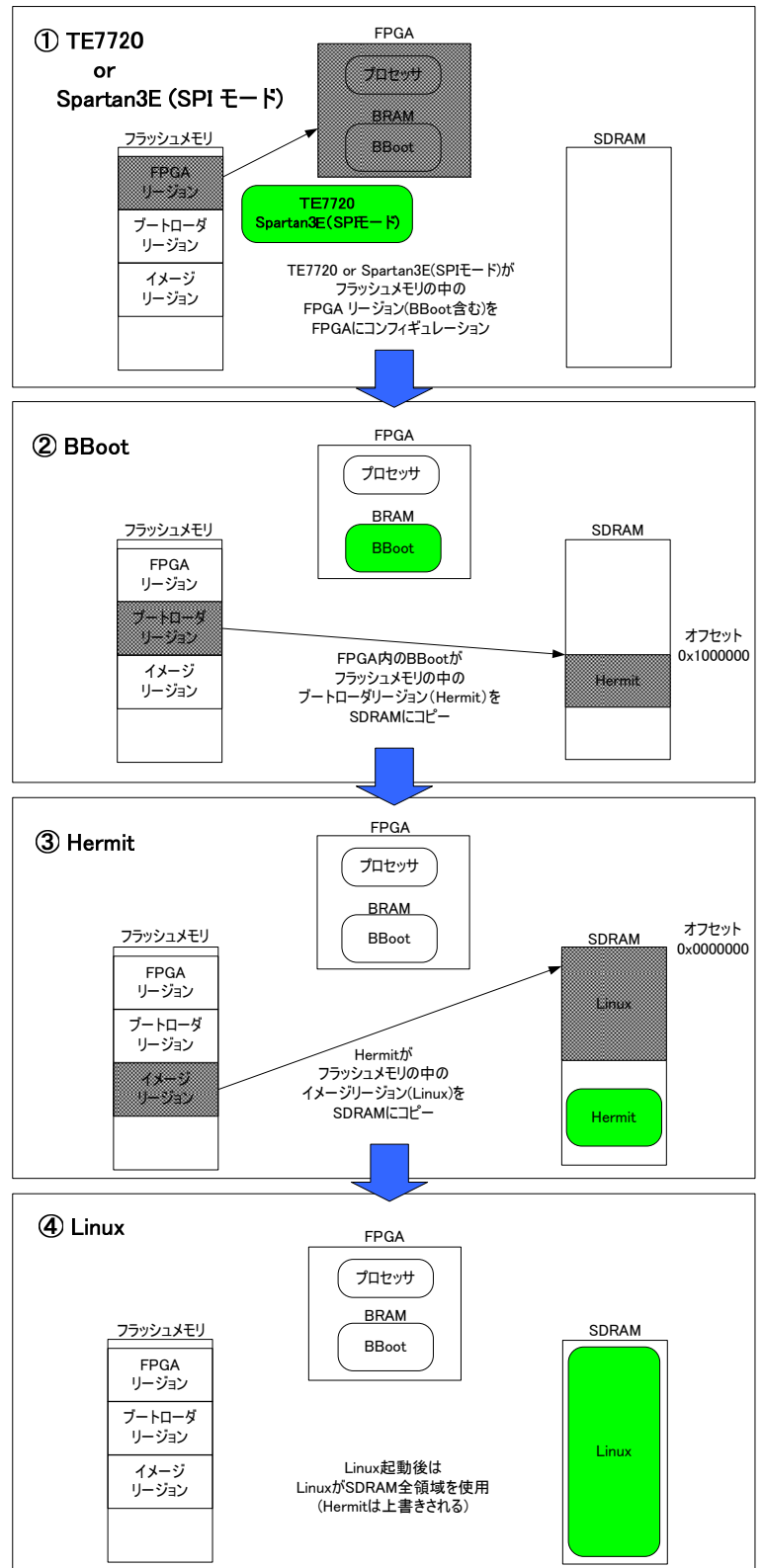
図 5-11 2 段階ブート
