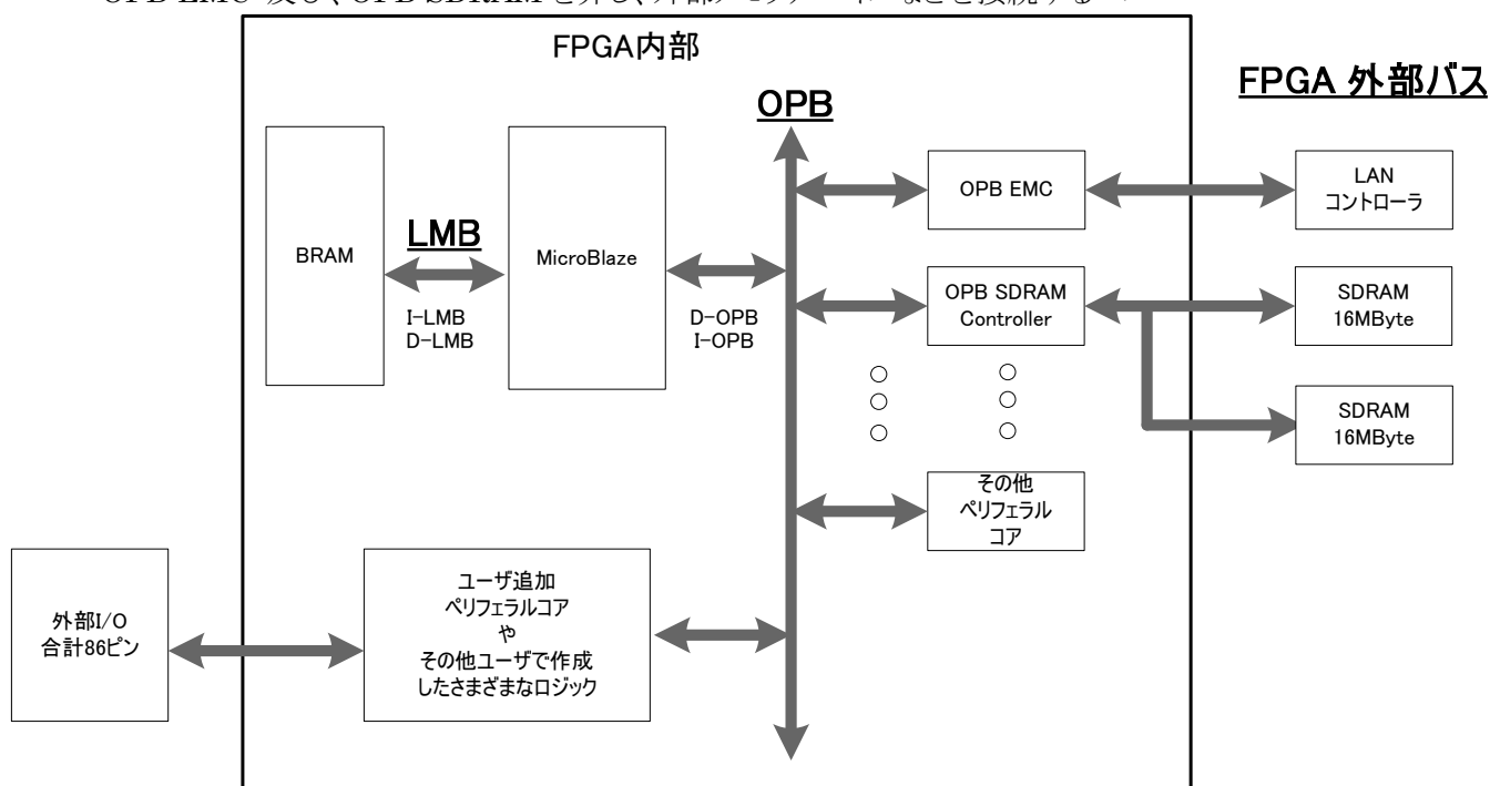
図 1-7 SZ130 のバス
