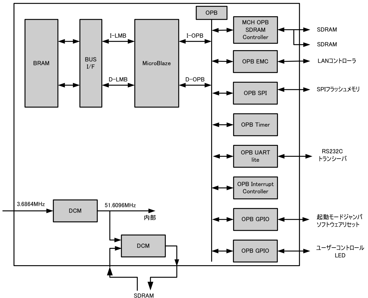
図 10-35 SZ130 デフォルトのブロック図
