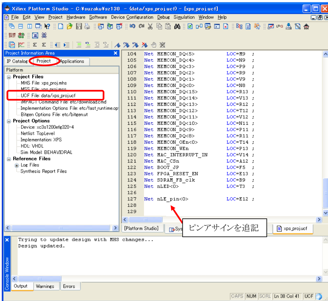
図 10-51 GPIO(xps_proj.ucf)
