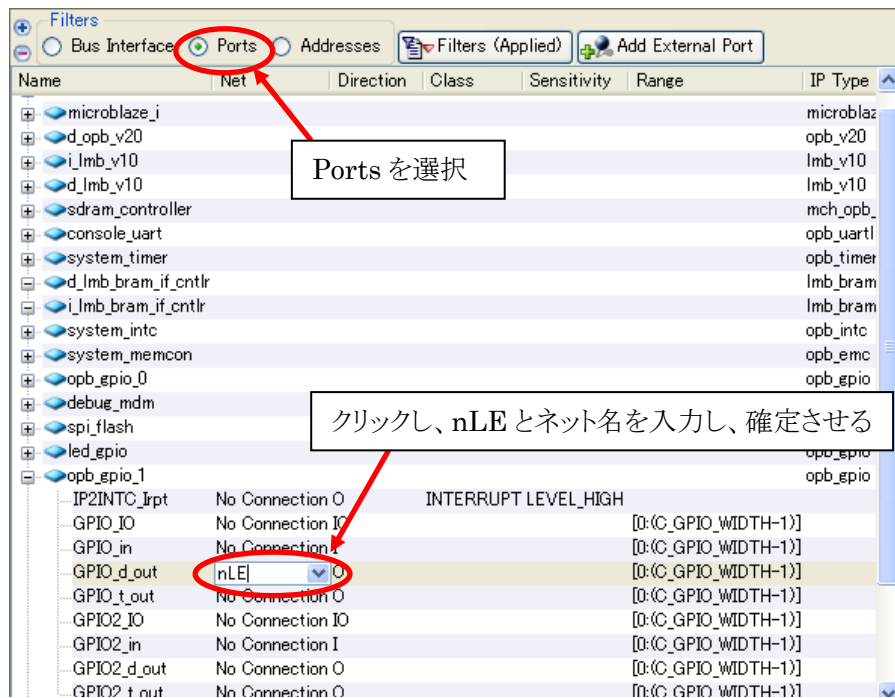
図 10-48 Net 名入力
