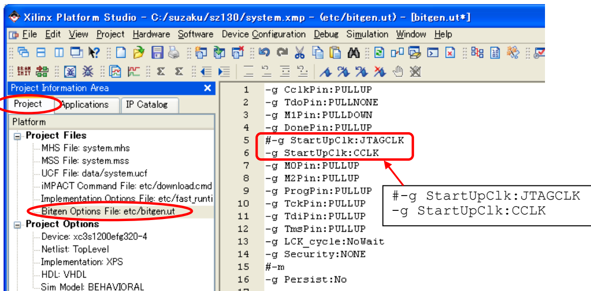
図 10-30 bitgen.ut の変更
