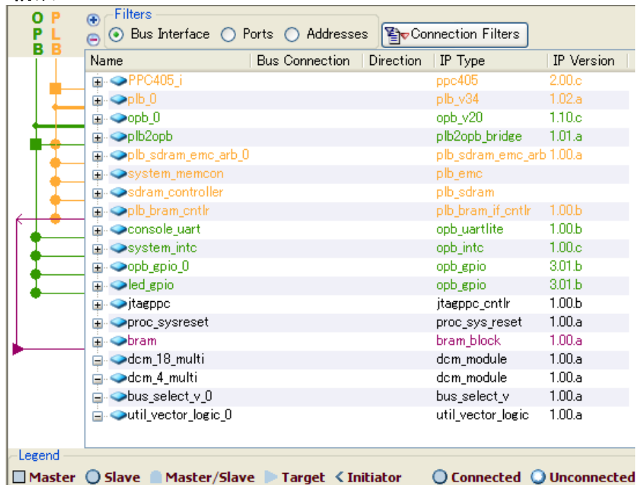
図 10-36 SZ310 のデフォルト(EDK)
