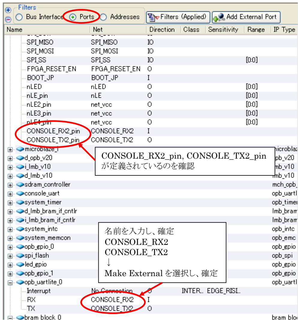
図 10-81 信号の定義
