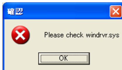
図 6-33 エラー表示
