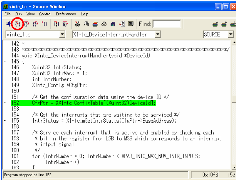
図 11-62 XIntc_DeviceInterruptHandler( )で Break
