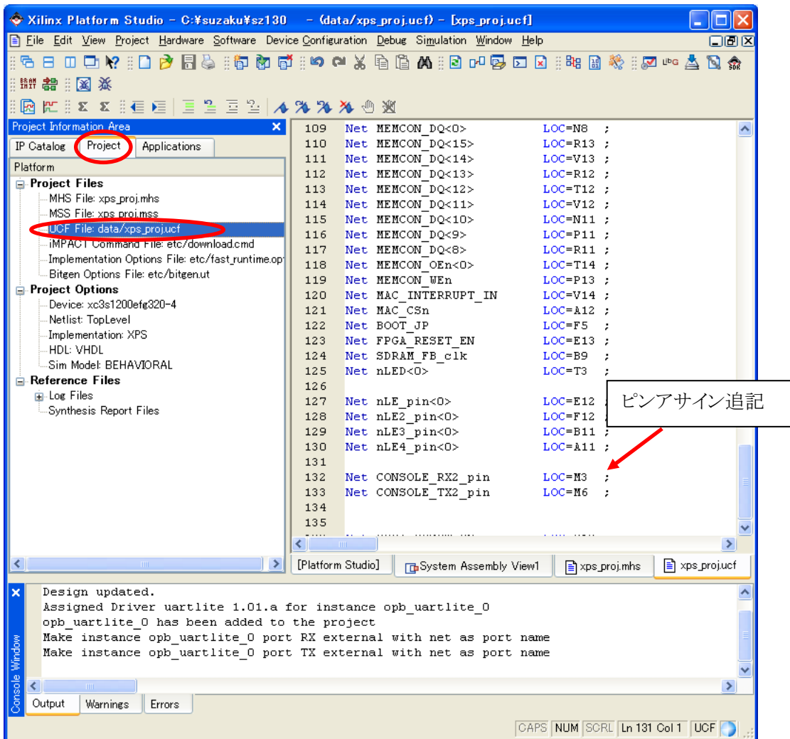
図 10-82 UART(xps_prj.ucf)
