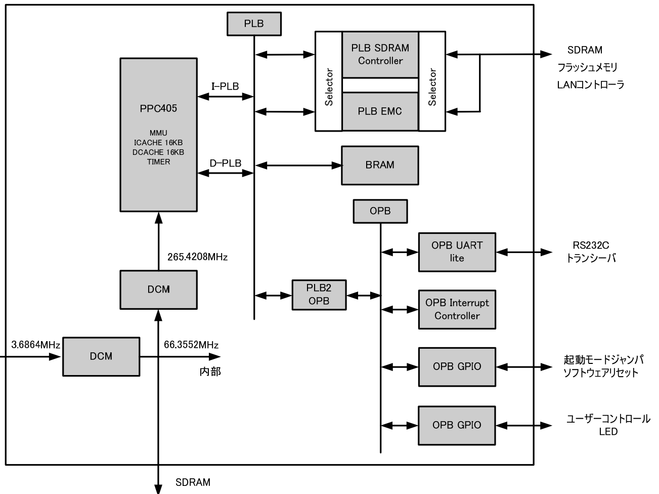
図 10-37 SZ310 デフォルトのブロック図
