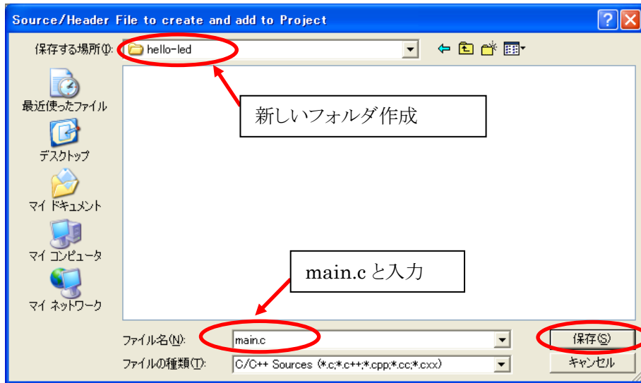
図 10-59 main.c 作成
