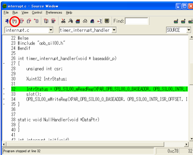
図 11-63 timer_interrupt_handler()で Break
