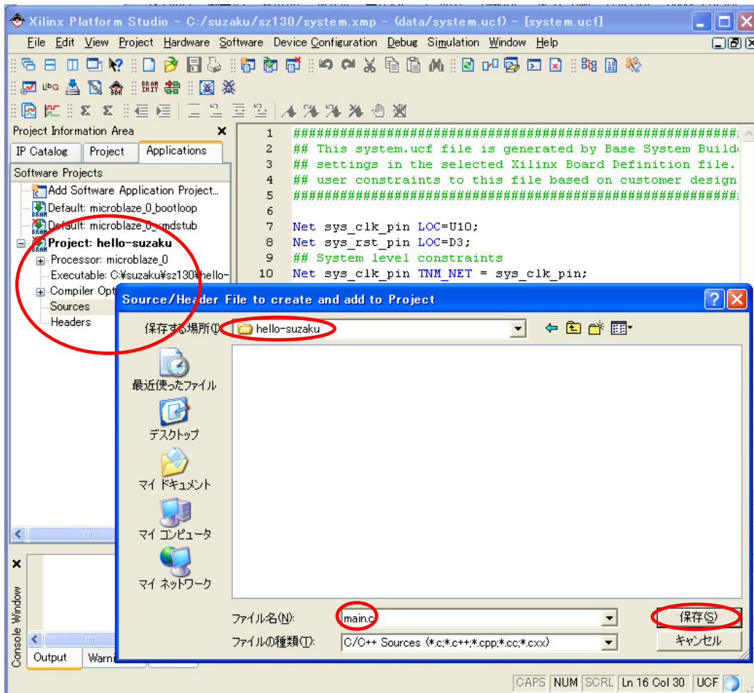
図 10-24 main.c 作成
