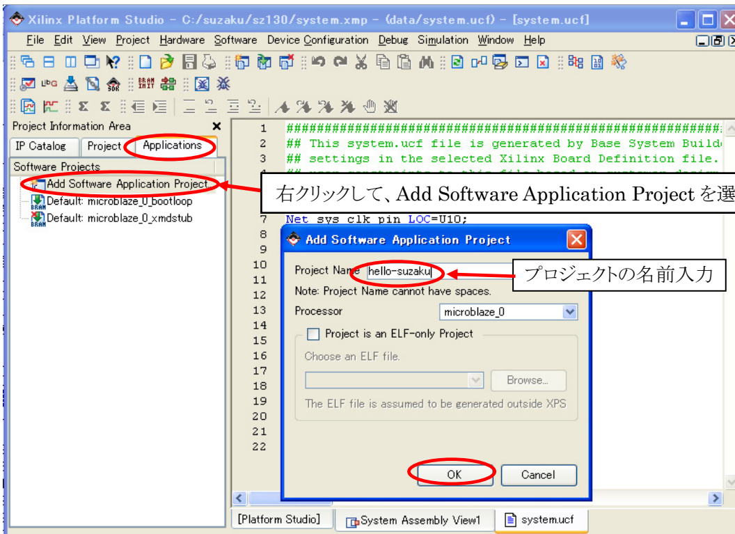
図 10-23 hello-suzaku 作成
