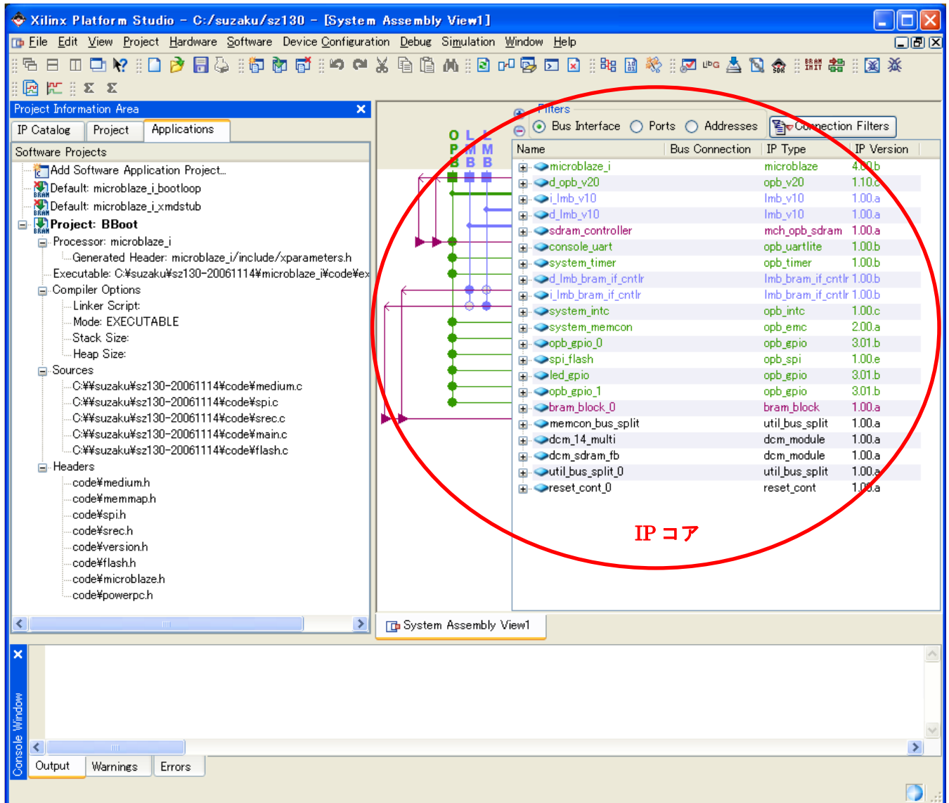
図 10-31 XPS 起動
