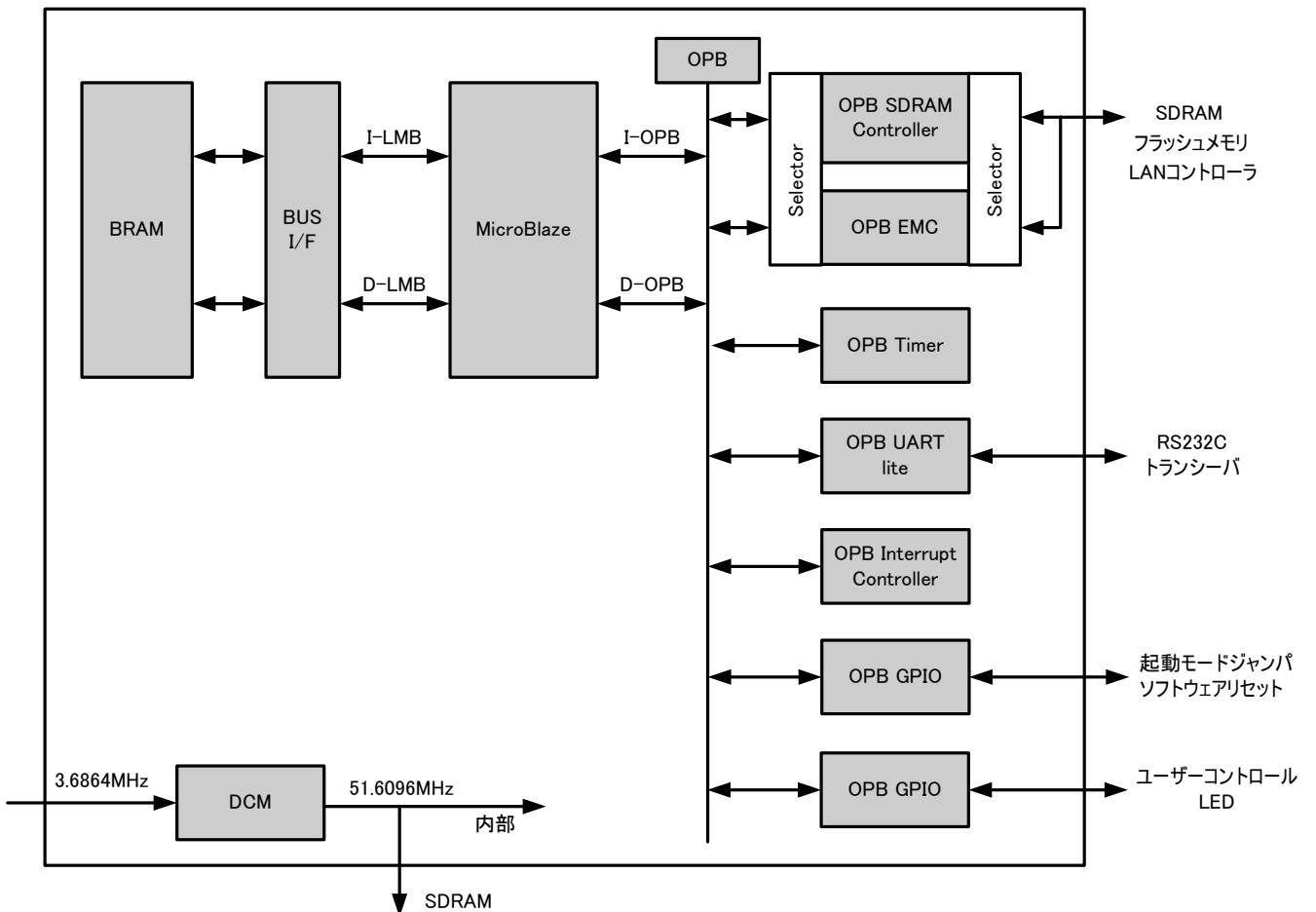
図 10-33 SZ010、SZ030 デフォルトのブロック図
