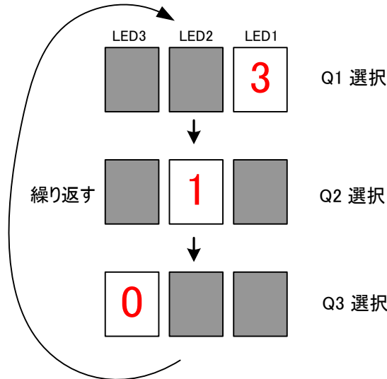
図 9-24 7セグメントLEDダイナミック点灯
