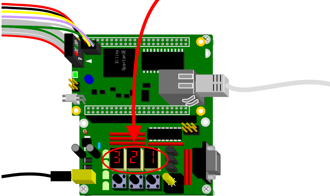
図 12-16 自作のコアをコントロール
