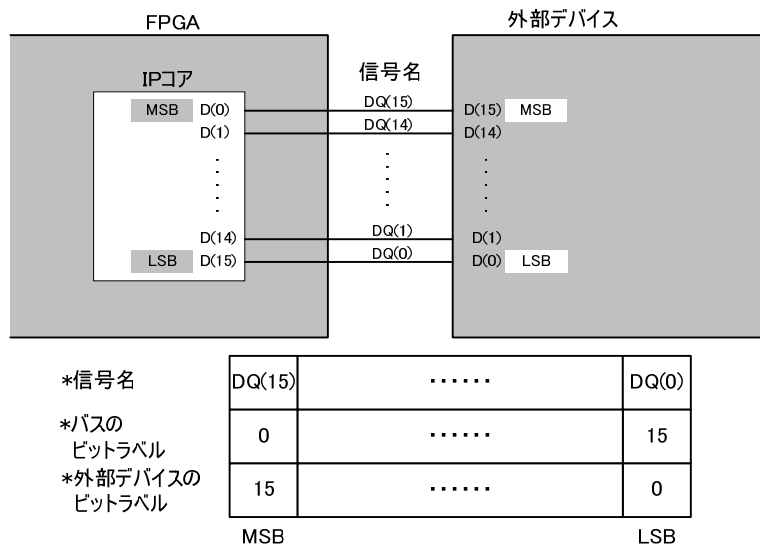
図 2-2 CoreConnect のビットラベルと信号
