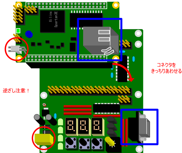
図 4-2 組み立て工程 1
