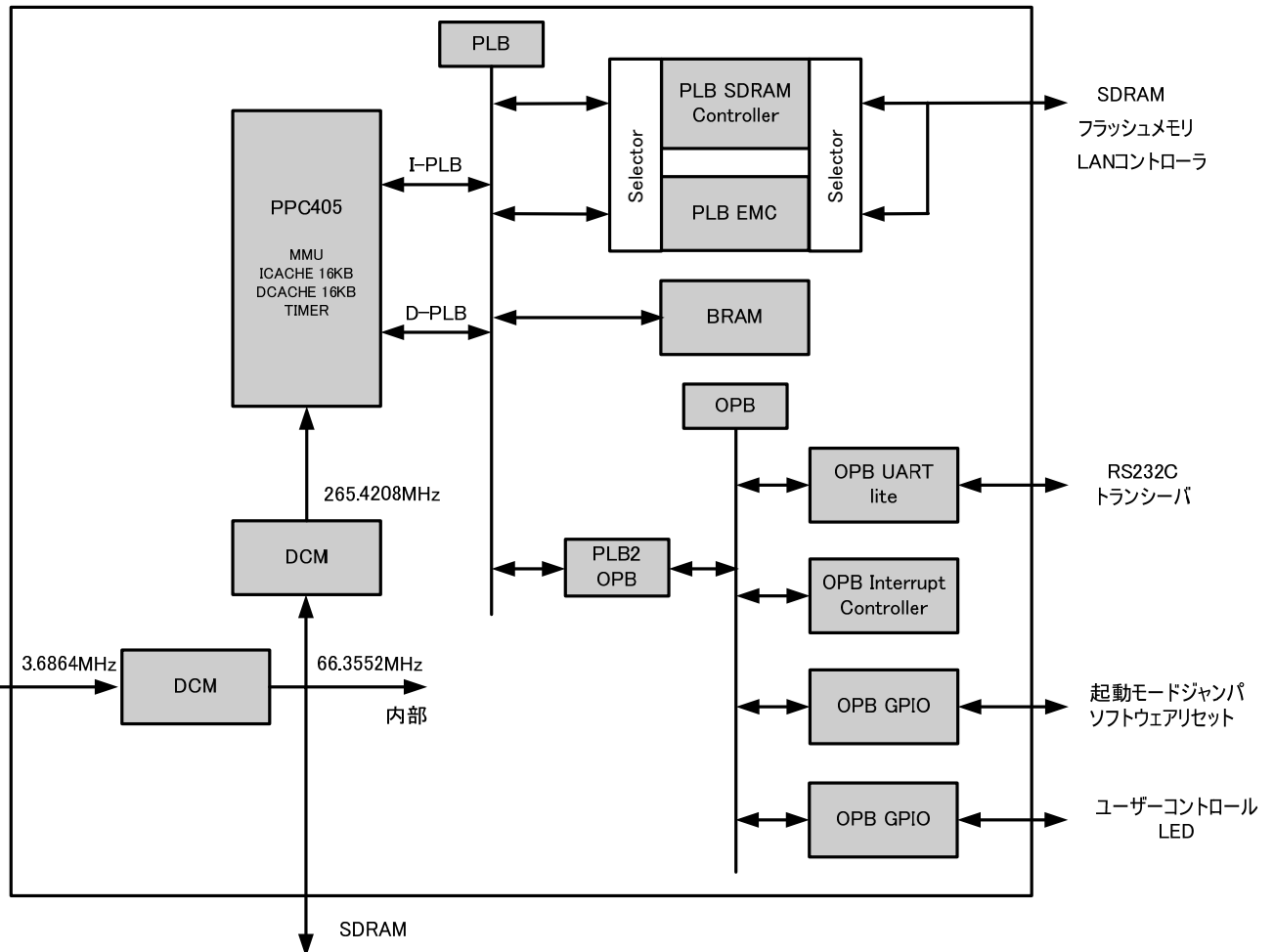
図 10-35 SZ310 デフォルトのブロック図
