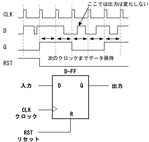
図 8-7 D-FF の動作
