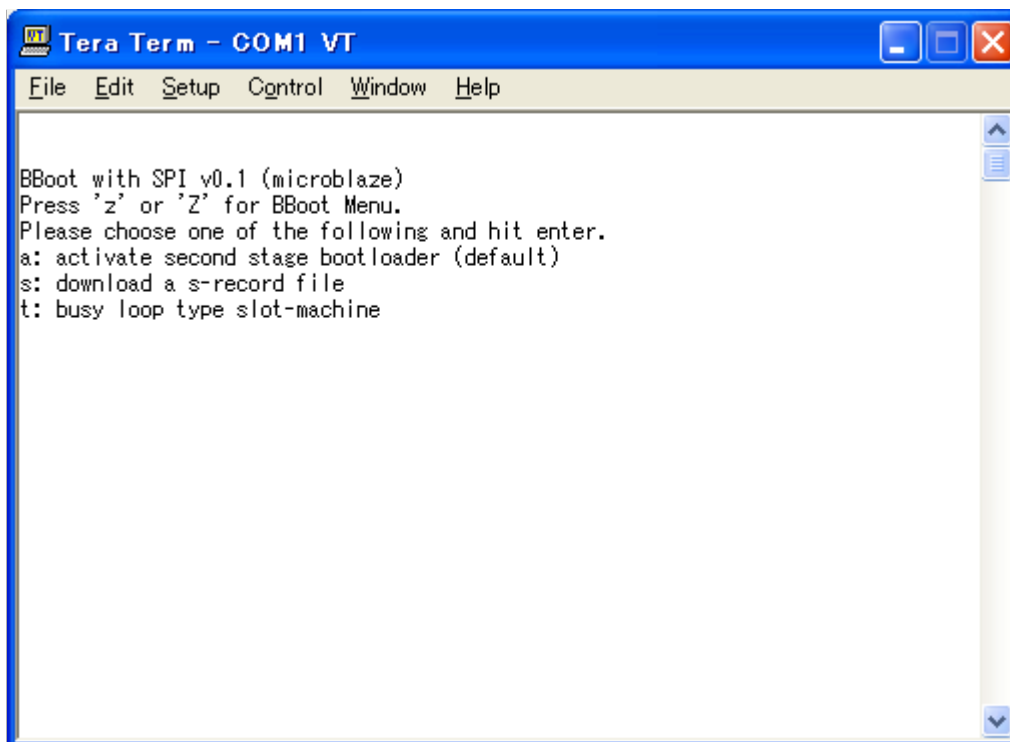
図 5-9 スロットマシンの起動(SZ130 の場合)
