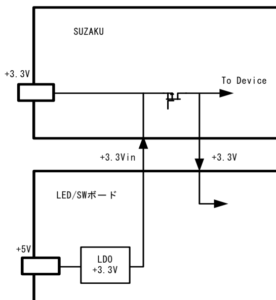
図 5-4 電源系統
