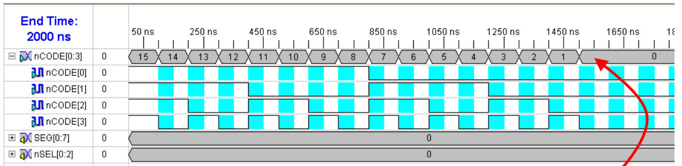
図 9-19 波形生成
