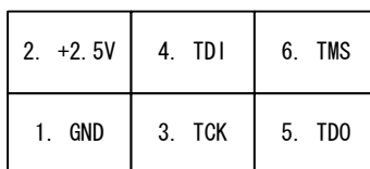
図 13-1 JTAG ピンアサイン
