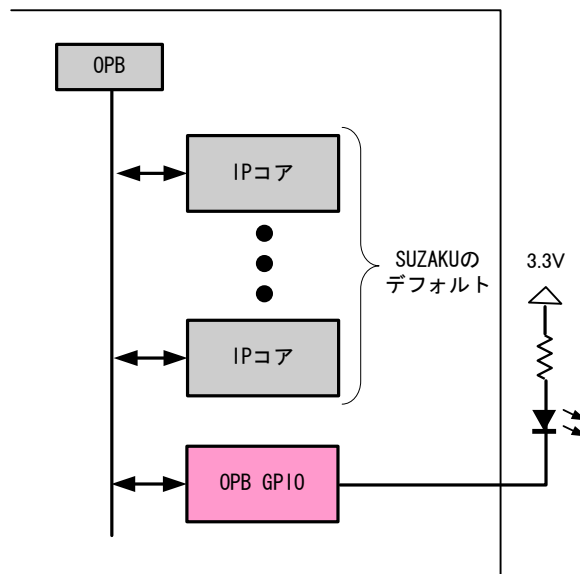
図 10-10 GPIO を追加して LED を点灯
