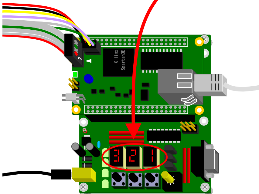
図 5-7 CGI を動かしてみる
