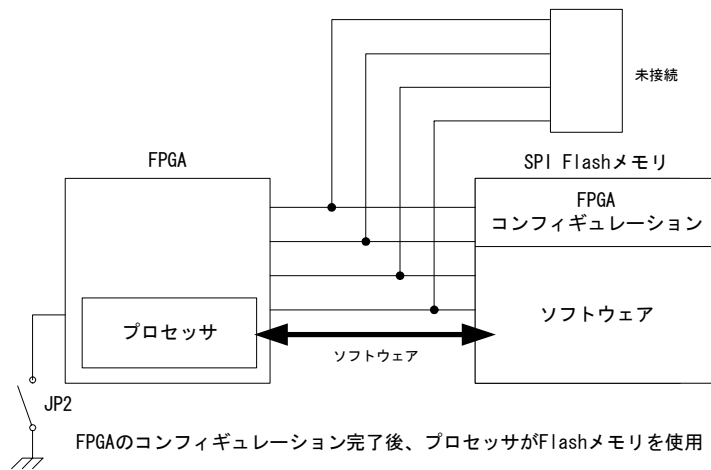
図 6-24 SPI モードの書き込み
