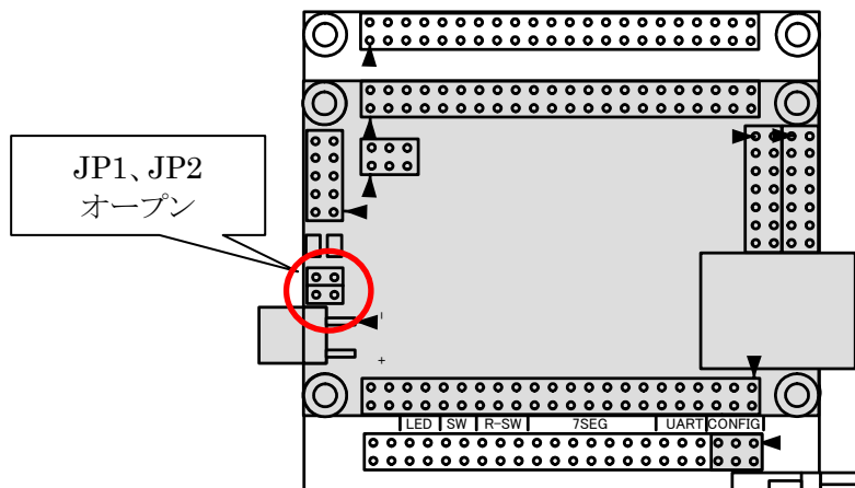
図 5-3 オートブートモード ジャンパの設定
