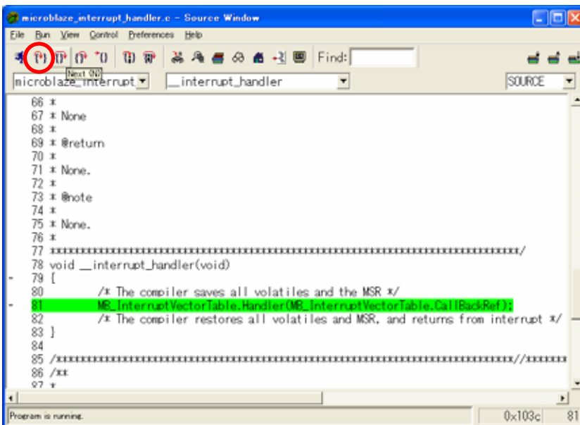
図 11-59 __interrupt_handler() で Break
