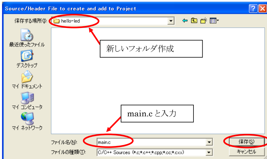
図 10-30 main.c 作成
