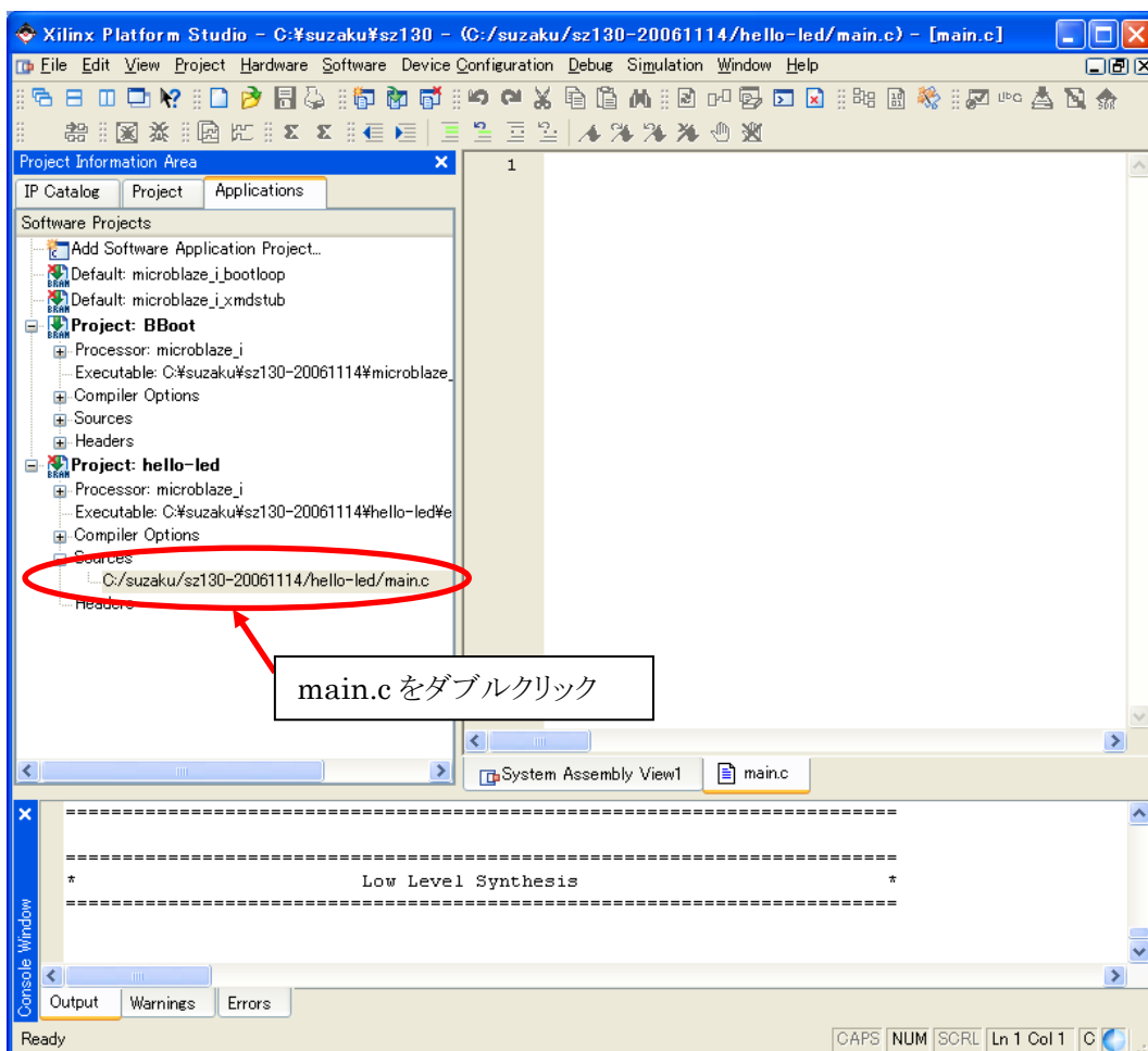
図 10-31 main.c を開く
