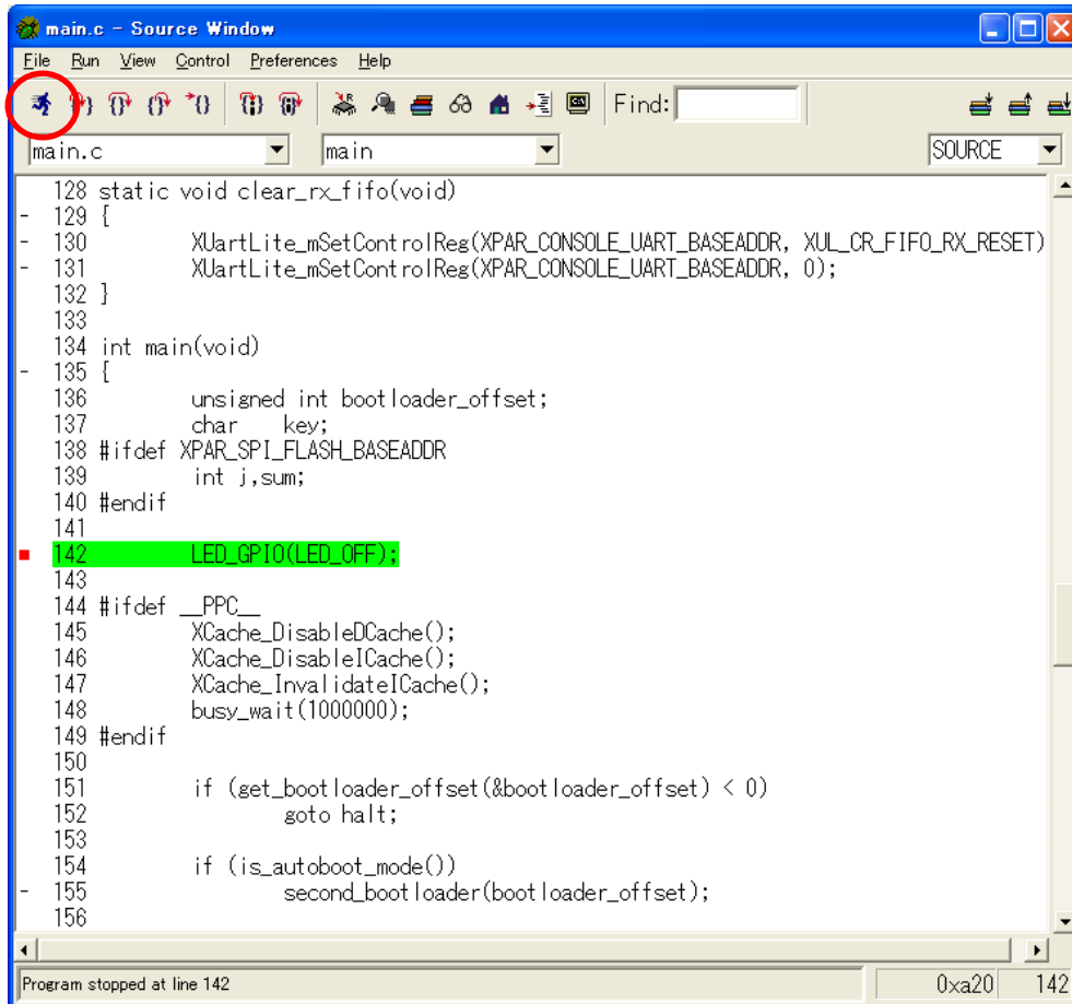
図 11-57 main で Break
