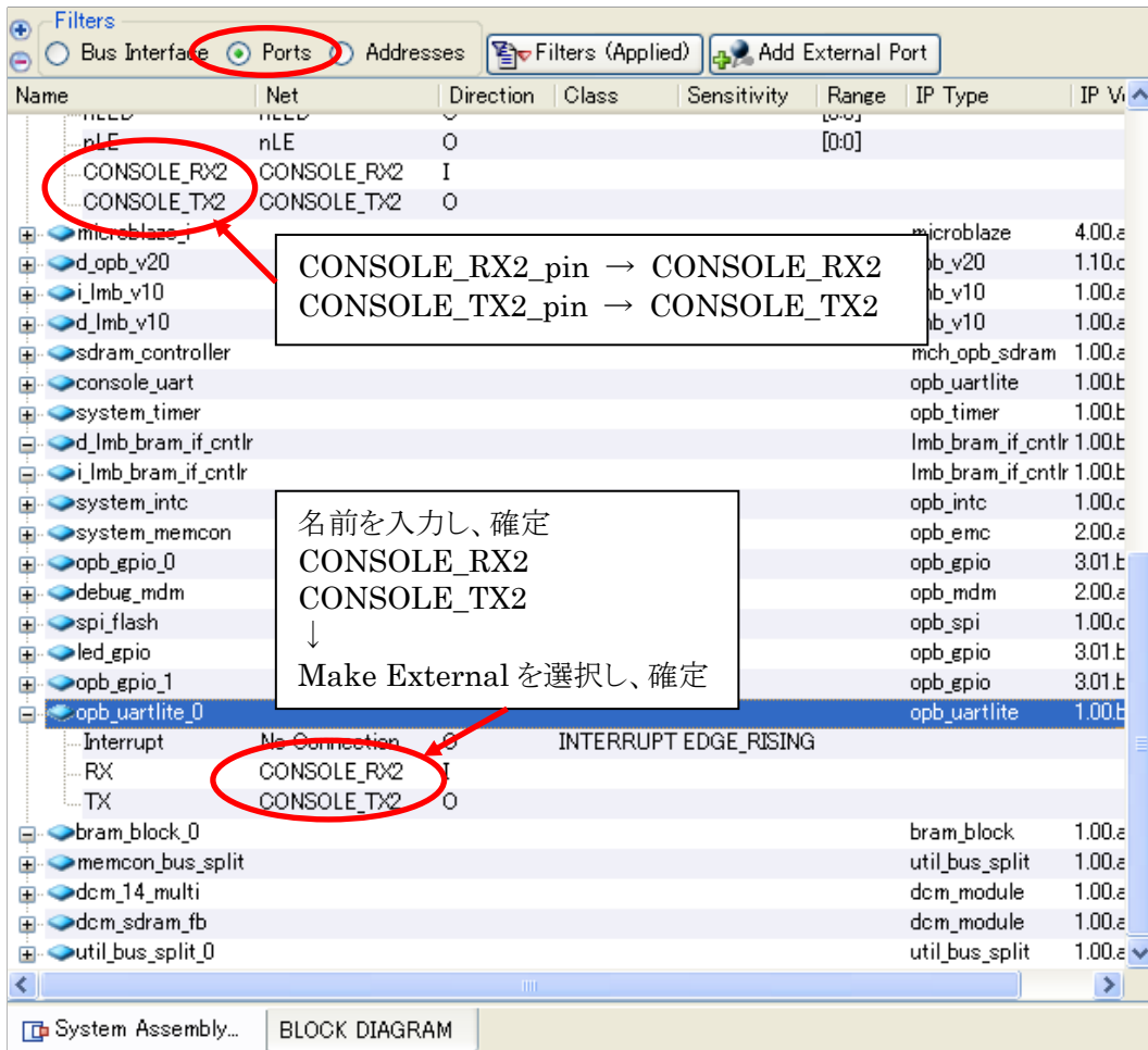
図 10-50 信号の定義
