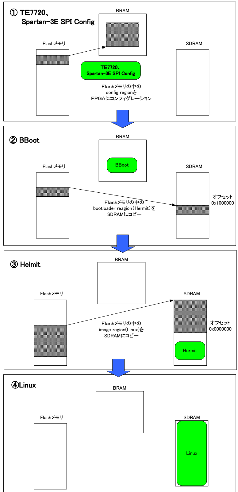
図 11-41 2 段階ブート
