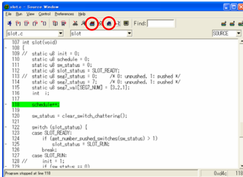
図 11-62 slot() で Break
