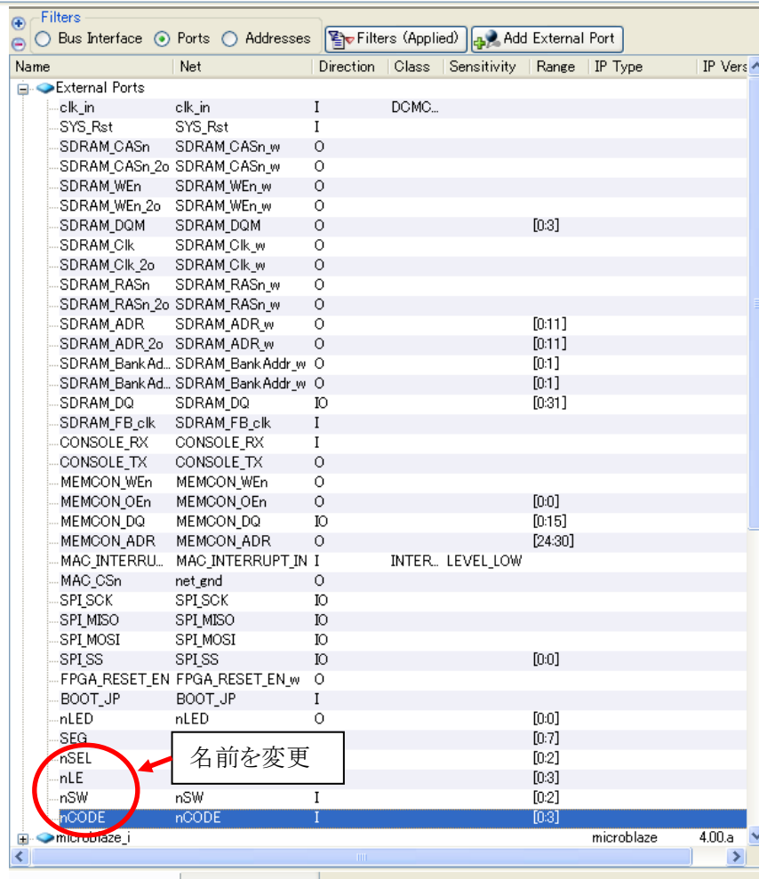
図 11-32 残り出力信号定義
