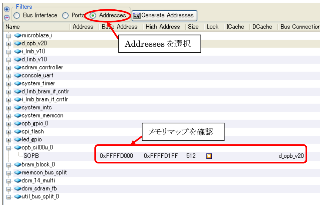
図 11-28 メモリマップ確認
