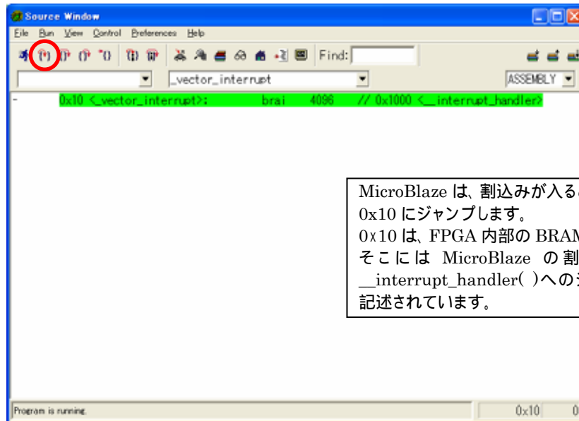
図 11-58 0x10 で Break
