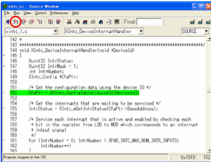
図 11-60 XIntc_DeviceInterruptHandler( )で Break
