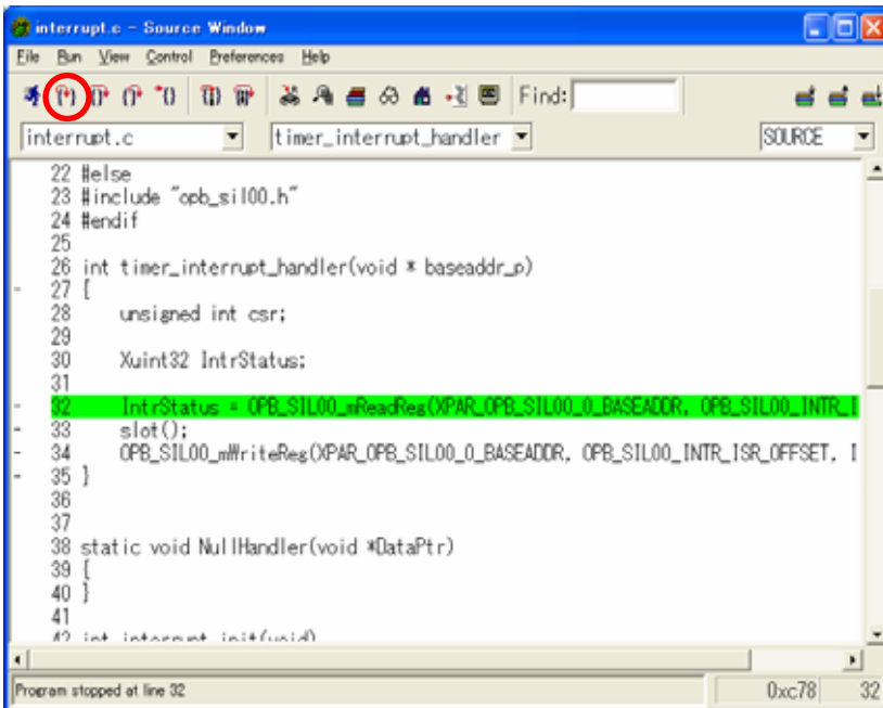
図 11-61 timer_interrupt_handler()で Break
