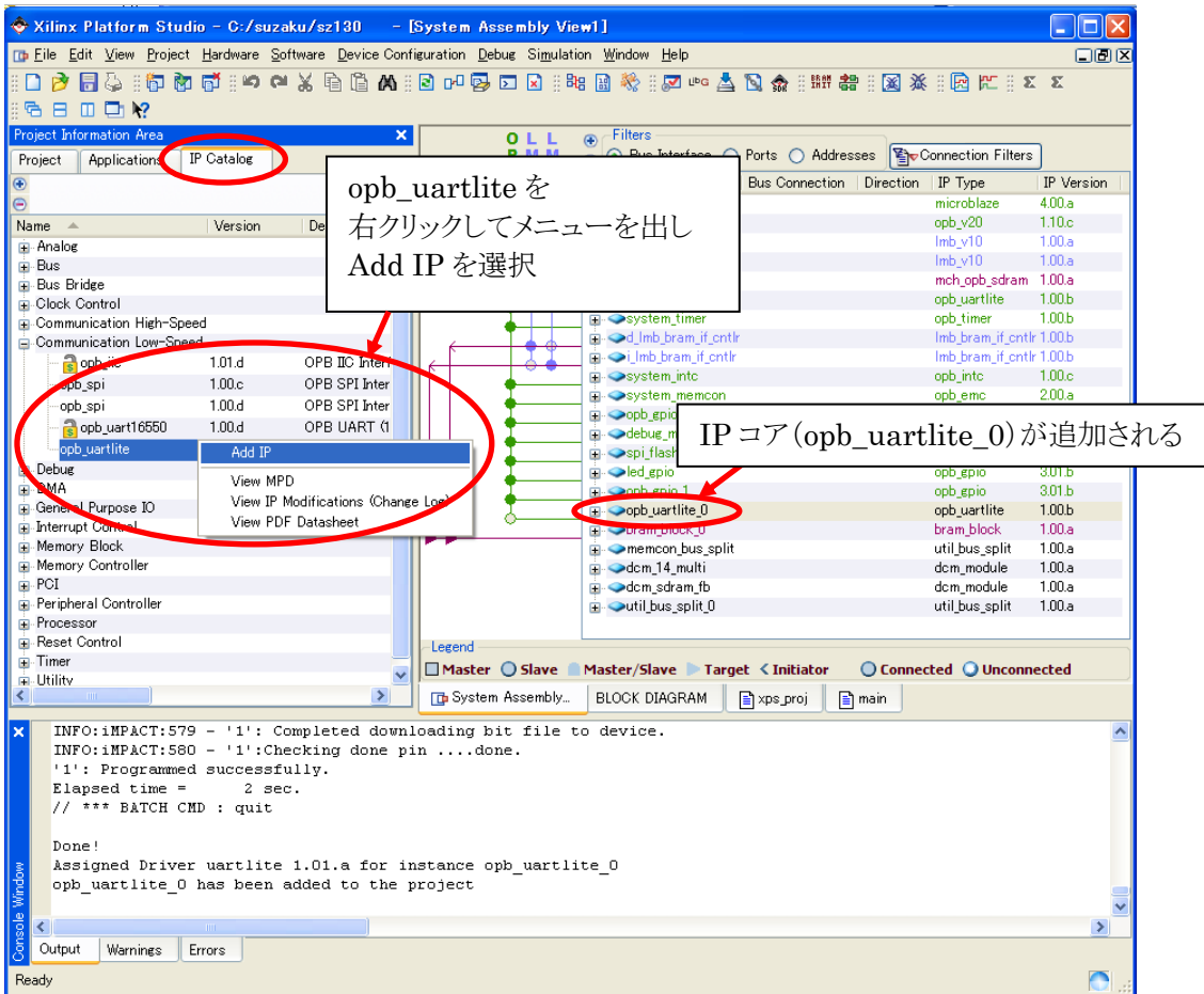
図 10-43 opb_uartlite の追加
