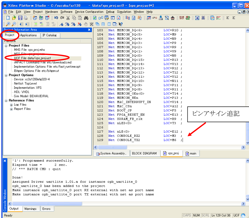
図 10-51 UART(xps_prj.ucf)
