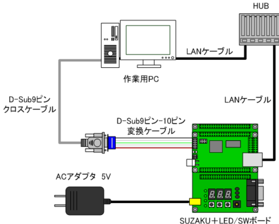
図 2.1. SIL00-U01 接続例
