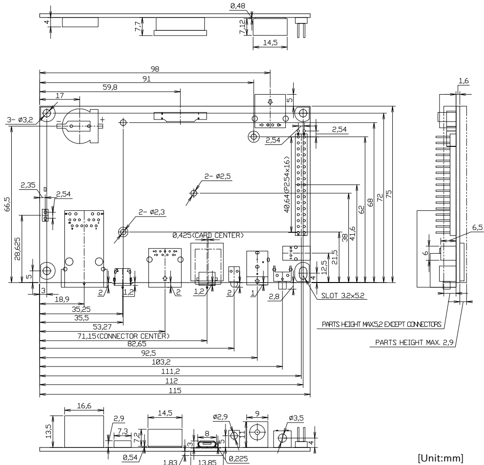
図 3.36 基板形状図
