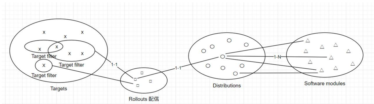
図 5.12 hawkBit が扱うソフトウェアのデータ構造
