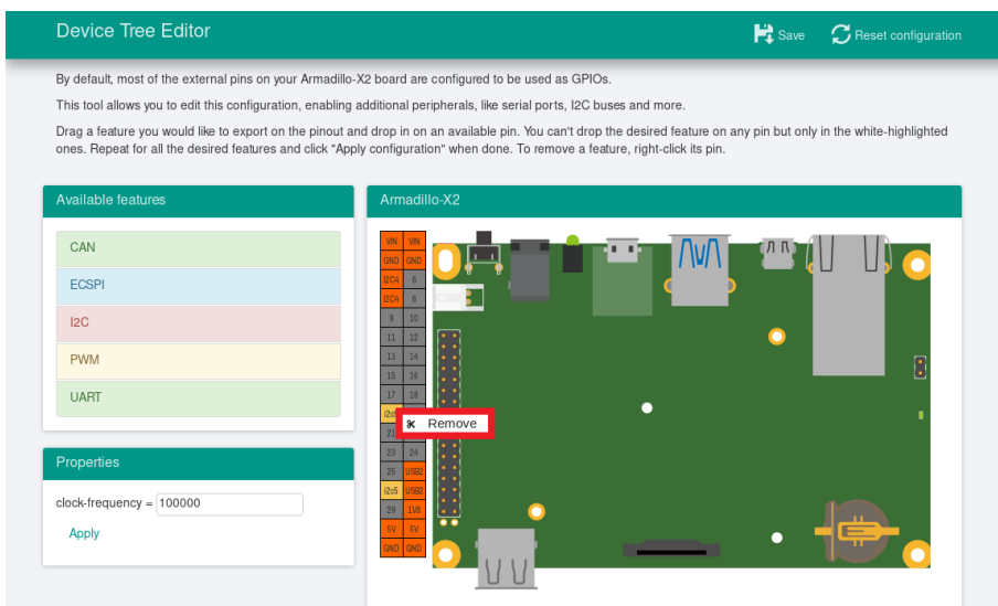
図 3.47 I2C5(SCL/SDA) の削除
