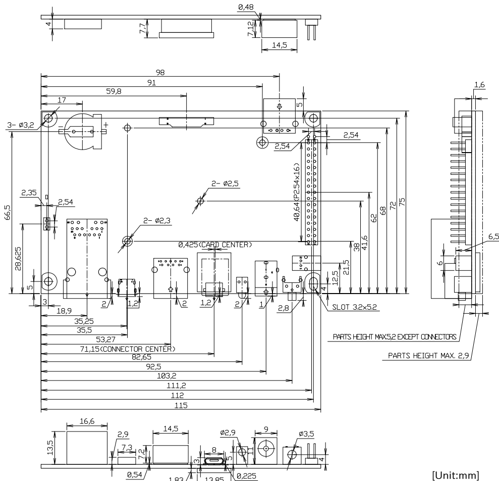
図 3.59 基板形状図
