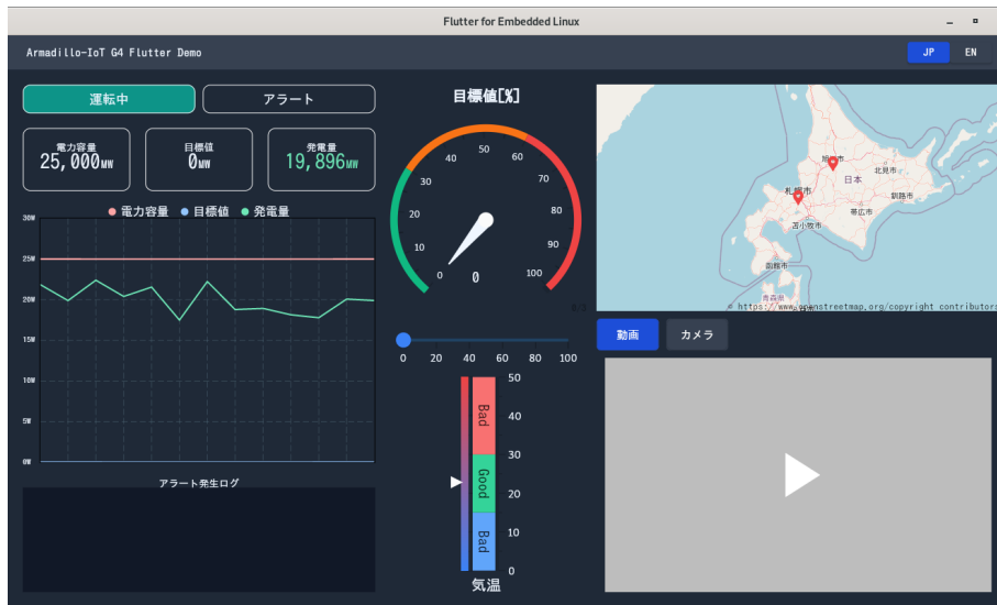
図 3.174 起動したサンプルアプリケーション
