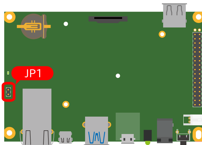
図 3.7 ジャンパピンの位置
