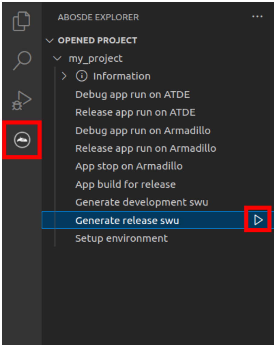
図 3.194 SWU イメージを作成する
