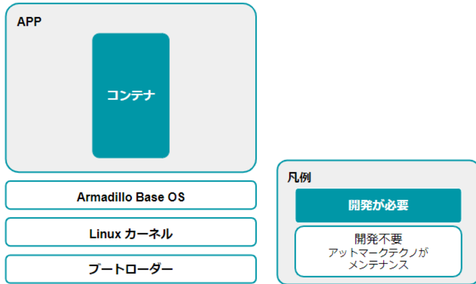
図 3.119 開発者が開発するもの、開発しなくていいもの
