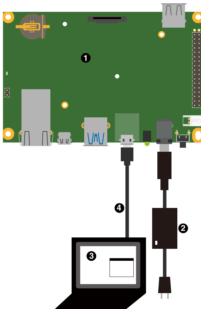
図 3.40 シリアルコンソールを使用する配線例
