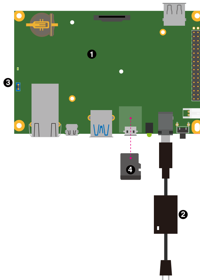
図 3.6 Armadillo-X2 を初期化する接続
