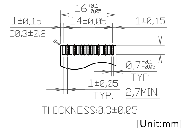
図 3.91 CON10 接続可能なフレキシブルフラットケーブルの形状
