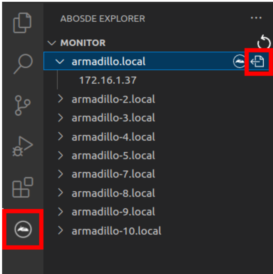
図 3.221 ABOSDE を使用して ssh 接続に使用する IP アドレスを設定する
