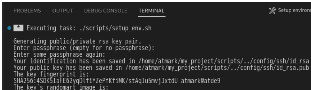
図 3.201 VSCode のターミナル
