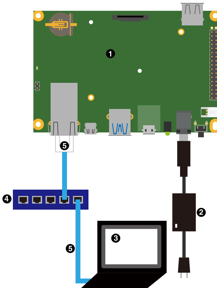
図 3.10 ABOS にアクセスするための接続
