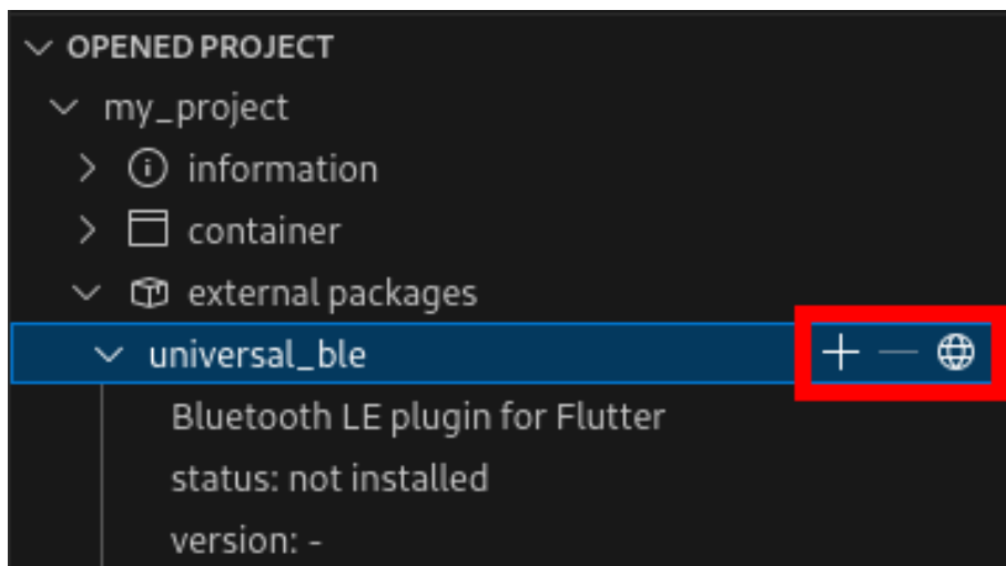
図 3.179 BLE パッケージをインストールする
