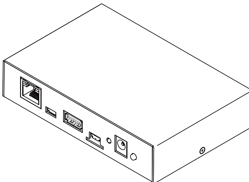
図 6.203 Armadillo-X2 オプションケース(金属製)
