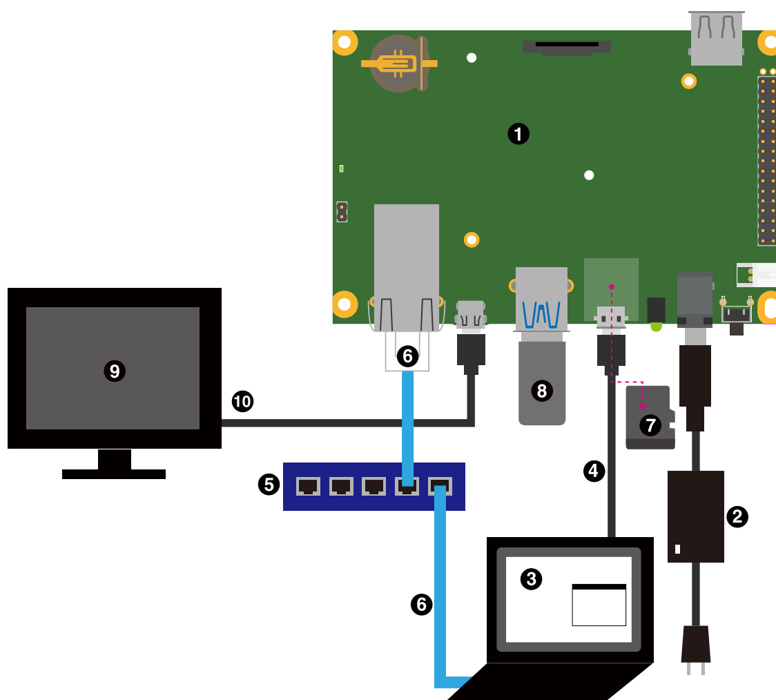
図 3.49 Armadillo-X2 の接続例
