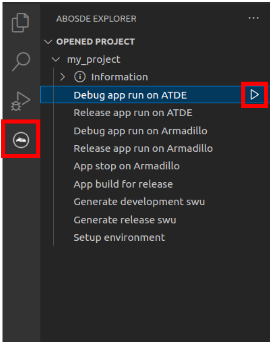
図 3.173 ATDE 上で Debug モードでビルドしたアプリケーションを実行する
