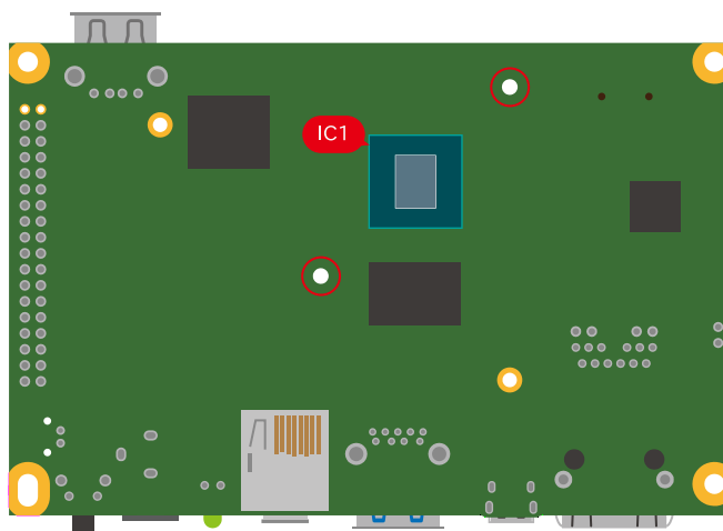
図 3.48 Armadillo-X2 の IC1 とヒートシンク固定穴の位置
