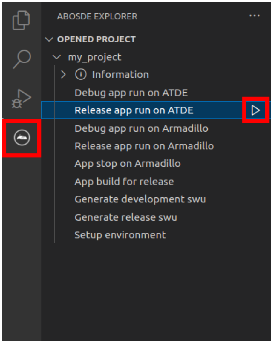
図 3.175 ATDE 上で Release モードでビルドしたアプリケーションを実行する
