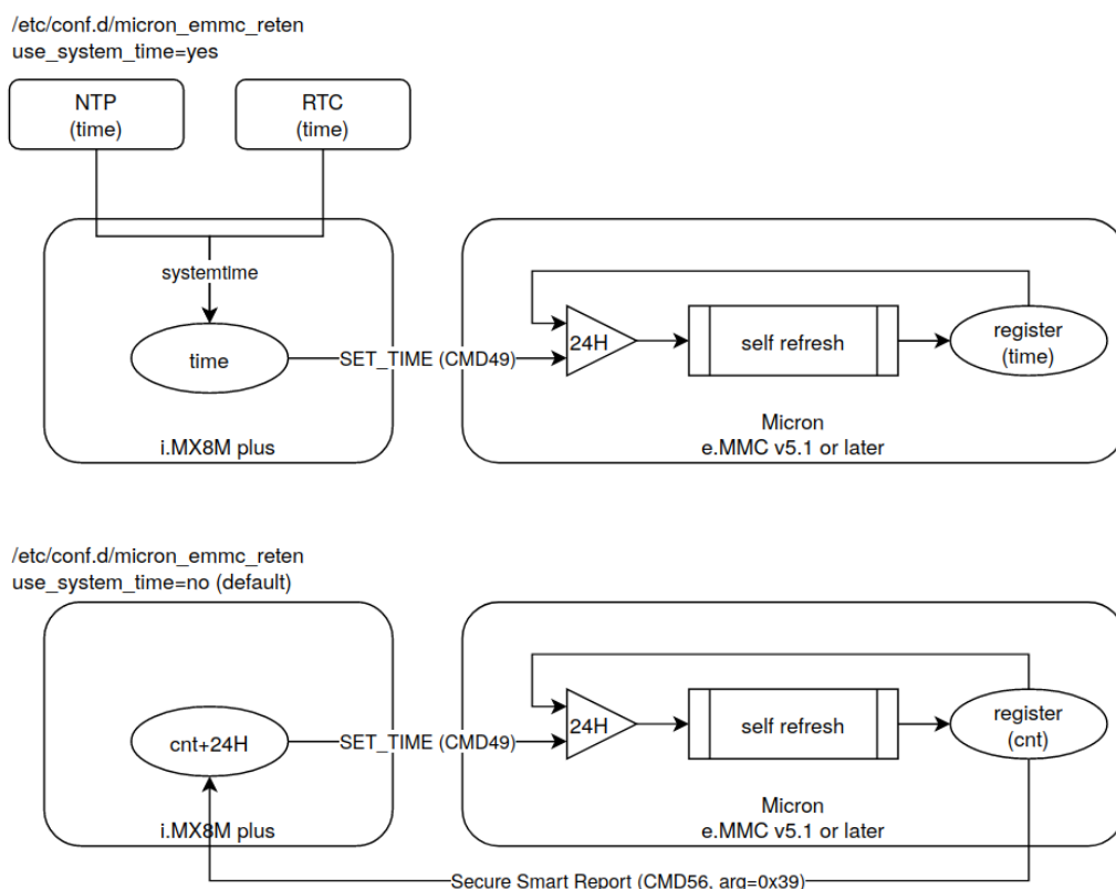
図 6.197 データリテンション開始トリガーの方式
