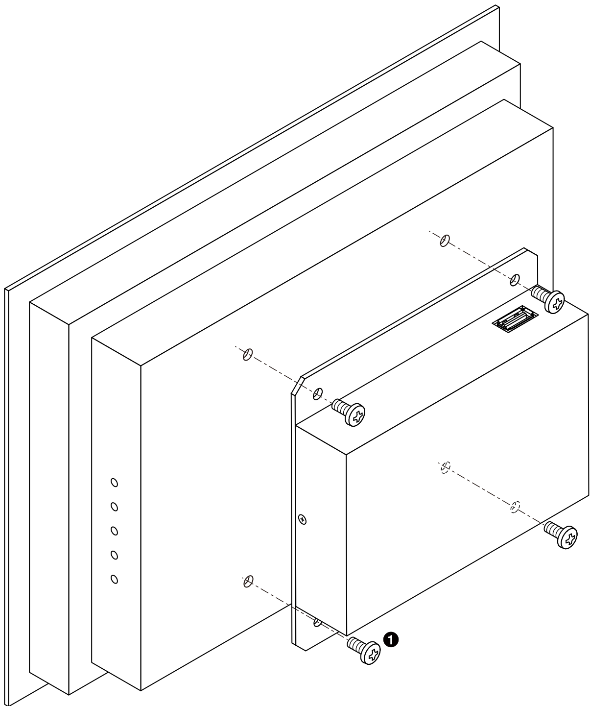
図 6.207 モニターに VESA 規格固定用プレートを取り付け
