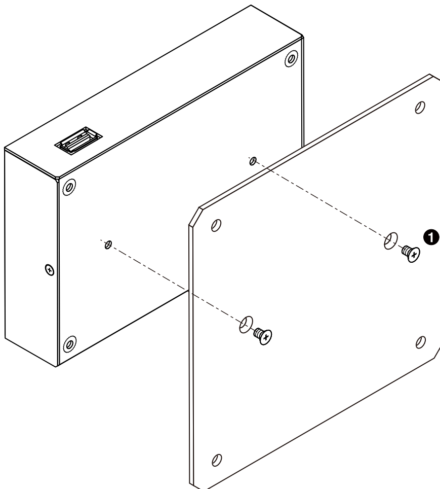
図 6.206 ケースに VESA 規格固定用プレートを取り付け
