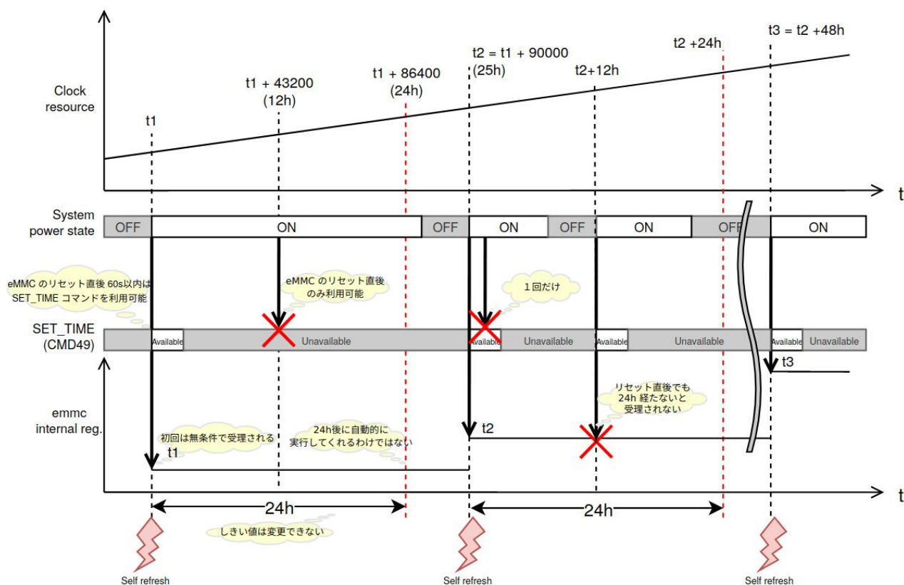
図 6.192 データリテンションの開始トリガーの動作例
