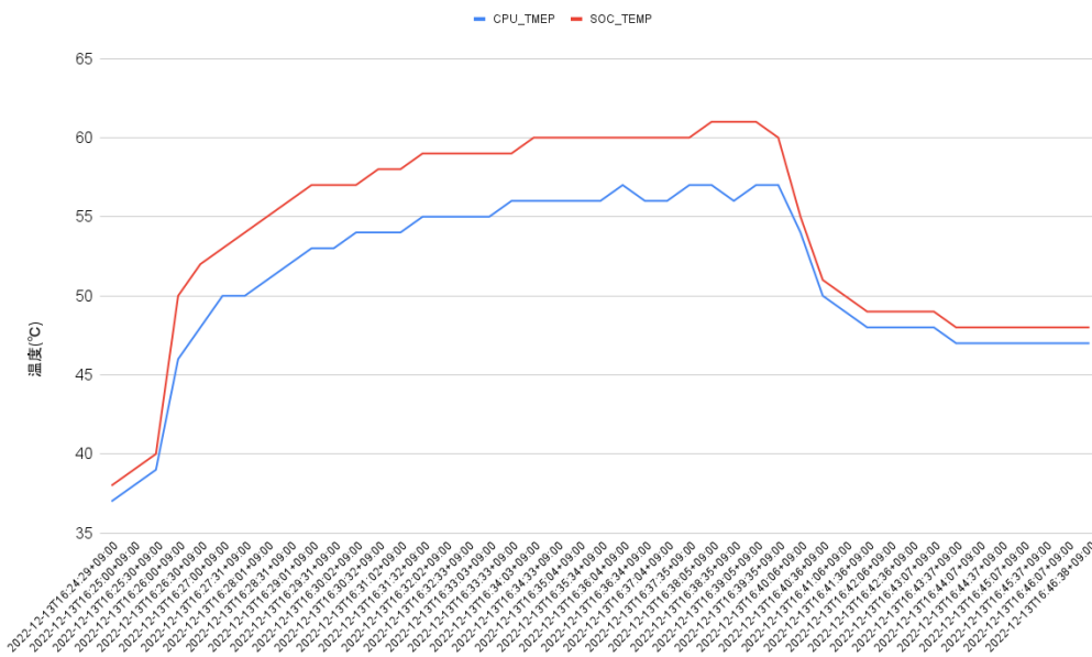
図 6.184 Armadillo-IoT ゲートウェイ G4 で取得した温度のグラフ
