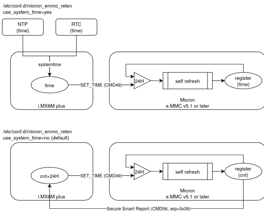
図 6.191 データリテンション開始トリガーの方式
