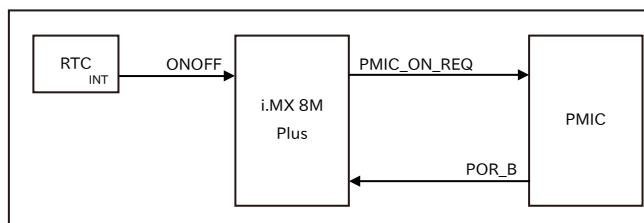
図 6.182 ONOFF 回路の構成
