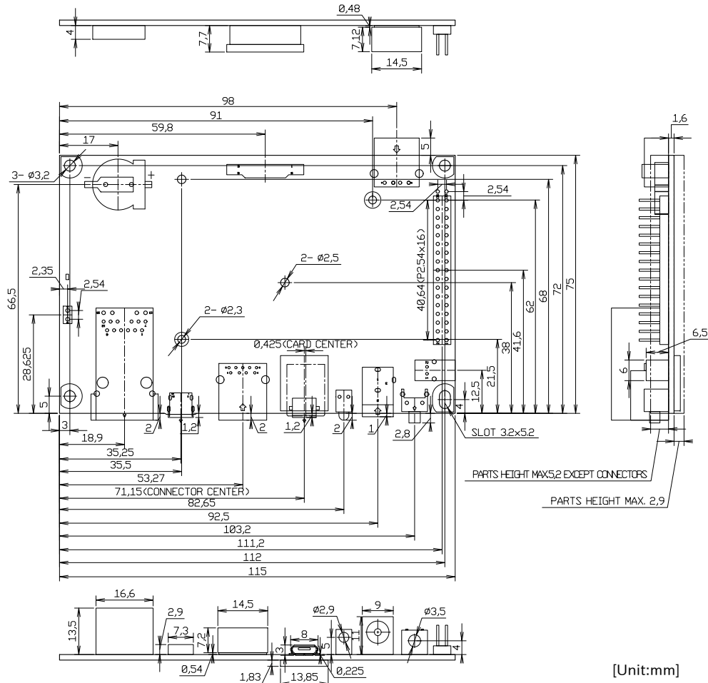
図 6.183 基板形状図
