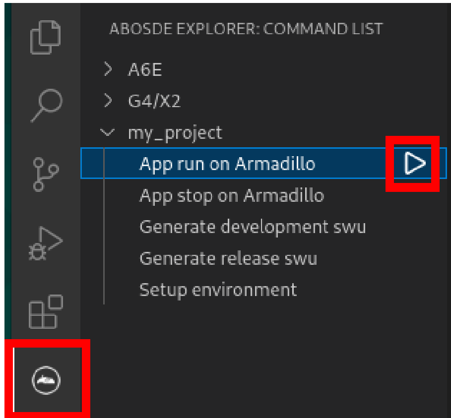
図 3.153 Armadillo 上でアプリケーションを実行する
