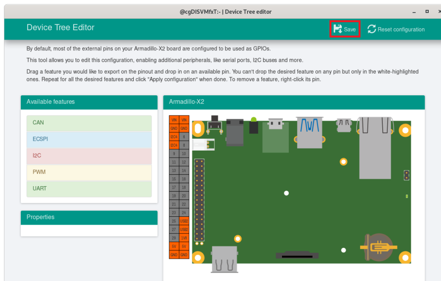
図 3.45 DTS/DTB の生成
