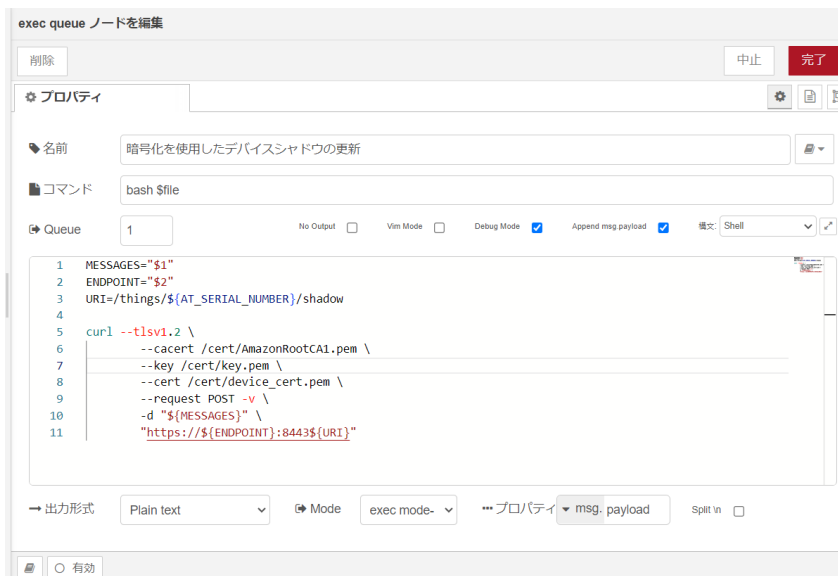
図 4.68 [暗号化を使用したデバイスシャドウの更新] ノードのプロパティ内容
