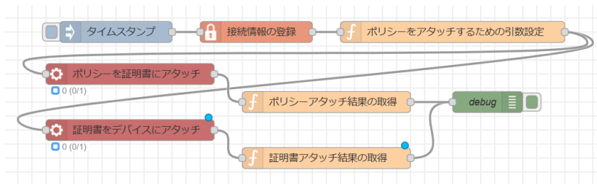
図 4.59 デバイスにポリシーをアタッチするフロー
