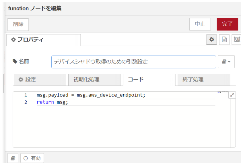
図 4.61 [デバイスシャドウ取得のための引数設定] ノードのプロパティ内容
