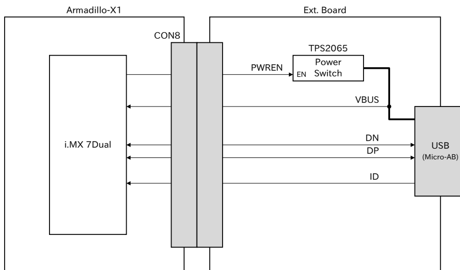
図 21.2 拡張インターフェース USB OTG ブロック図
