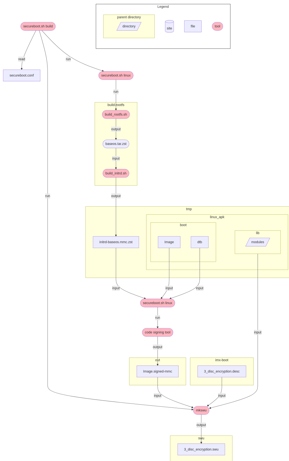
図 3.9 3_disk_encryption.swu を生成するまでの流れ
