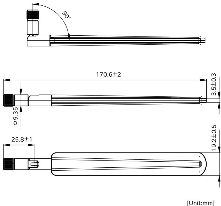
図 6.230 3G/LTE 用外付けアンテナ形状図
