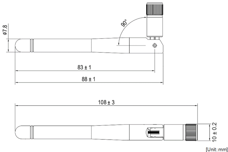
図 6.232 無線 LAN/BT 用外付けアンテナ形状図
