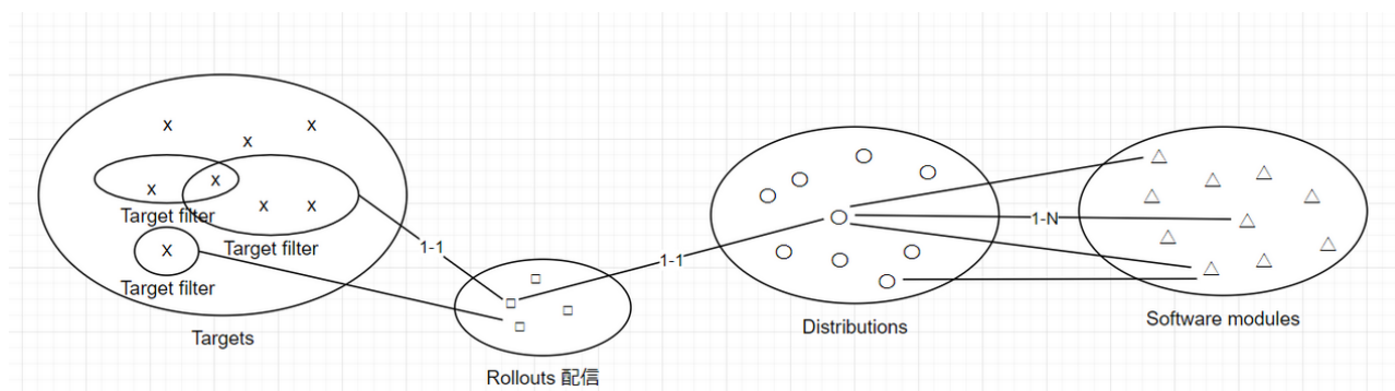
図 5.14 hawkBit が扱うソフトウェアのデータ構造
