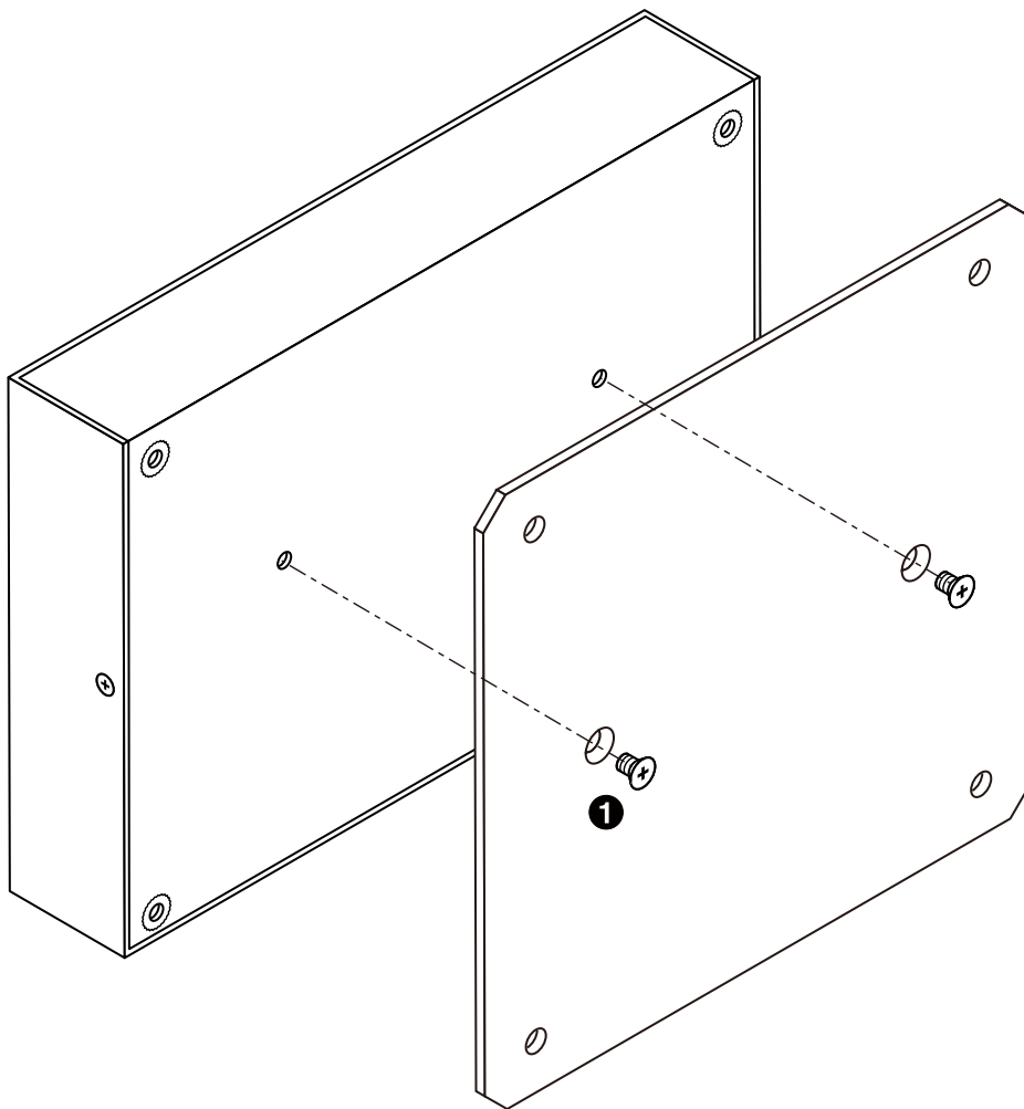
図 6.235 ケースに VESA 規格固定用プレートを取り付け
