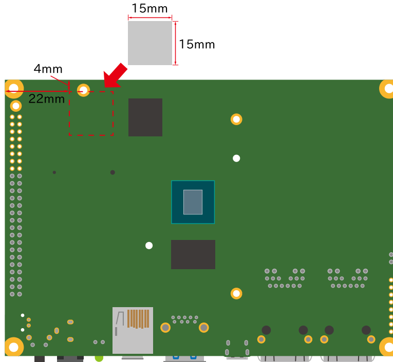
図 4.19 オプションケース(金属製) 放熱シート貼付(WLAN+BT コンポモジュール搭載モデル)
