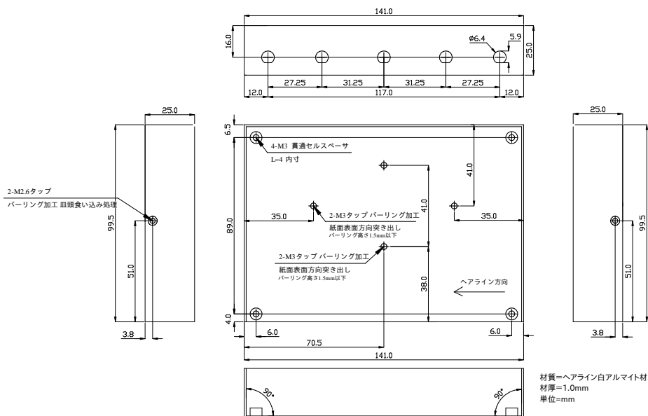
図 6.229 LTE+WLAN モデル ケース(下)形状図
