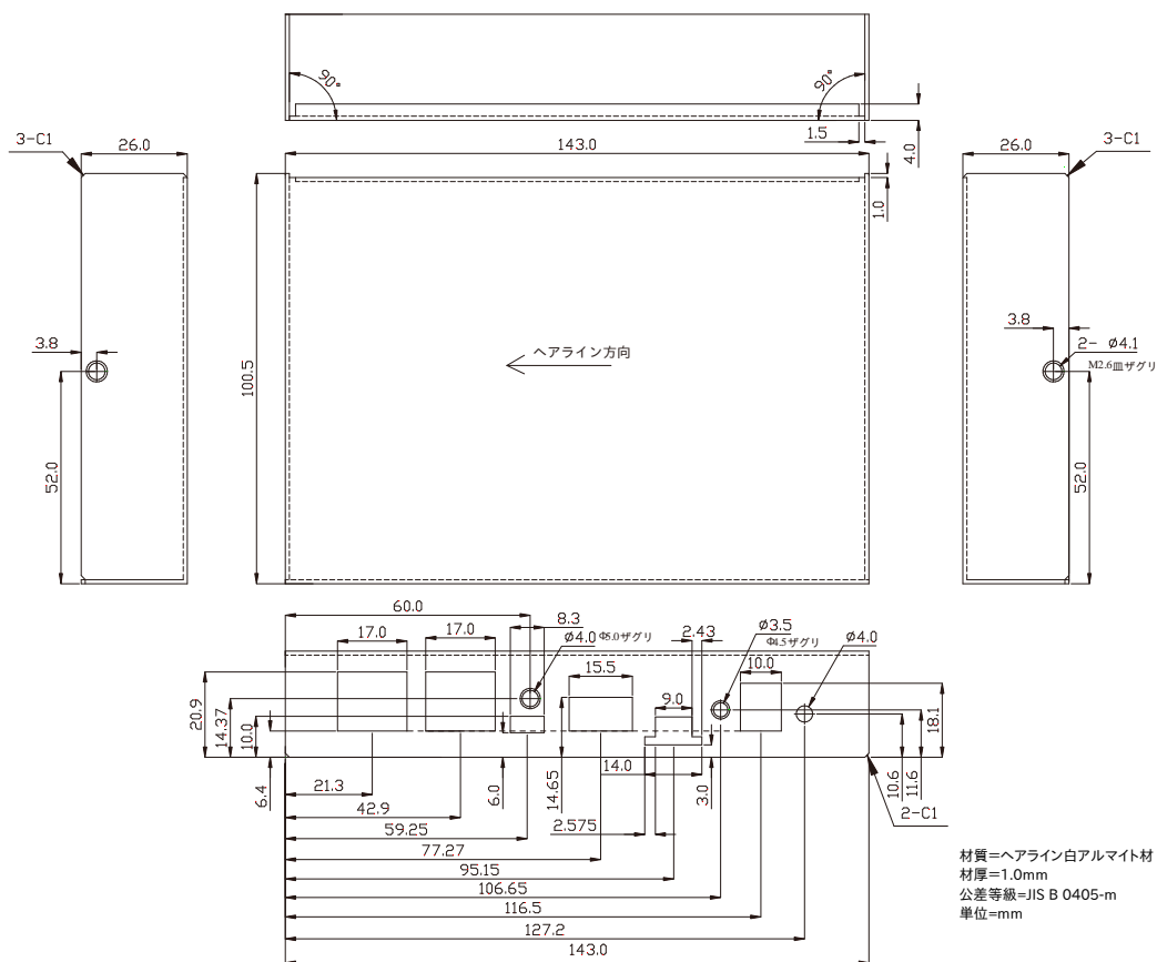
図 6.224 LTE モデル ケース(上)形状図
