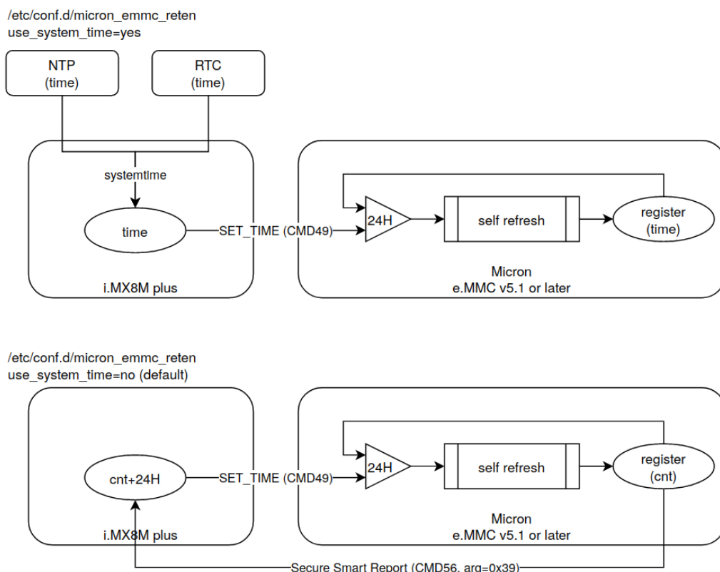
図 6.214 データリテンション開始トリガーの方式
