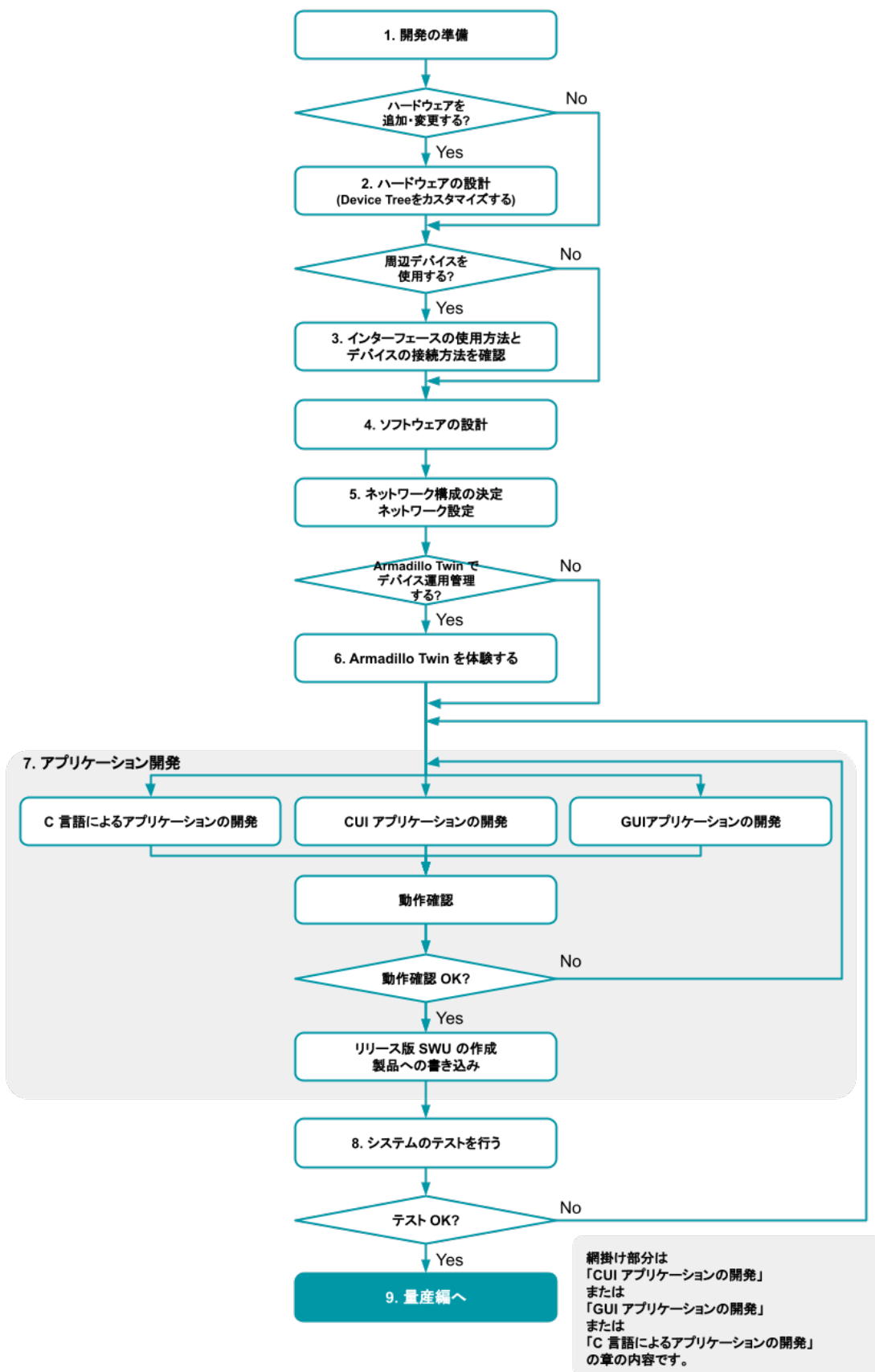
図 3.45 アプリケーション開発の流れ
