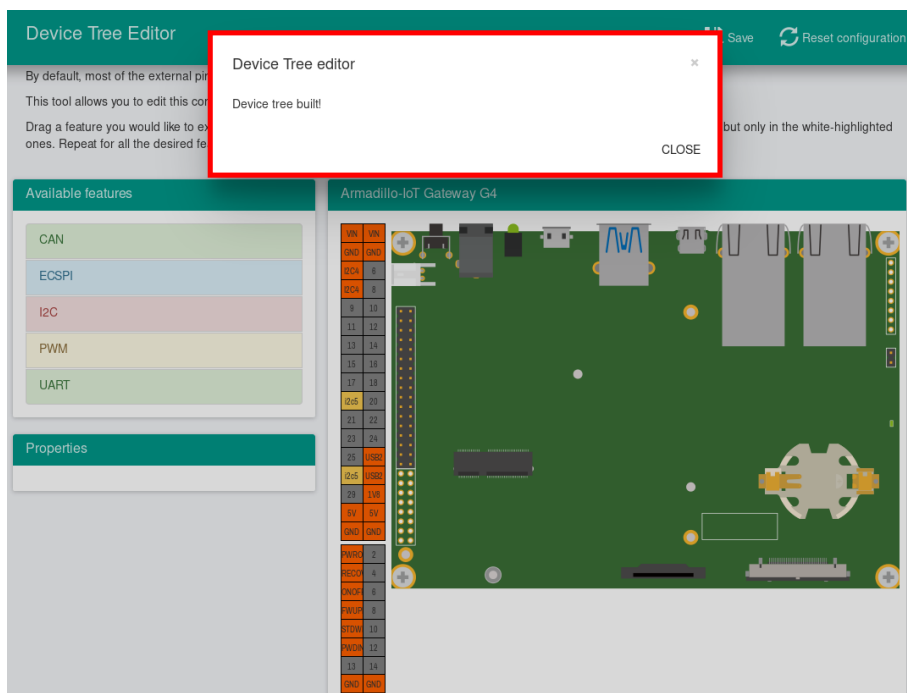
図 3.75 DTS/DTB の生成完了
