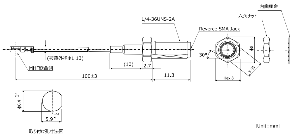
図 6.260 無線 LAN/BT 用アンテナケーブル形状図
