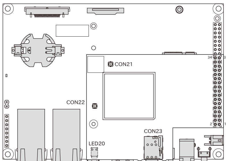
図 3.80 Armadillo-IoT ゲートウェイ G4 インターフェース LTE モデル追加分
