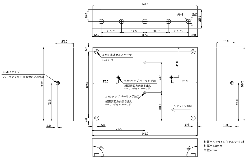
図 6.256 LTE+WLAN モデル ケース(下)形状図
