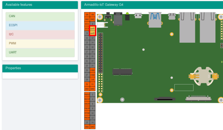
図 3.68 CON11 8/10 ピンへのドロップ
