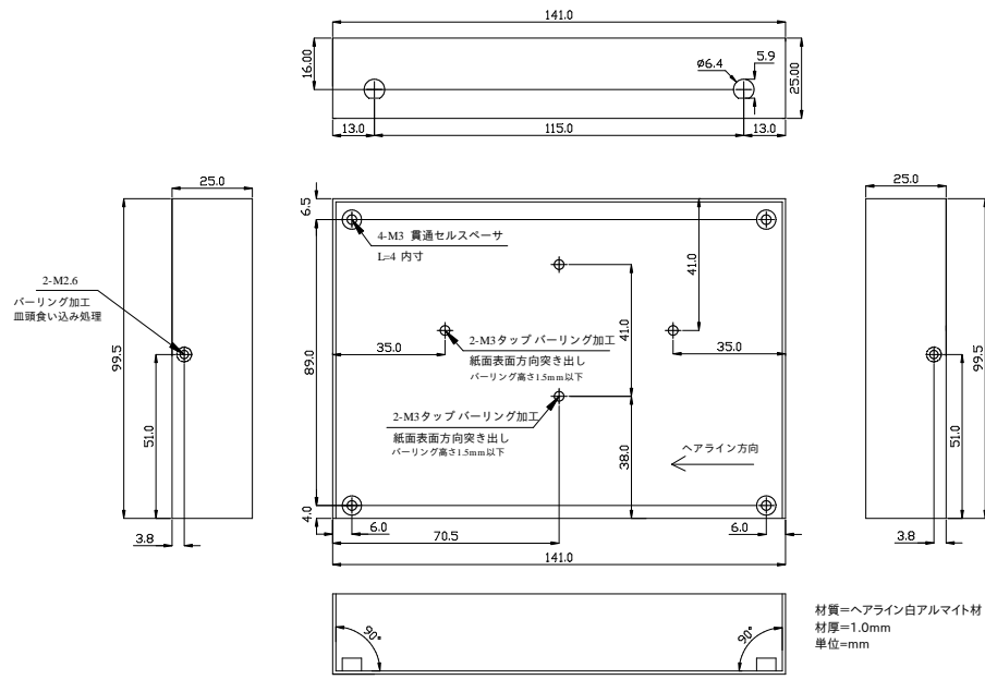
図 6.252 LTE モデル ケース(下)形状図
