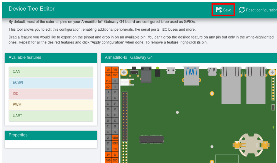
図 3.74 DTS/DTB の生成
