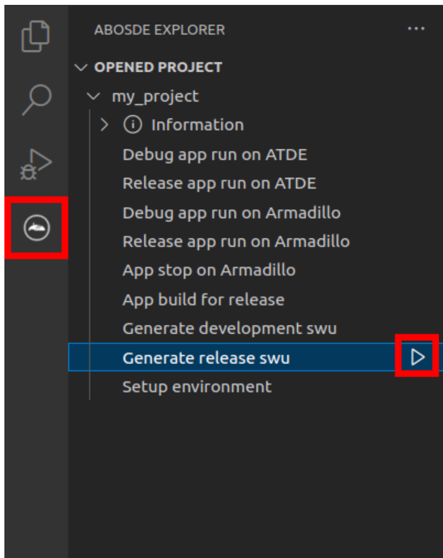
図 3.203 SWU イメージを作成する
