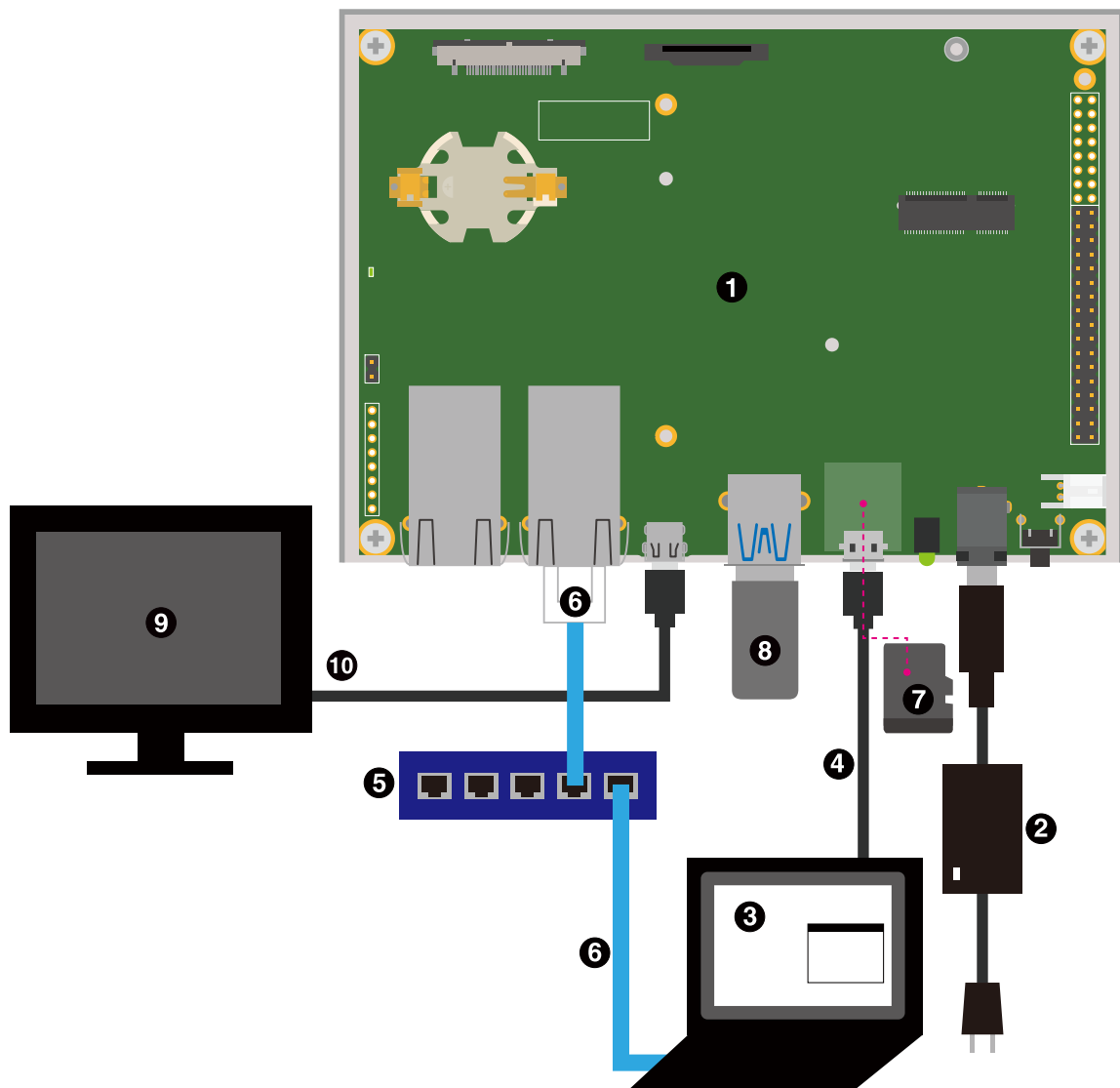
図 3.49 Armadillo-IoT ゲートウェイ G4 の接続例
