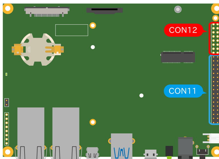
図 3.51 Armadillo-IoT ゲートウェイ G4 の拡張インターフェース
