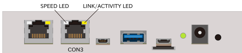
図 3.83 CON3 LAN LED 配置
