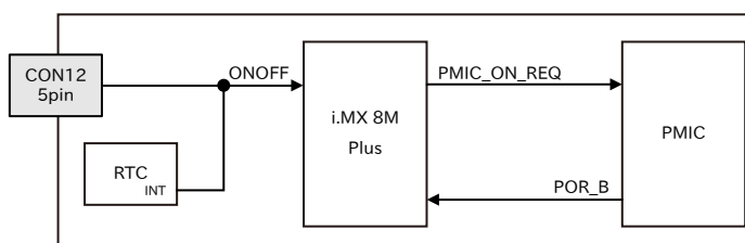
図 3.60 ONOFF 回路の構成
