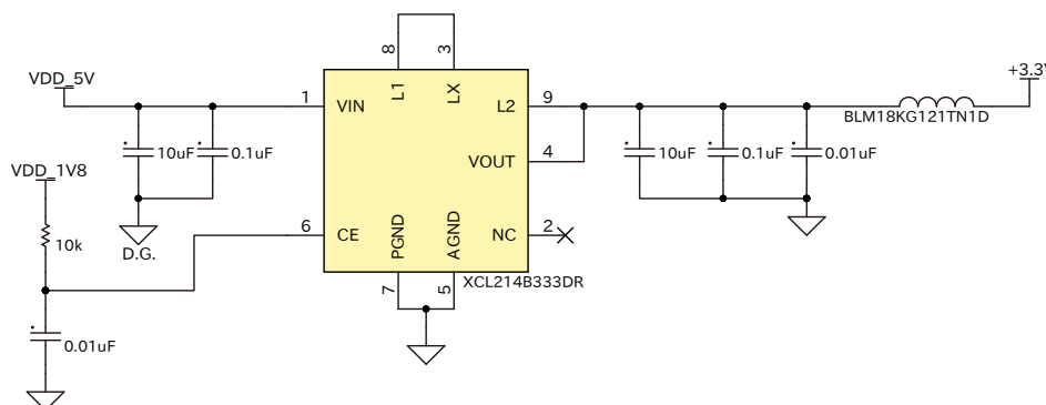
図 3.54 DC/DC コンバータ回路(VDD_5V 入力、3.3V 1.5A 出力)例
