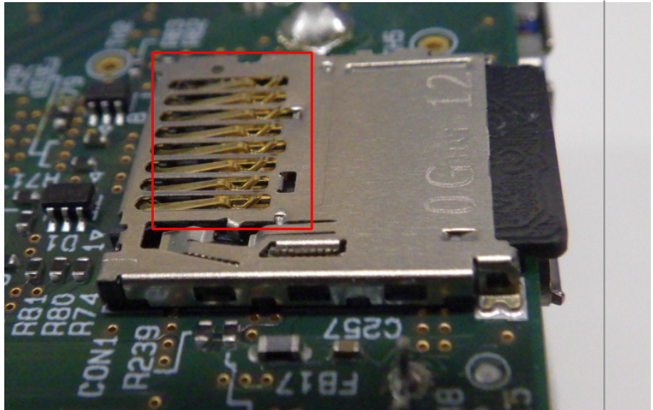
図 3.81 CON1 microSD スロット 取り扱い上の注意事項
