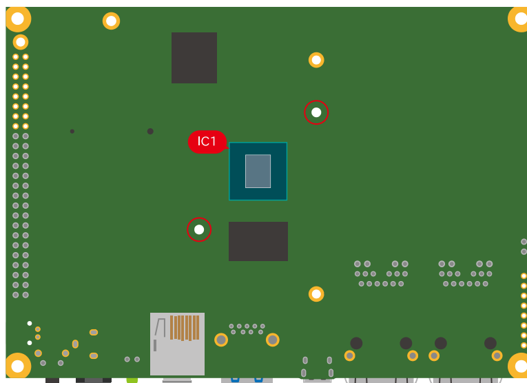
図 3.48 Armadillo-IoT ゲートウェイ G4 の IC1 とヒートシンク固定穴の位置
