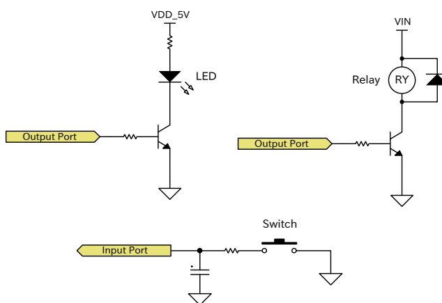
図 3.53 スイッチ、LED、リレー接続例
