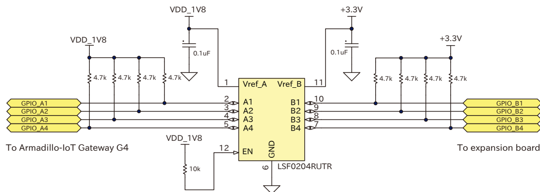
図 3.55 1.8V ↔ 3.3V 双方向レベル変換回路の例
