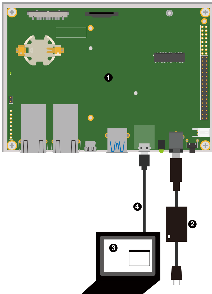
図 3.40 シリアルコンソールを使用する配線例
