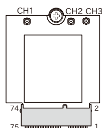
図 3.92 WLAN+BT コンボモジュール アンテナケーブル接続用レセプタクルの配置
