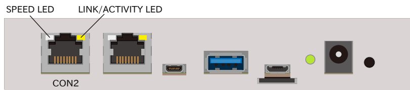
図 3.82 CON2 LAN LED 配置
