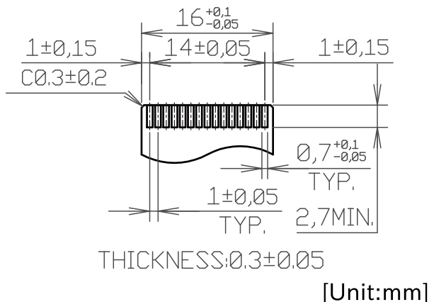
図 3.100 CON10 接続可能なフレキシブルフラットケーブルの形状
