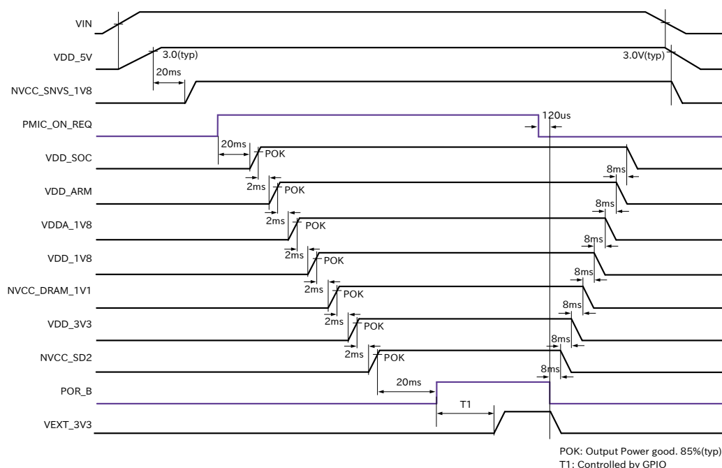
図 3.57 電源シーケンス
