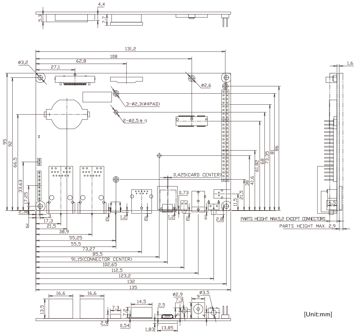
図 3.61 基板形状図
