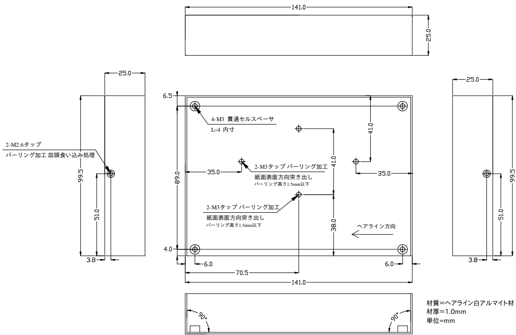
図 6.247 LAN モデル ケース(下)形状図
