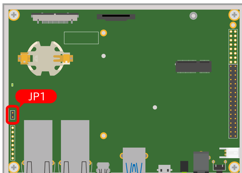
図 3.18 JP1 の位置
