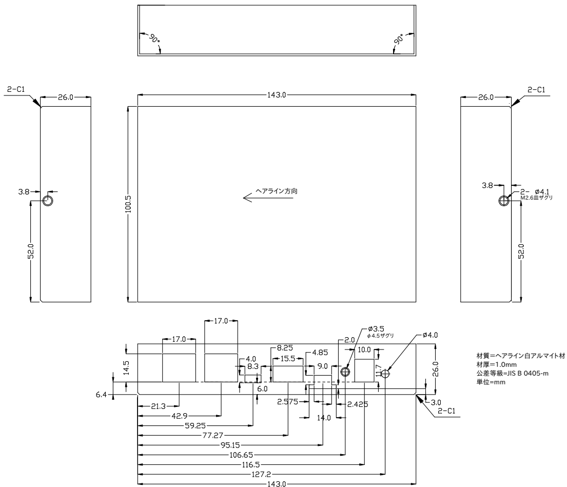
図 6.246 LAN モデル ケース(上)形状図
