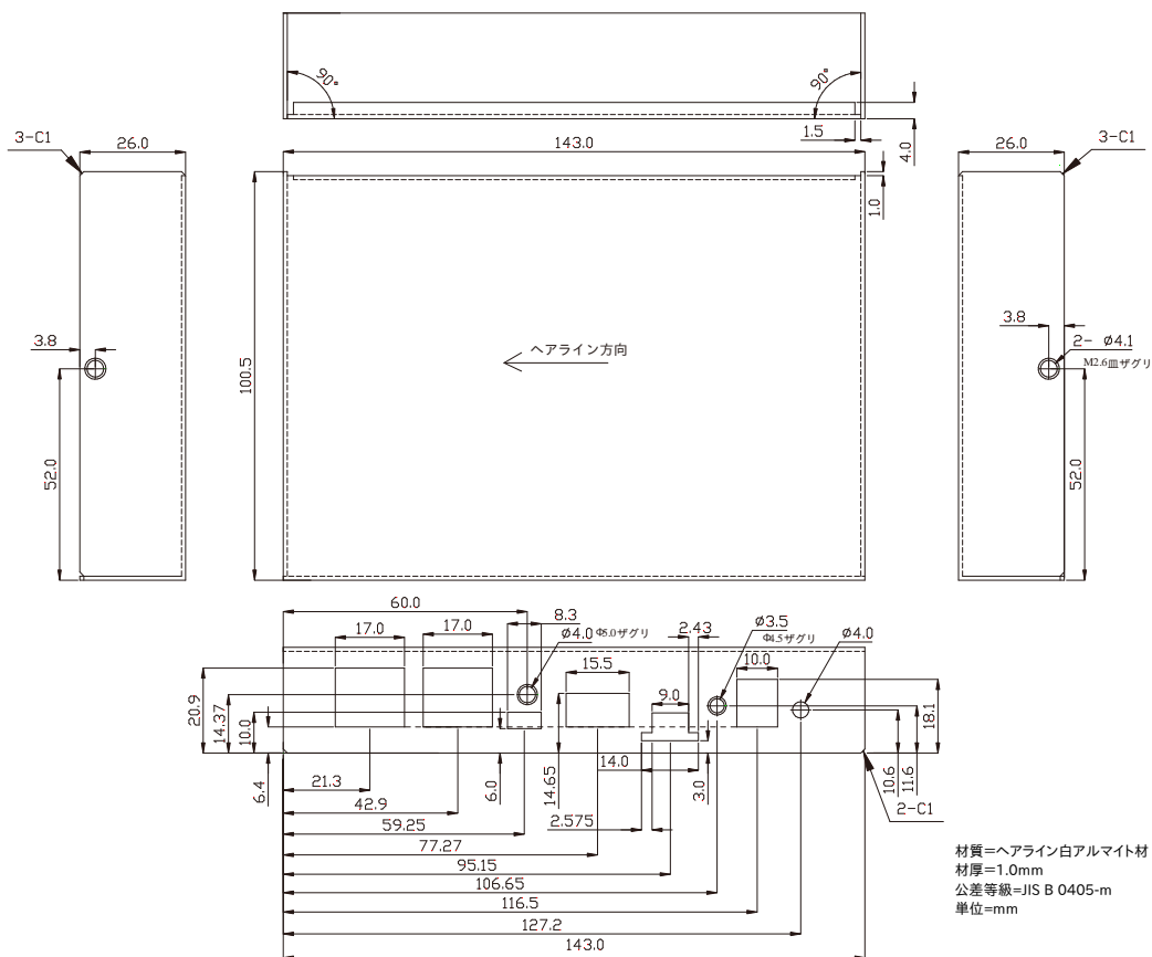
図 6.252 LTE+WLAN モデル ケース(上)形状図
