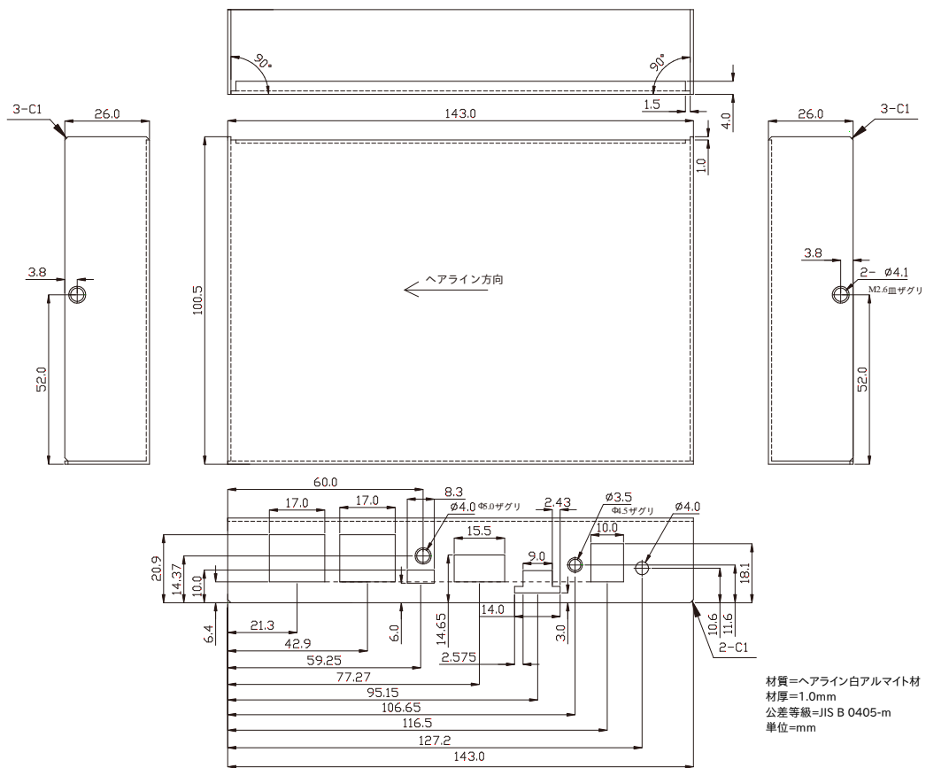
図 6.248 LTE モデル ケース(上)形状図
