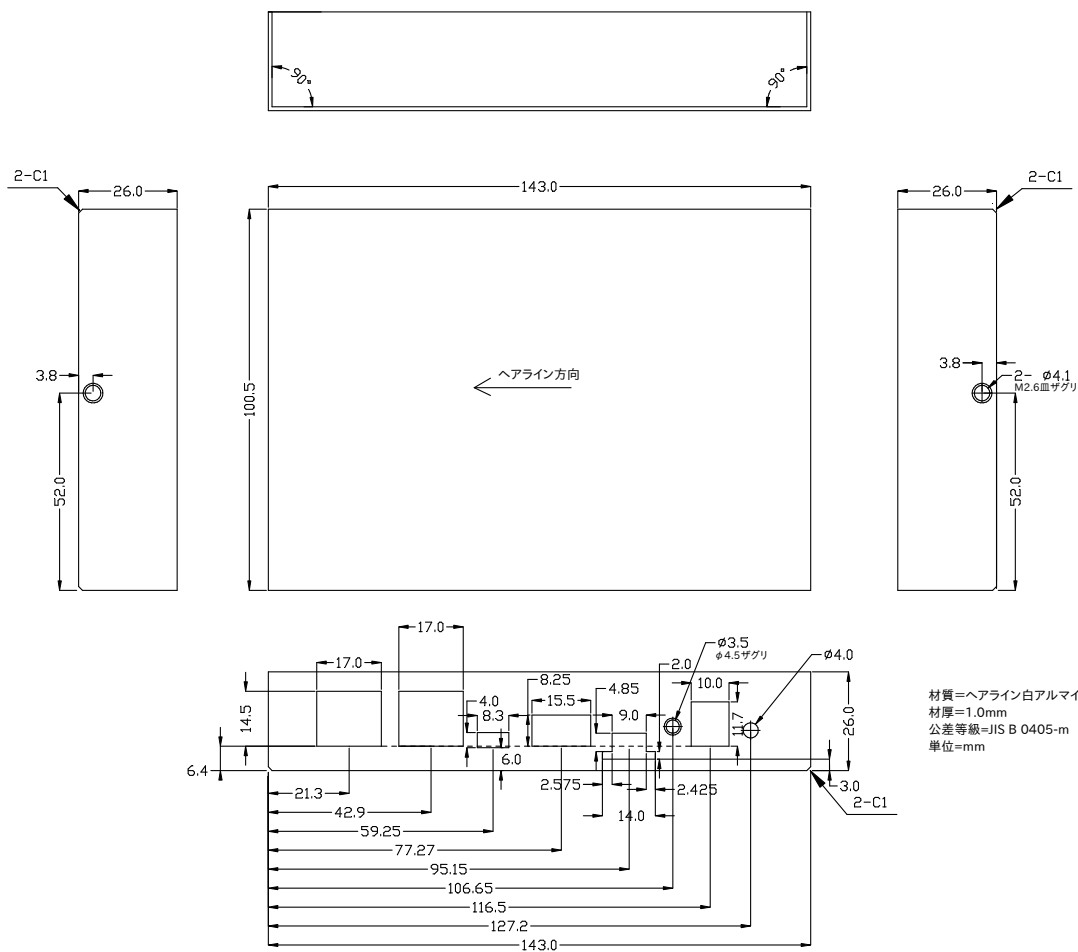
図 6.250 WLAN モデル ケース(上)形状図
