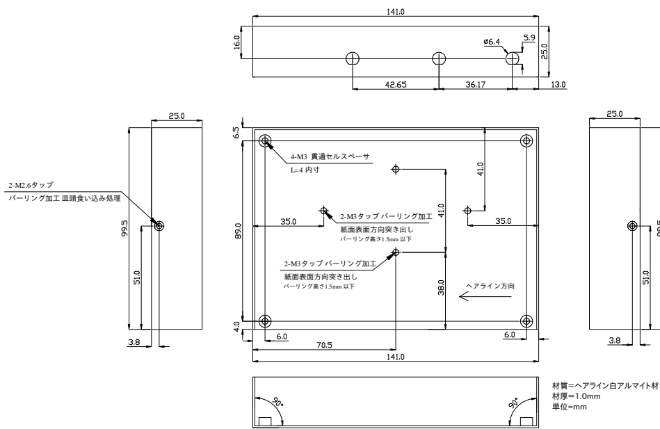
図 6.251 WLAN モデル ケース(下)形状図
