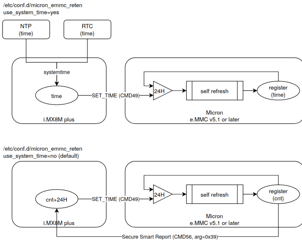
図 6.237 データリテンション開始トリガーの方式
