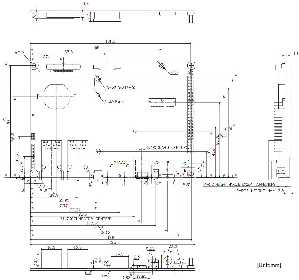
図 6.231 基板形状図
