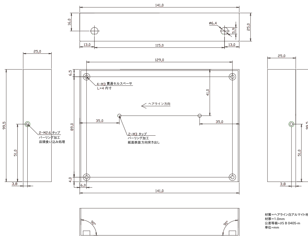
図 14.30 LTE モデル ケース(下)形状図
