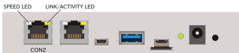
図 14.9 CON2 LAN LED 配置
