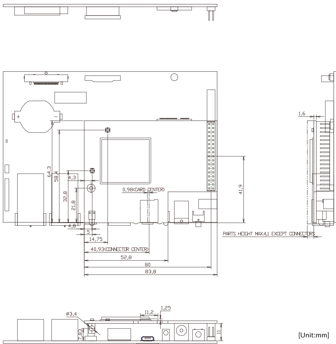
図 14.14 基板形状図(LTE モデル 追加分)
