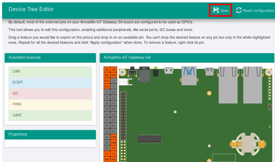
図 9.156 DTS/DTB の生成
