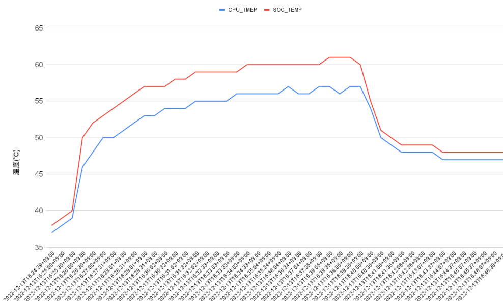
図 10.266 Armadillo-IoT ゲートウェイ G4 で取得した温度のグラフ
