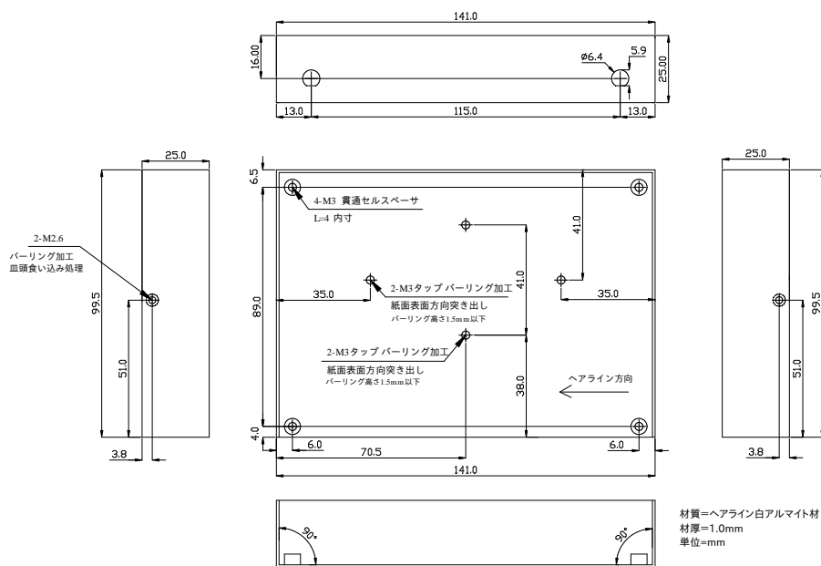
図 14.32 LTE モデル ケース(下)形状図
