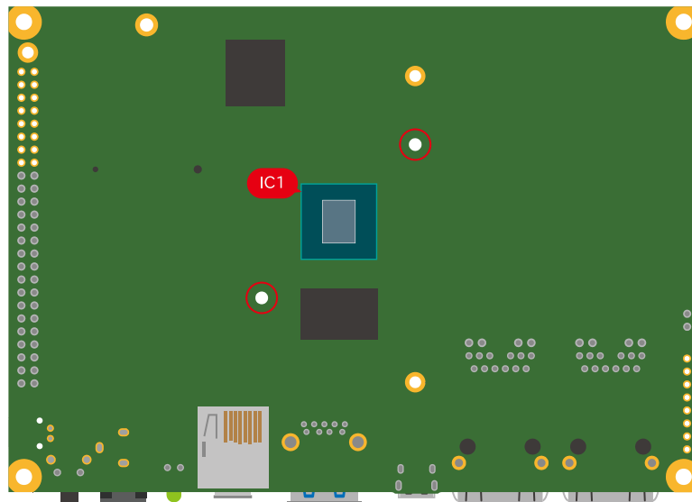
図 14.16 Armadillo-IoT ゲートウェイ G4 の IC1 とヒートシンク固定穴の位置
