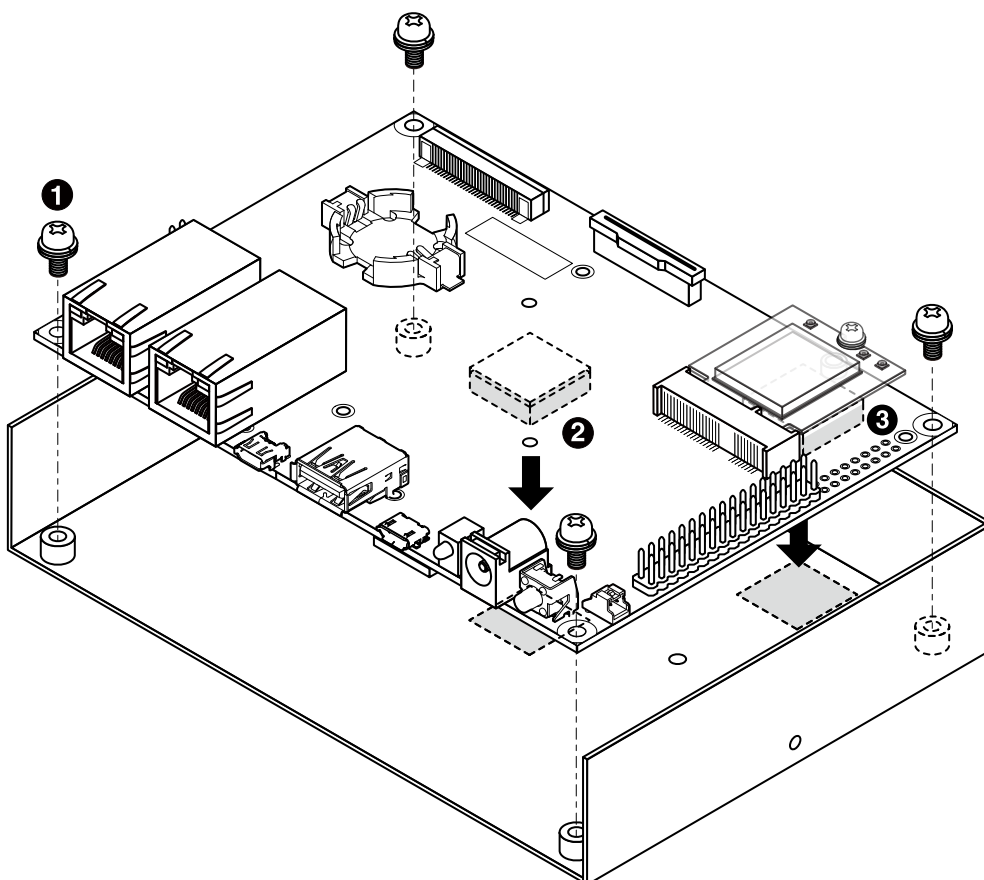
図 14.26 オプションケース(金属製) ケース(下)ねじ止め
