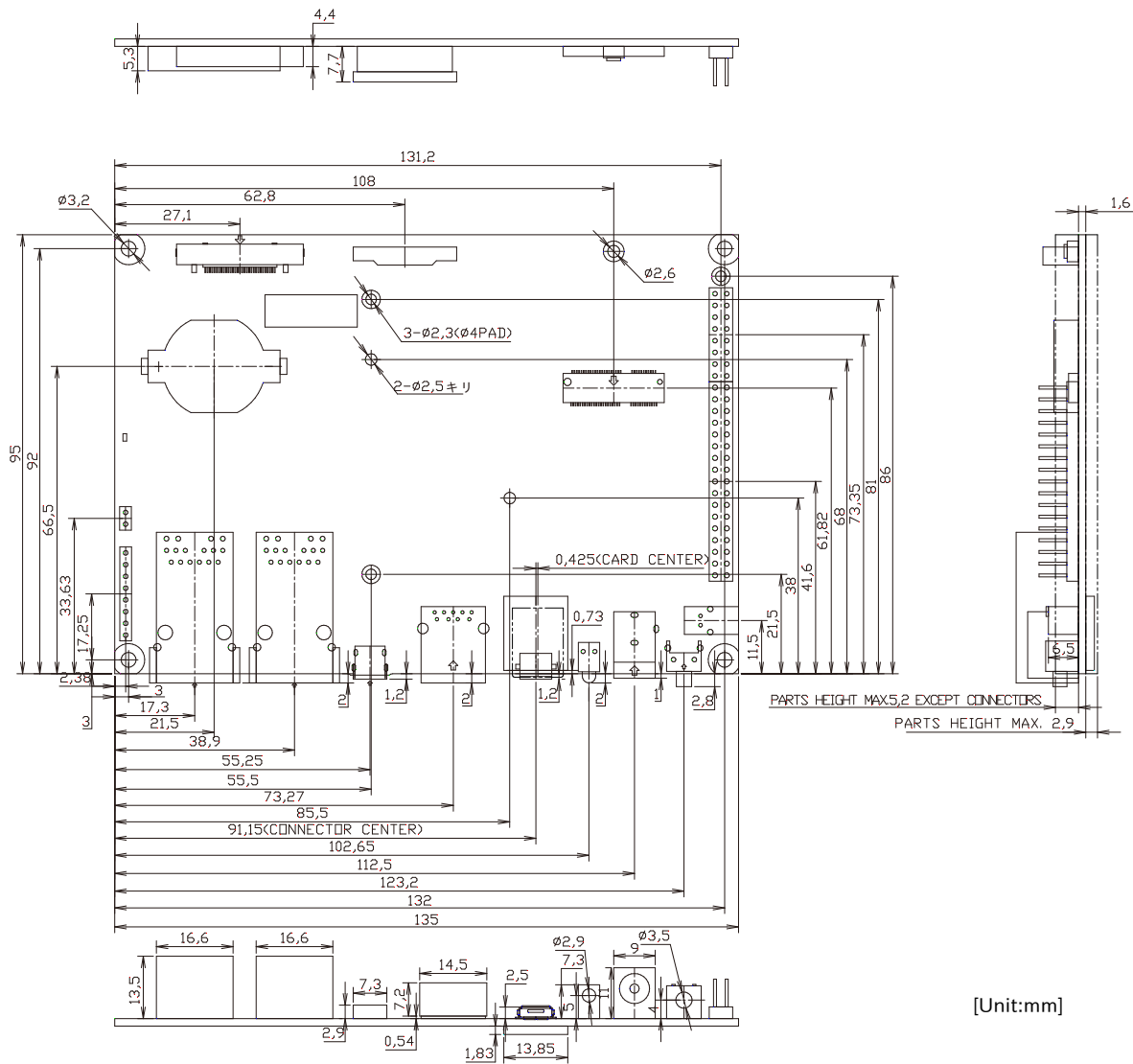
図 14.14 基板形状図
