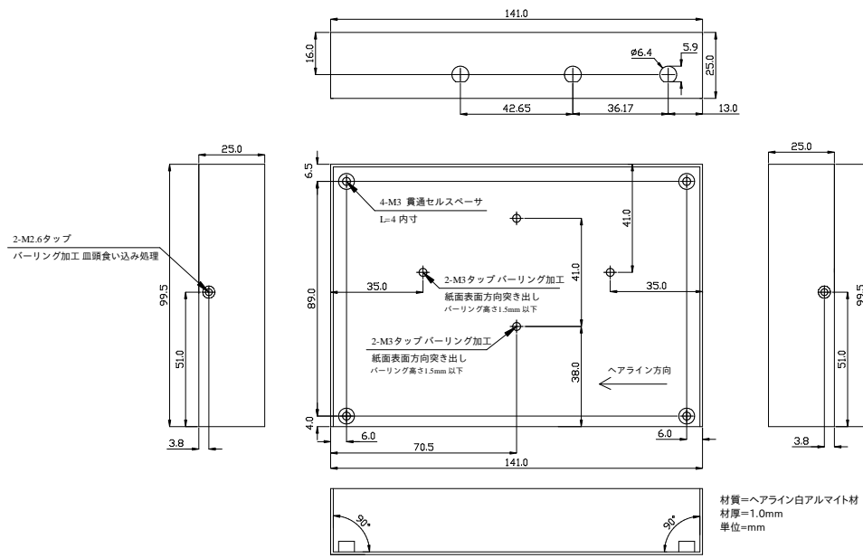
図 14.34 WLAN モデル ケース(下)形状図
