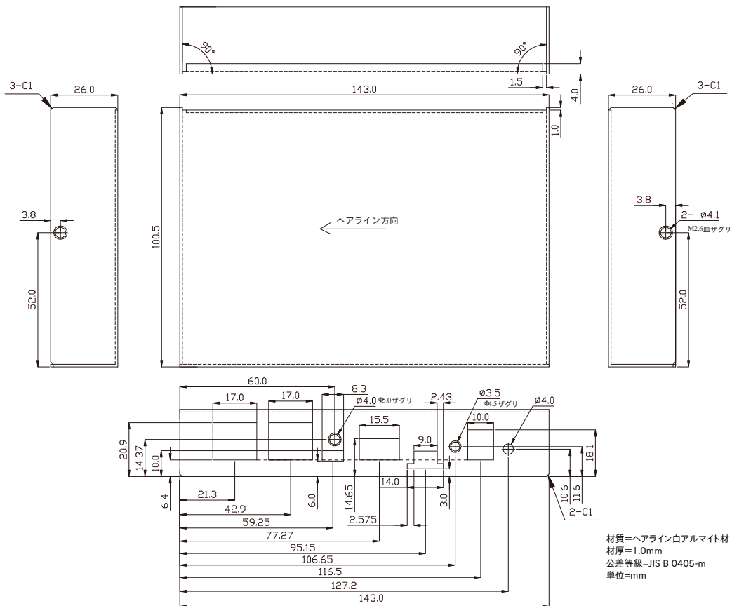
図 14.35 LTE+WLAN モデル ケース(上)形状図
