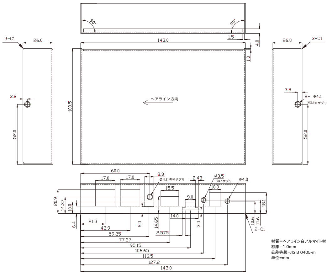
図 14.31 LTE モデル ケース(上)形状図
