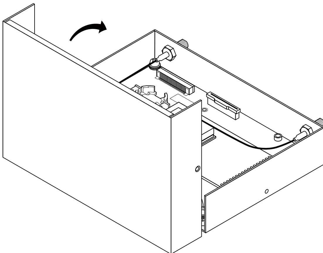
図 14.27 オプションケース(金属製) ケース嵌め合わせ
