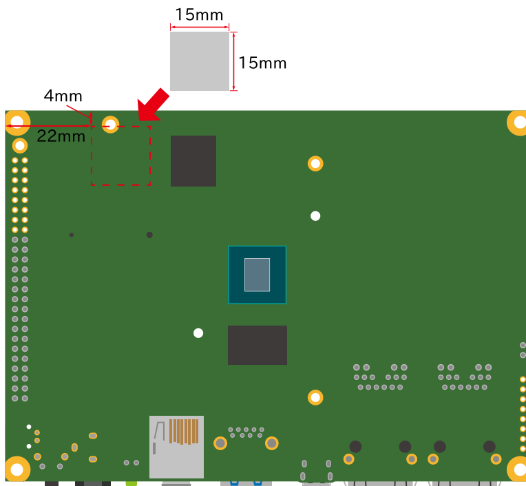
図 14.25 オプションケース(金属製) 放熱シート貼付(WLAN+BT コンボモジュール搭載モデル)
