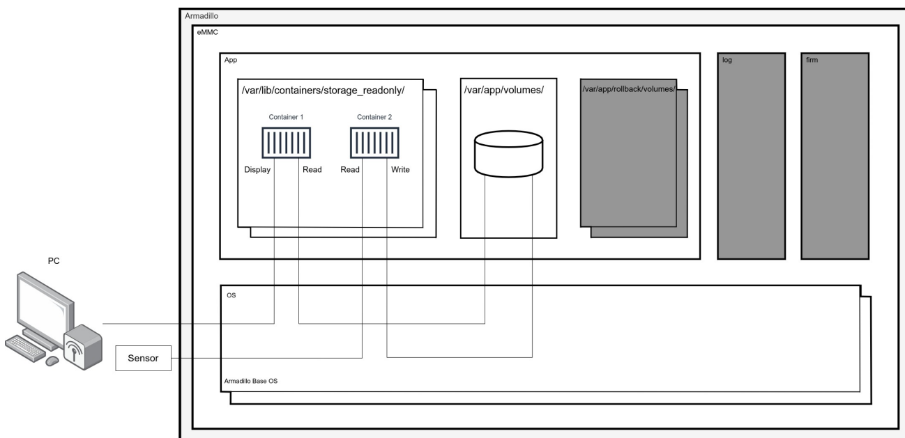
図 11.9 センサから読み取ったデータを PC に出力するシステム構成図
