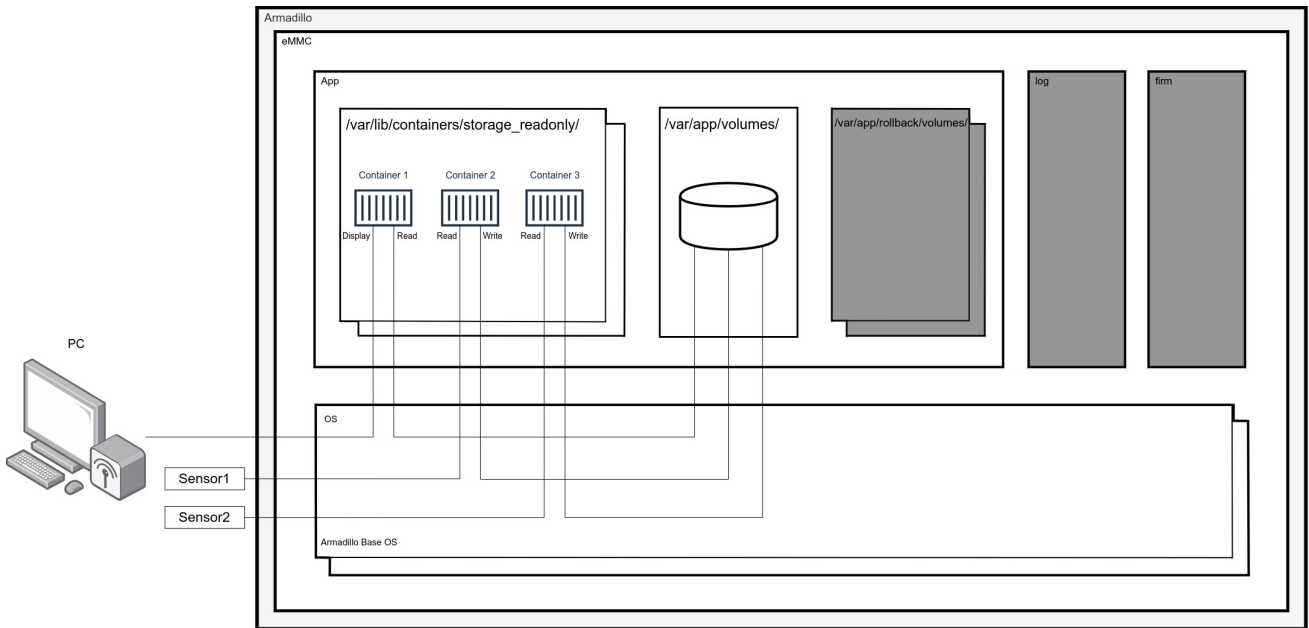
図 11.11 複数のセンサからデータを読み取るシステム構成図
