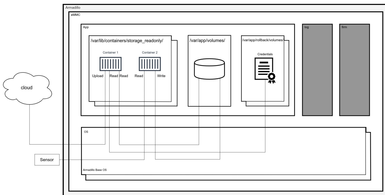
図 11.10 センサからデータを読み取りクラウドに出力するシステム構成図
