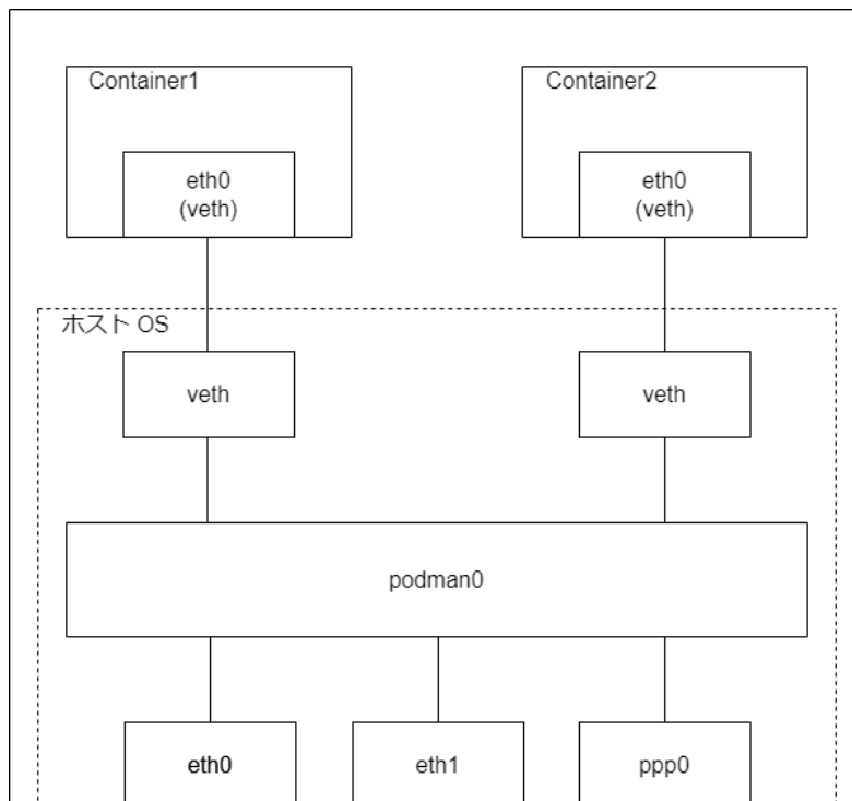
図 11.24 ブリッジモードの構成
