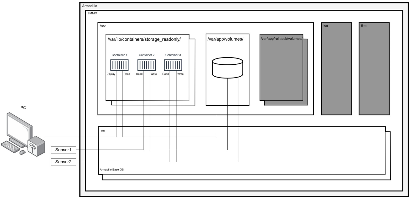
図 11.16 複数のセンサからデータを読み取るシステム構成図
