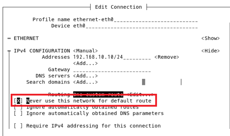
図 11.44 nmtui デフォルトゲートウェイ無効化
