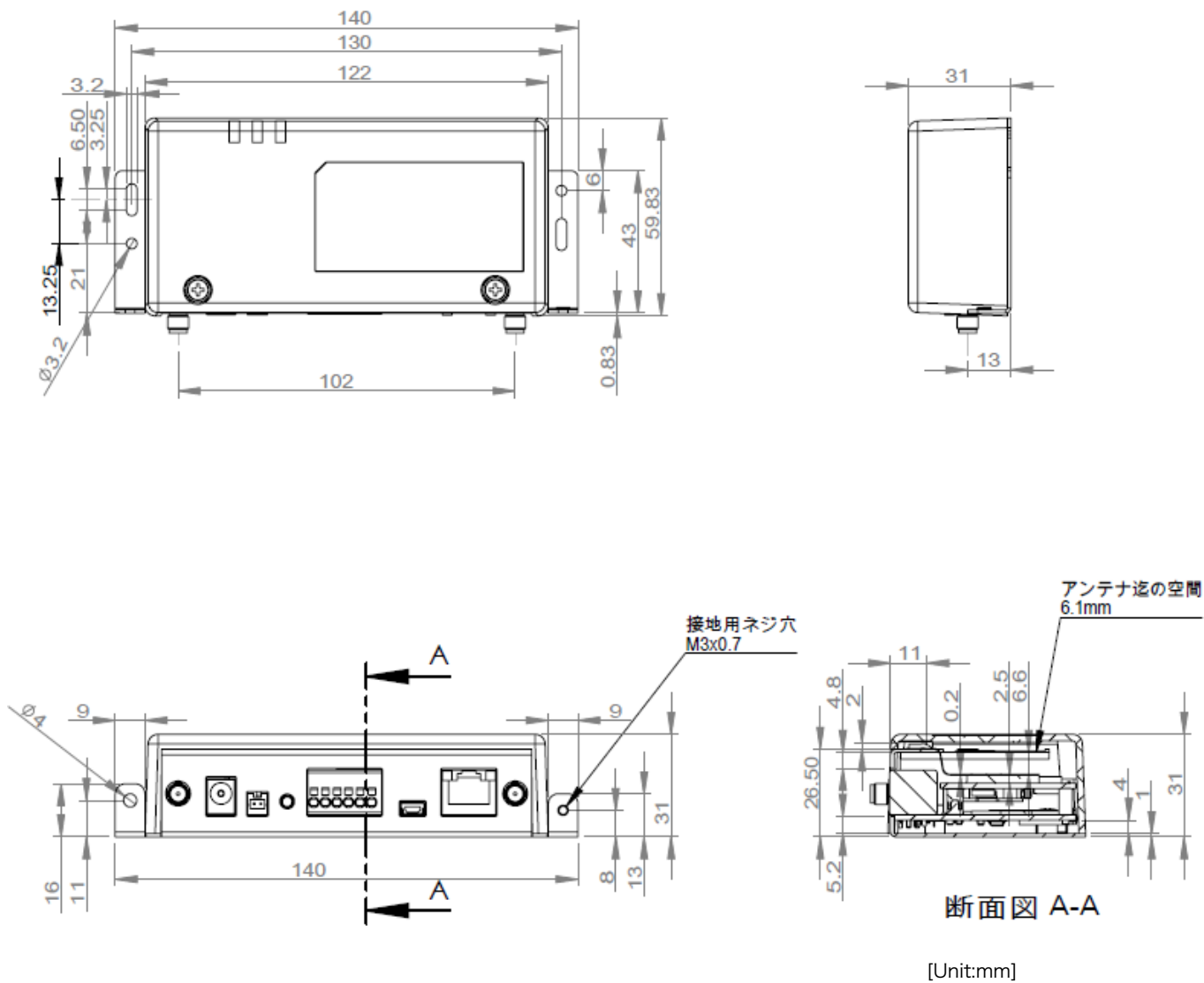
図 5.1 筐体形状図
