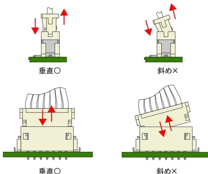
図 17.5 挿抜角度
