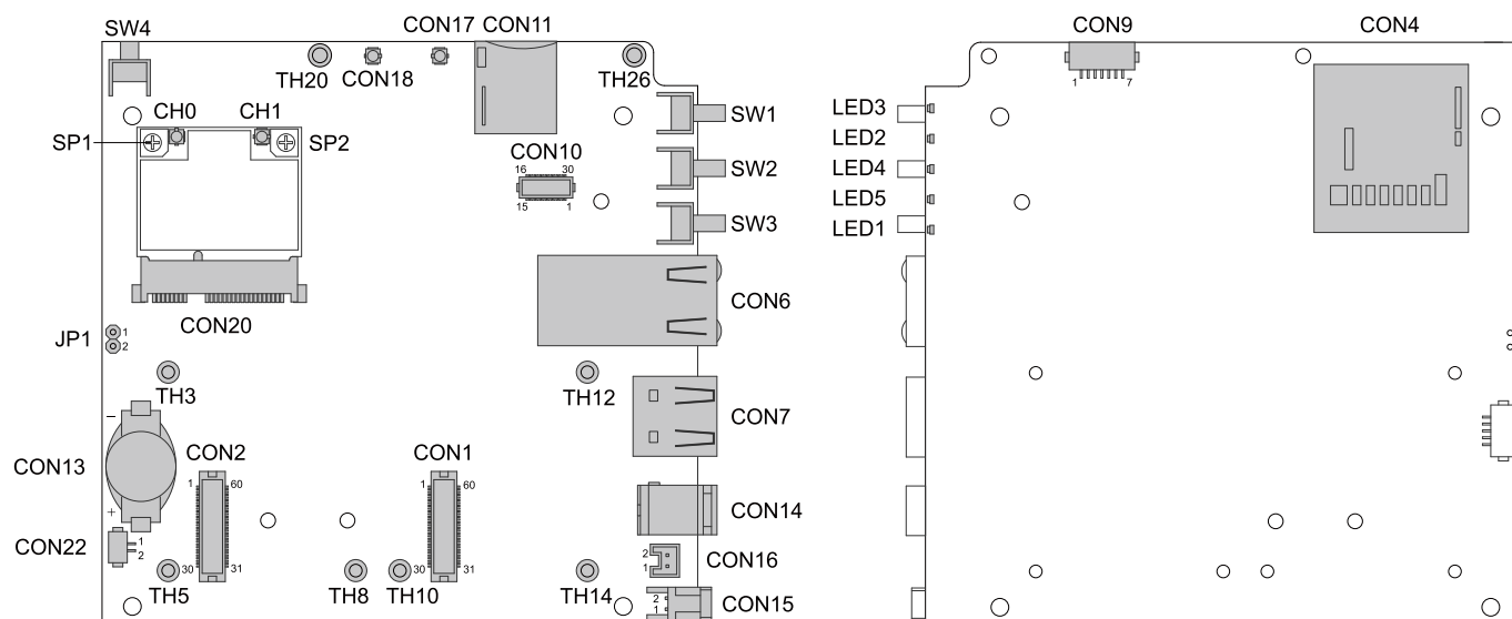
図 4.11 インターフェースレイアウト図(AEH-AR9462 搭載) [3]
