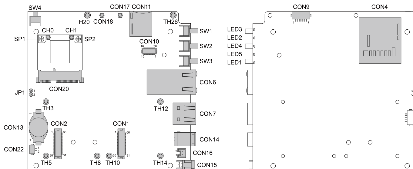
図 4.12 インターフェースレイアウト図(WPEB-265AXI(BT) [B33] 搭載) [4]
