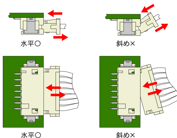
図 4.14 挿抜角度
