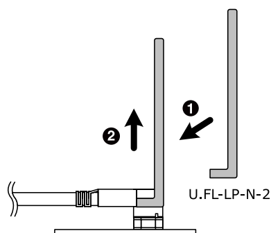
図 20.17 外付けアンテナケーブルの引き抜き方法
