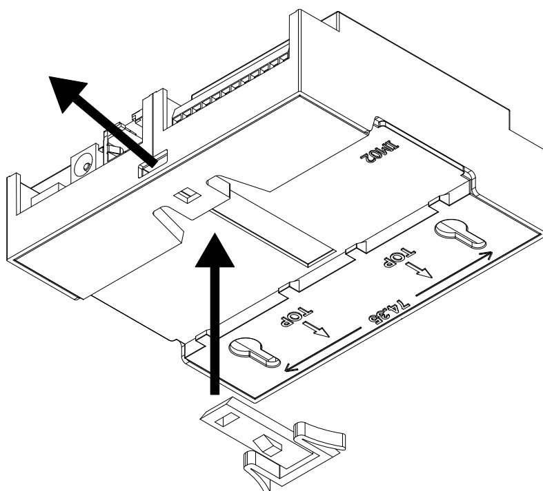
図 3.66 フック取り付け 1
