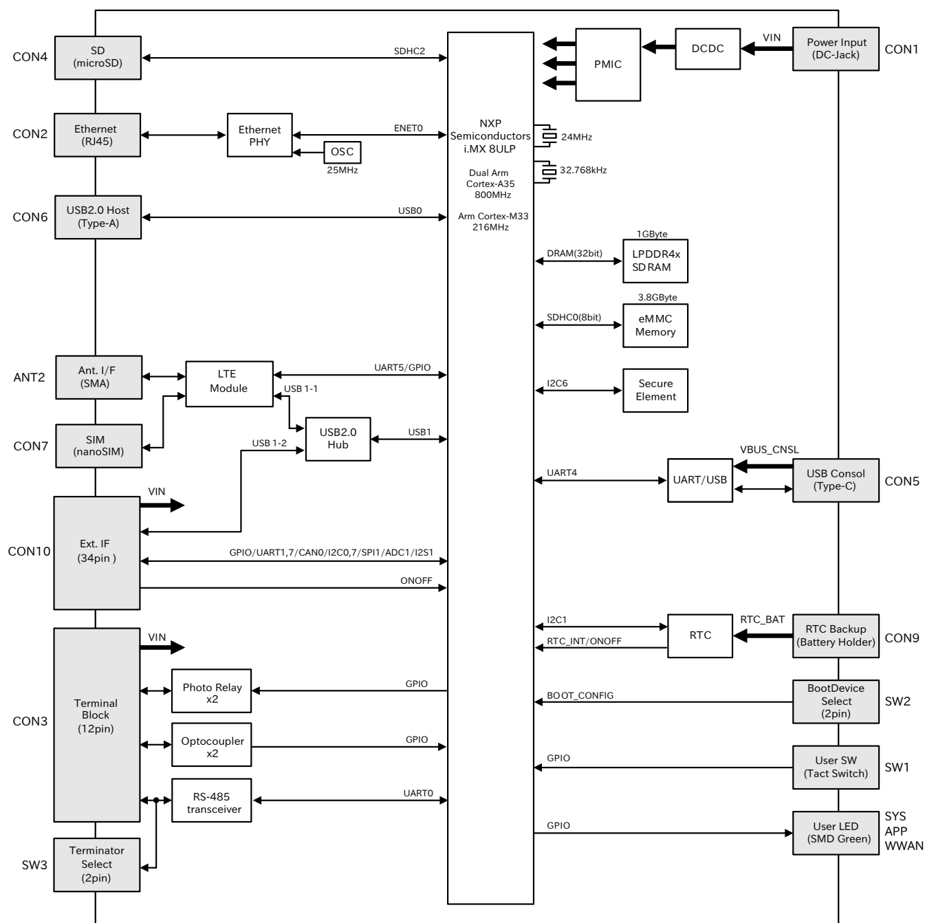
図 2.12 ブロック図(AG9120-C02Z)
