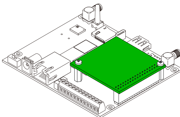
図 3.53 垂直方向に拡張基板を配置した場合の接続イメージ
