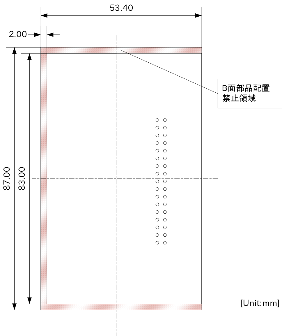
図 3.54 水平方向に拡張する場合の部品搭載制限(B 面側)
