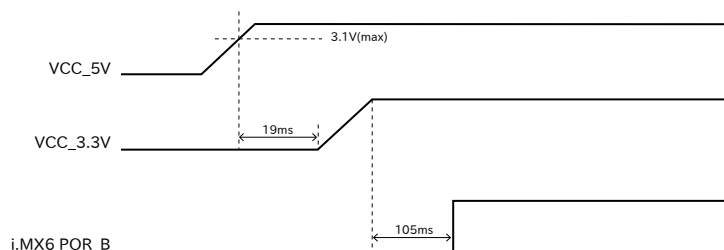
図 3.56 電源シーケンス
