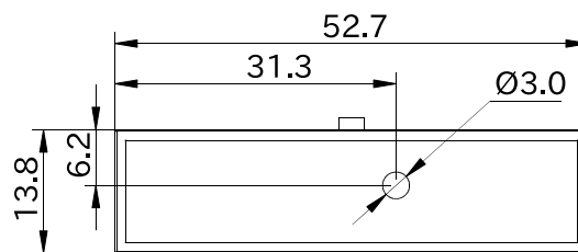
図 6.282 形状図 カバーパーツ A (アンテナ穴有り)
