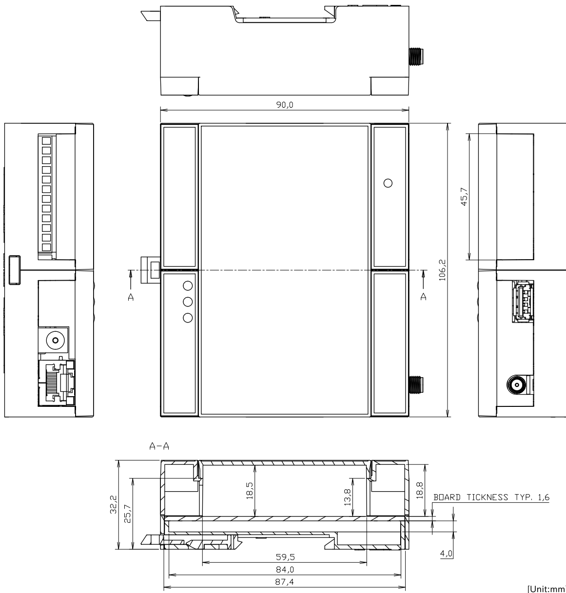
図 3.63 ケース形状図(スタンダードタイプ)
