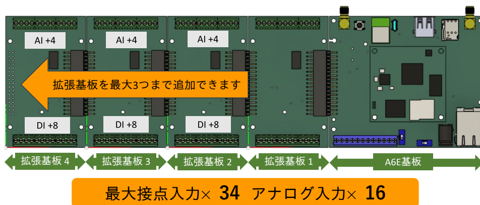
図 6.291 +Di8+Ai4 拡張基板のカスケード接続
