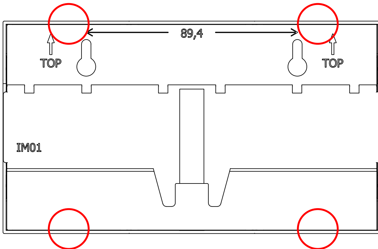
図 3.77 ケースボトムの子メ(+Di8+Ai4 タイプ)
