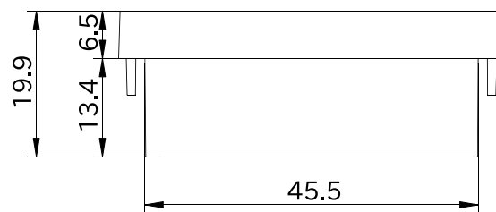
図 6.283 形状図 カバーパーツ A (アンテナ穴無し)
