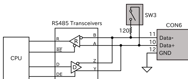
図 3.123 RS-485 内部回路
