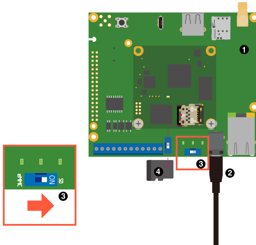
図 3.13 Armadillo-IoT ゲートウェイ A6E を初期化する接続
