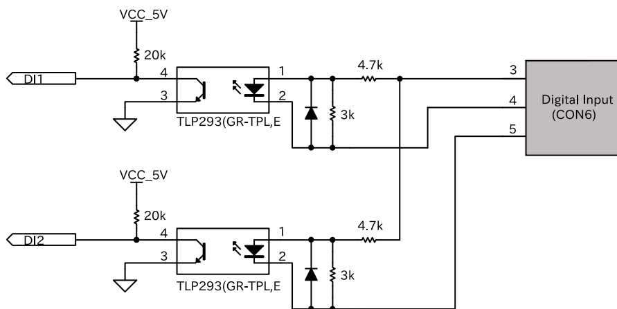
図 3.131 接点入力(CON6) 内部回路
