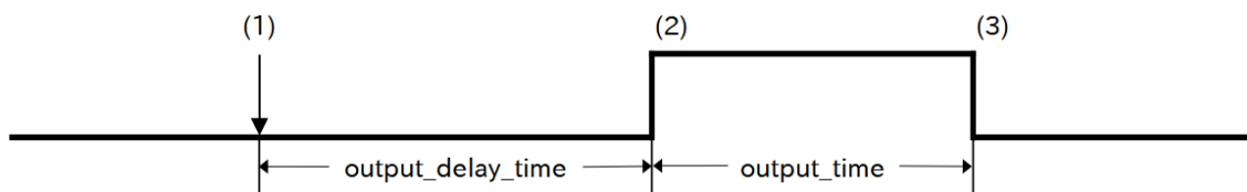
図 3.236 DO の出力タイミング
