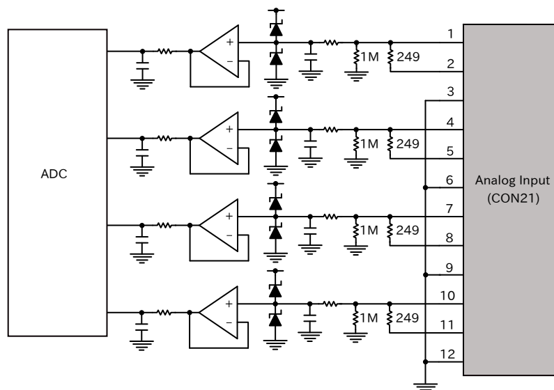
図 3.143 アナログ入力(CON21) 内部回路
