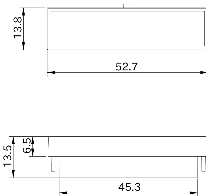
図 6.286 形状図 カバーパーツ C
