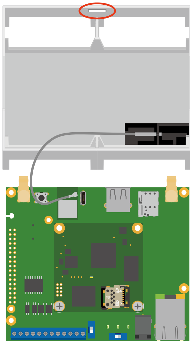
図 3.89 WLAN 基板アンテナの貼り付け位置 (スタンダードタイプ WLAN モデル)
