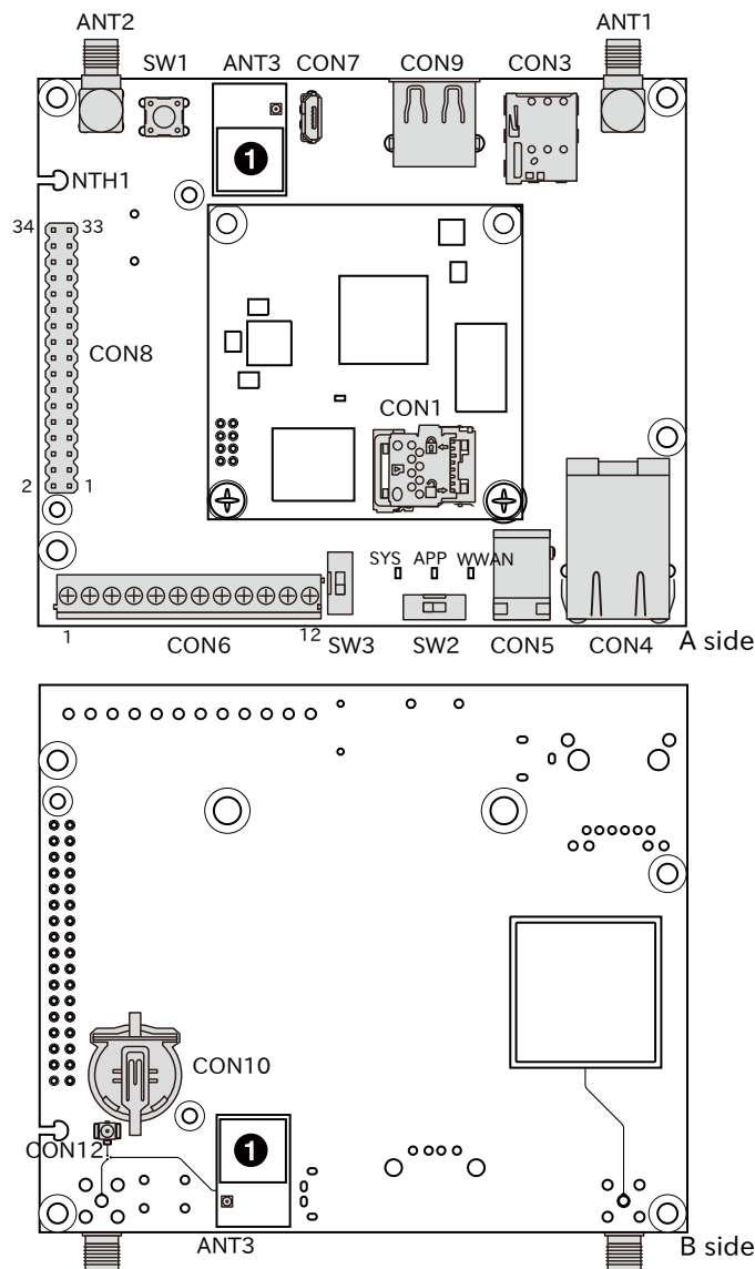
図 3.92 Armadillo-IoT ゲートウェイ A6E のインターフェース (スタンダードタイプ)
