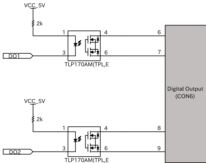
図 3.139 接点出力(CON6) 内部回路
