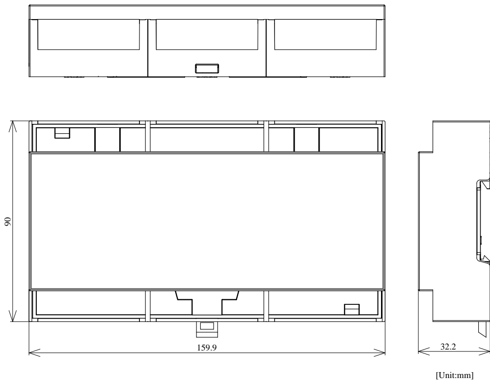
図 6.280 形状図 ケース外形(トップとボトムを組み合わせた状態)
