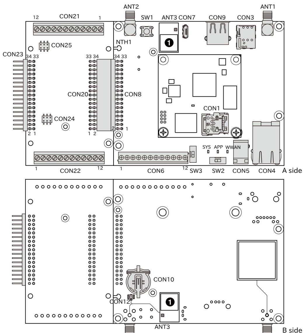
図 3.93 Armadillo-IoT ゲートウェイ A6E のインターフェース (+Di8+Ai4 タイプ)
