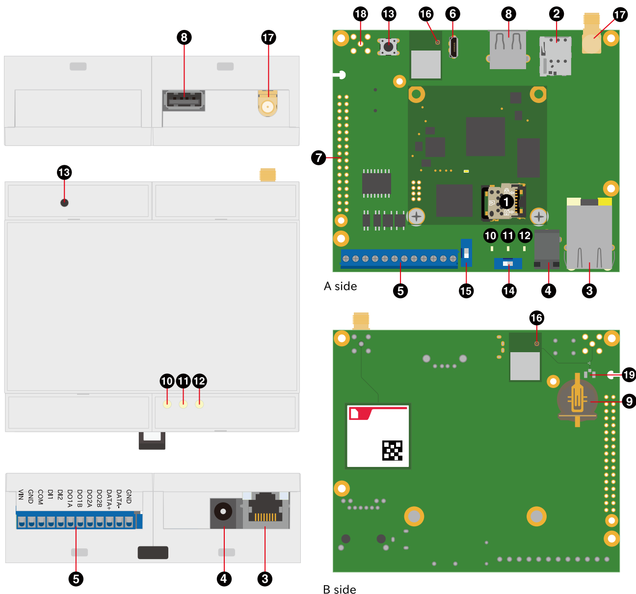
図 2.12 Armadillo-IoT ゲートウェイ A6E インターフェースレイアウト (スタンダードタイプ)
