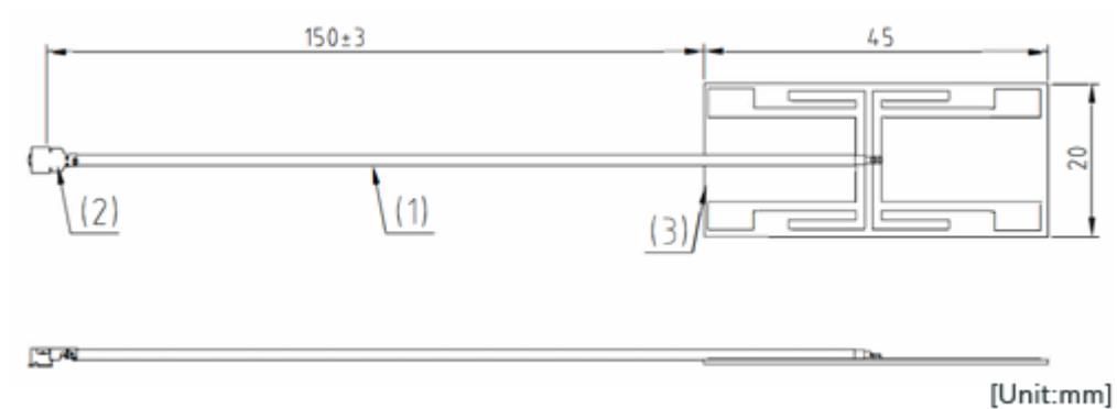
図 3.65 WLAN 基板アンテナ形状図(Cat.1 bis+WLAN モデル)
