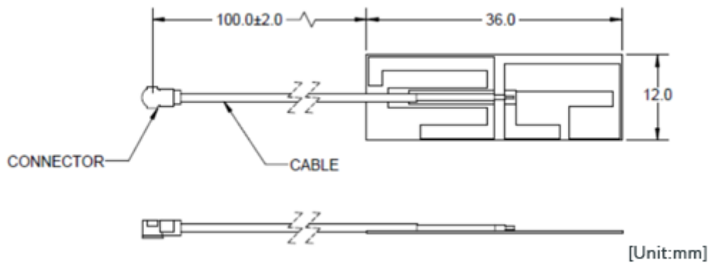
図 3.66 WLAN 基板アンテナ形状図(WLAN モデル)
