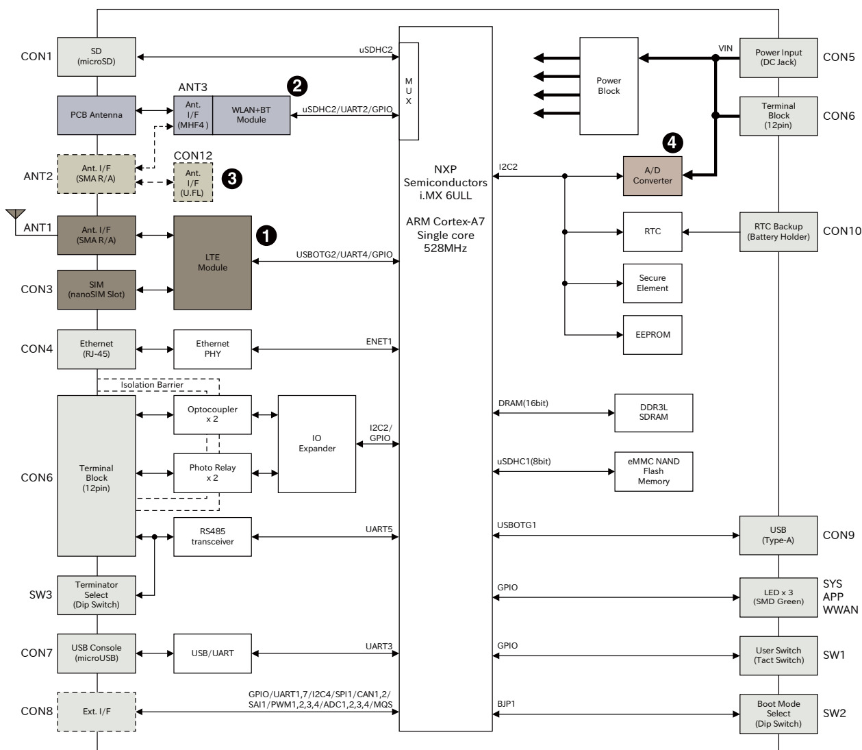
図 2.14 ブロック図 (スタンダードタイプ)
