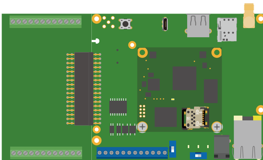
図 3.50 水平方向に拡張基板を配置した場合の接続例
