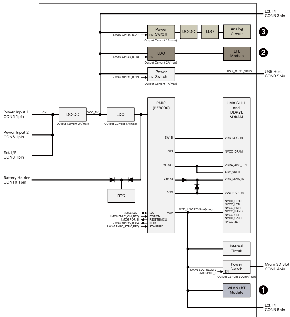
図 3.55 電源回路の構成
