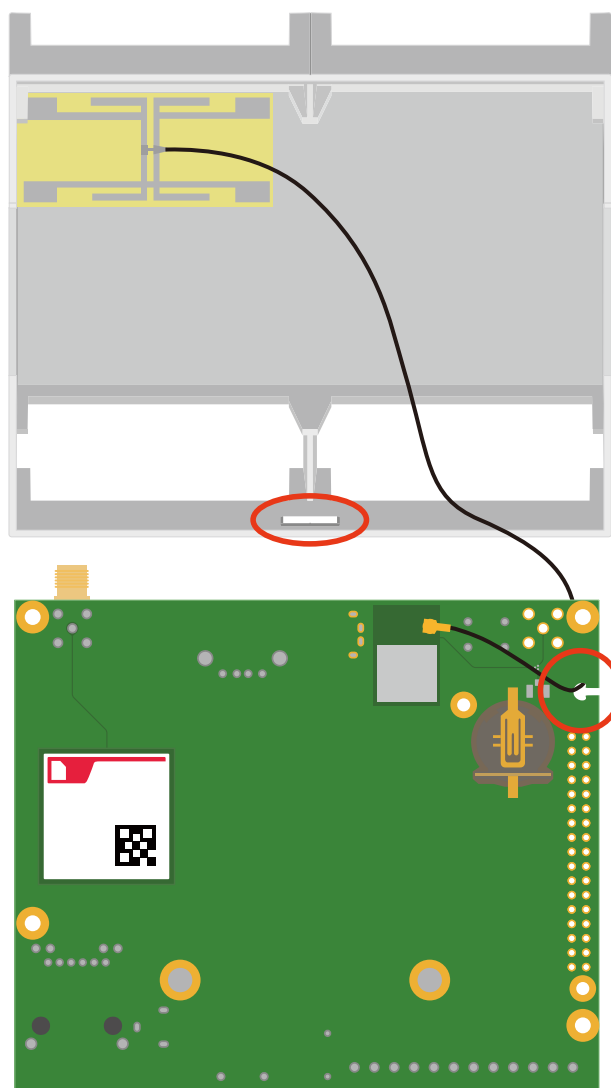
図 3.87 WLAN 基板アンテナの貼り付け位置 (スタンダードタイプ Cat.1 bis+WLAN モデル)
