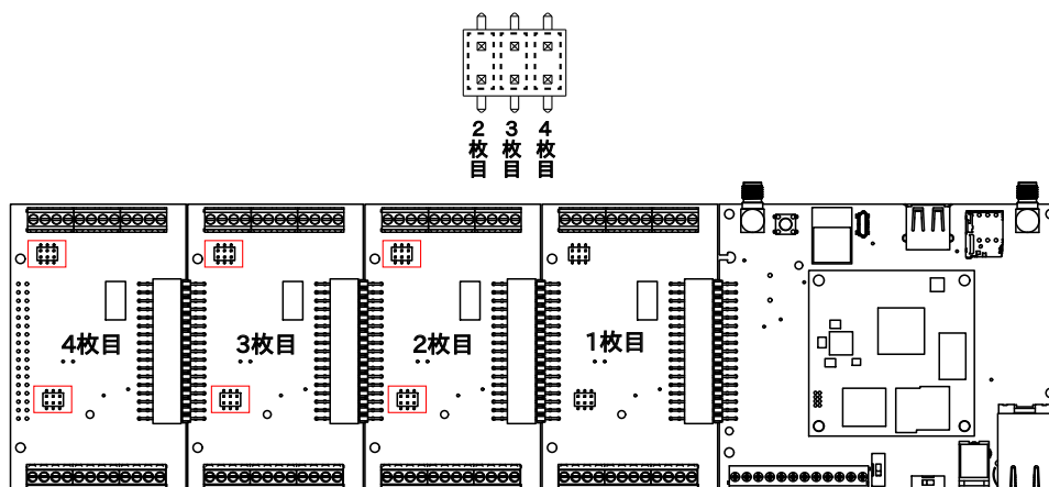
図 6.294 ピンヘッドの位置と設定
