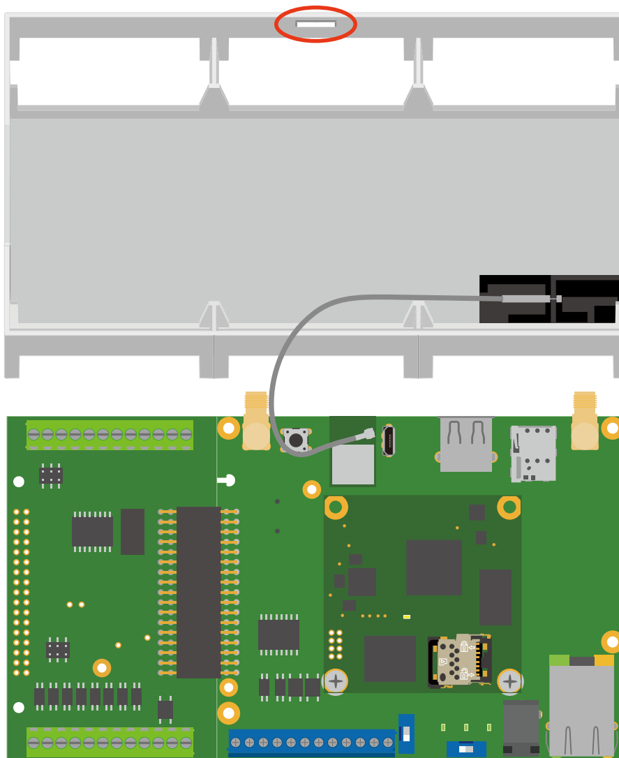
図 3.90 WLAN 基板アンテナの貼り付け位置 (+Di8+Ai4 タイプ WLAN モデル)
