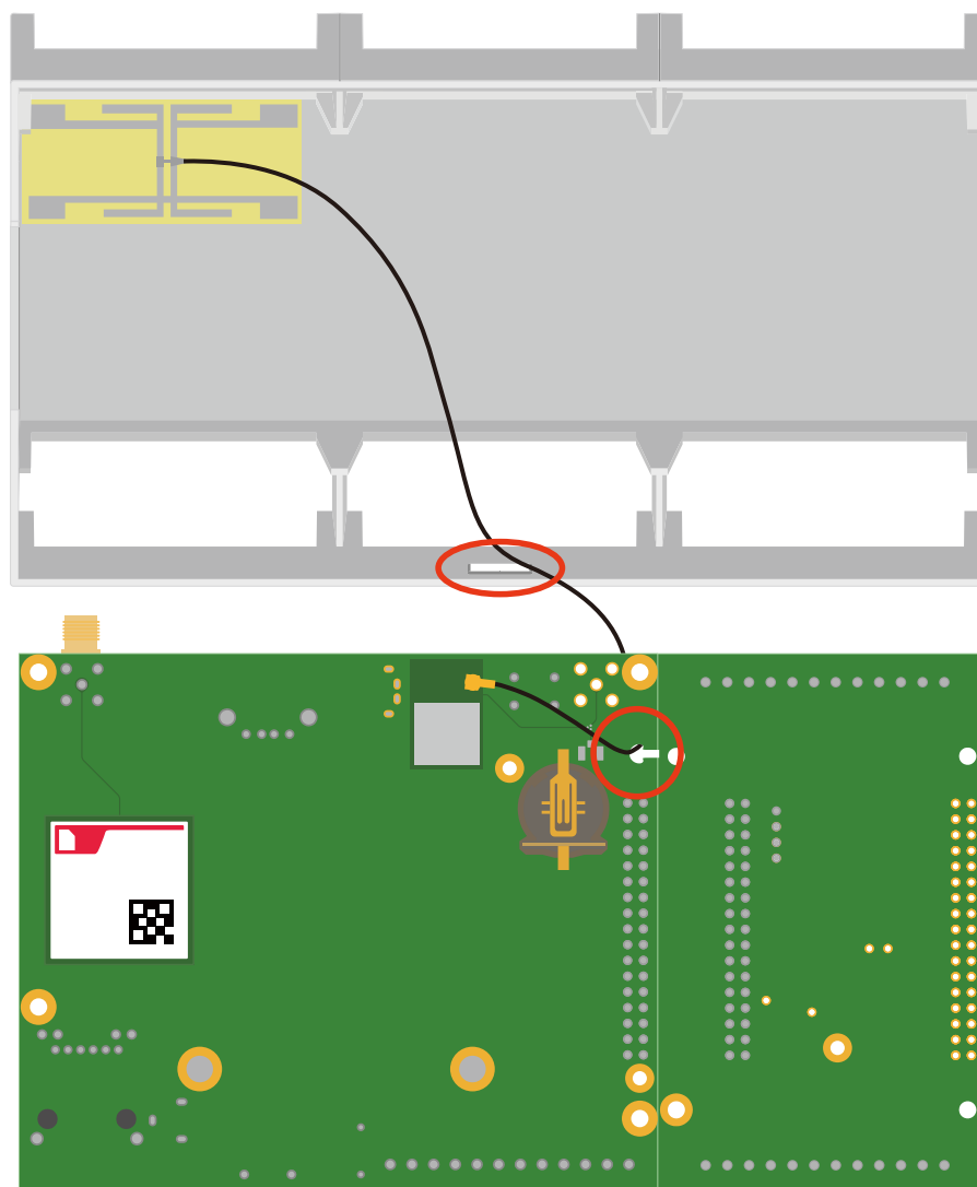
図 3.88 WLAN 基板アンテナの貼り付け位置 (+Di8+Ai4 タイプ Cat.1 bis+WLAN モデル)
