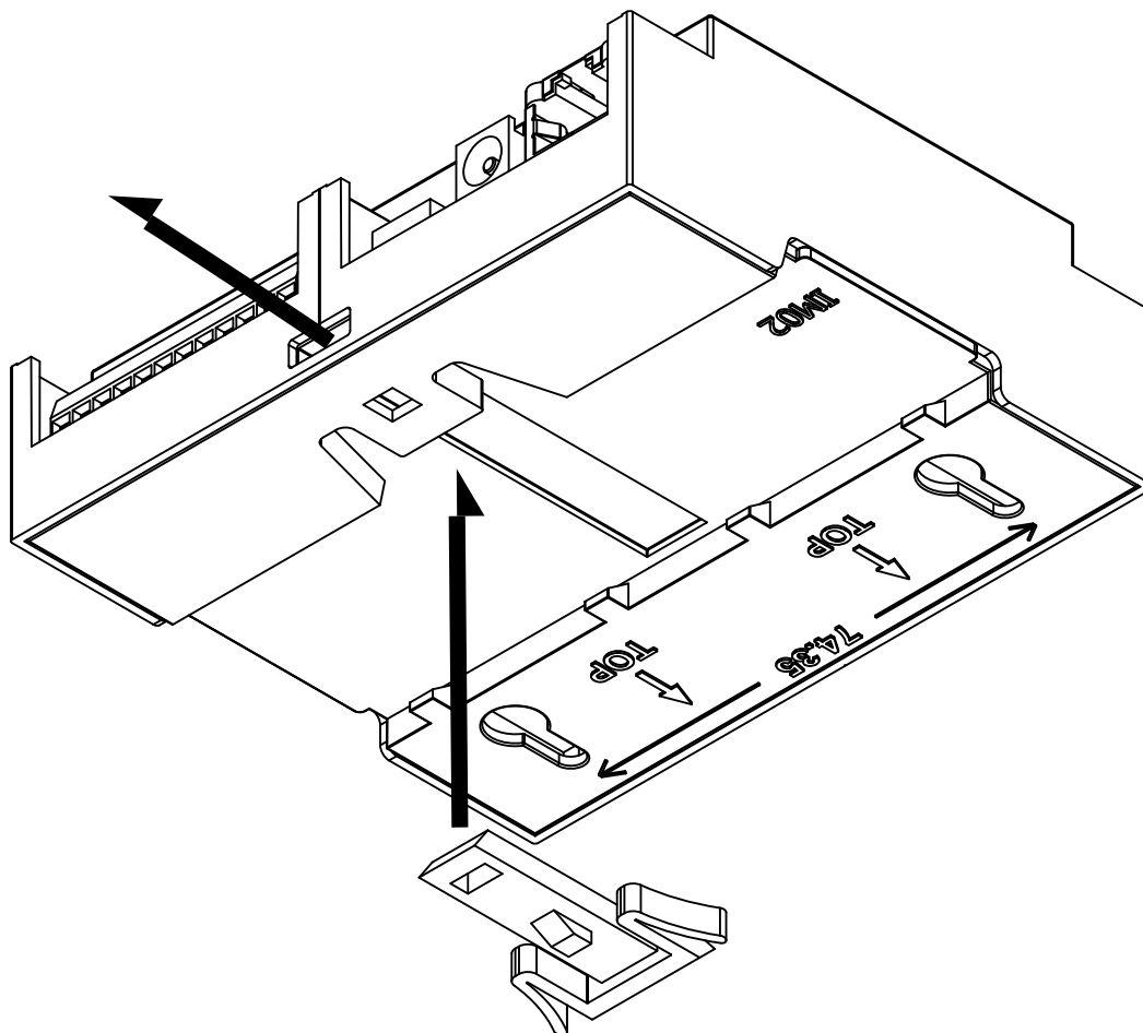
図 3.69 フック取り付け 1 (スタンダードタイプ)
