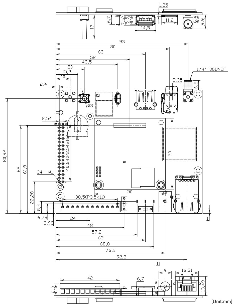
図 3.58 コネクタ、スイッチ、LED 位置(スタンダードタイプ)
