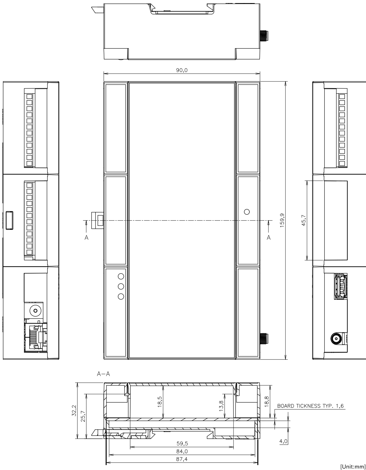
図 3.64 ケース形状図(+Di8+Ai4 タイプ)
