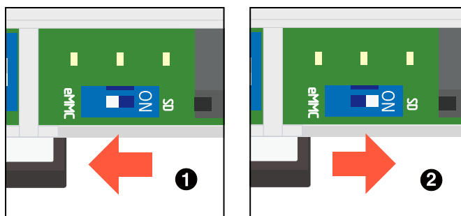
図 3.180 スイッチの状態と起動デバイス
