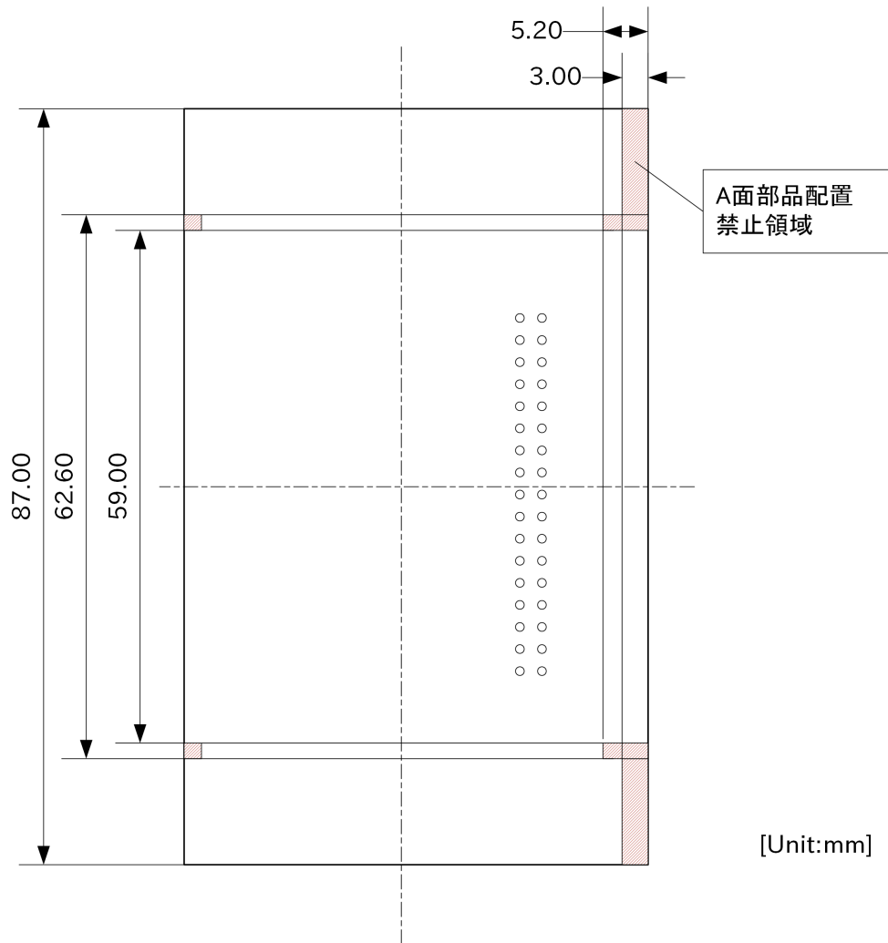
図 3.53 水平方向に拡張する場合の部品搭載制限(A 面側)
