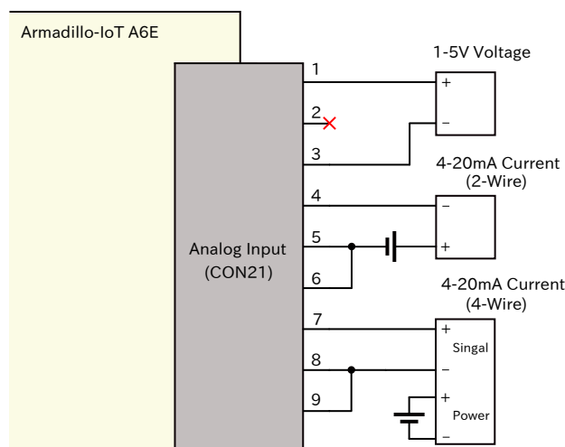
図 3.144 アナログ入力(CON21) 接続例
