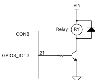
図 3.48 ピンを出力専用で使用した回路例
