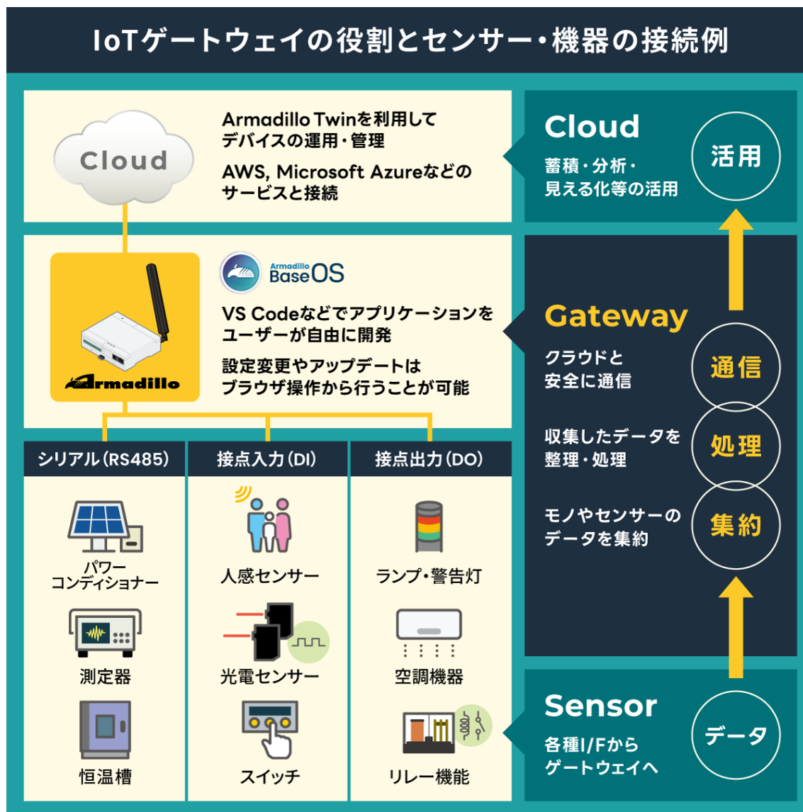
図 2.2 様々なデバイスとの接続例
