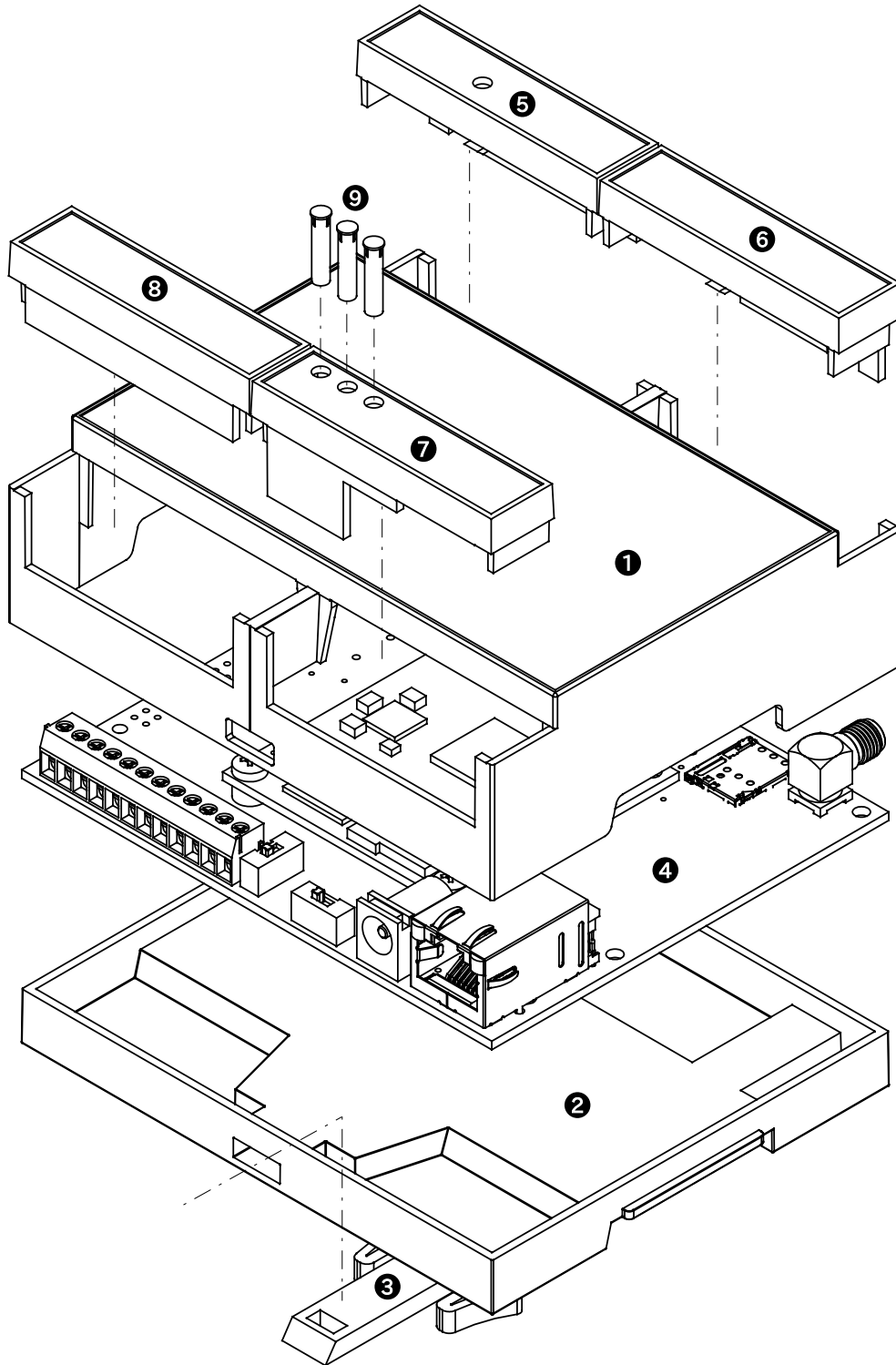
図 3.68 ケース展開図 (スタンダードタイプ)
