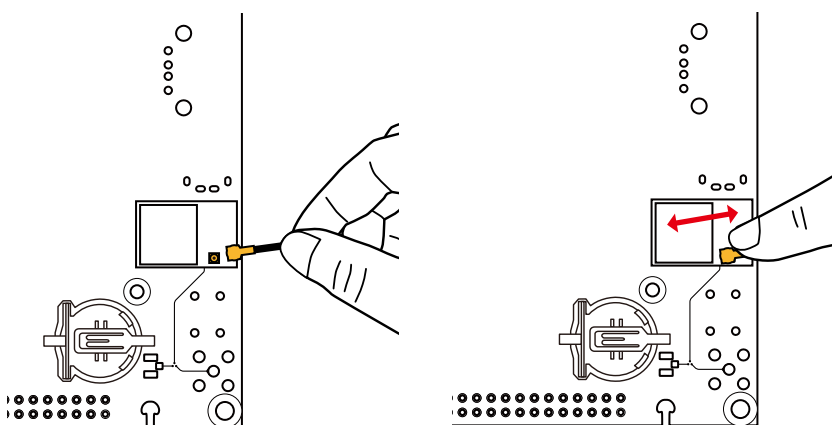
図 3.84 WLAN 基板アンテナの手による取り付け前の準備
