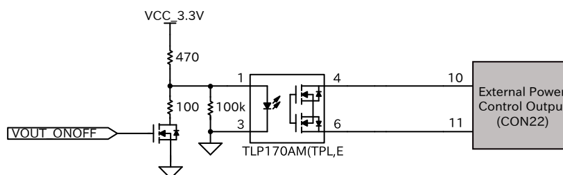
図 3.181 CON22 外部電源制御出力内部回路
