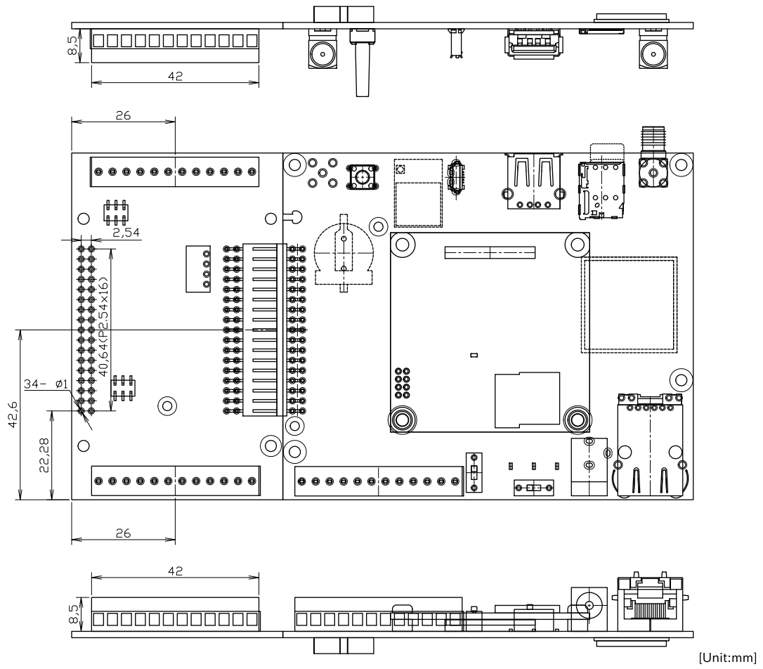
図 3.61 コネクタ、スイッチ、LED 位置(+Di8+Ai4 タイプ)
