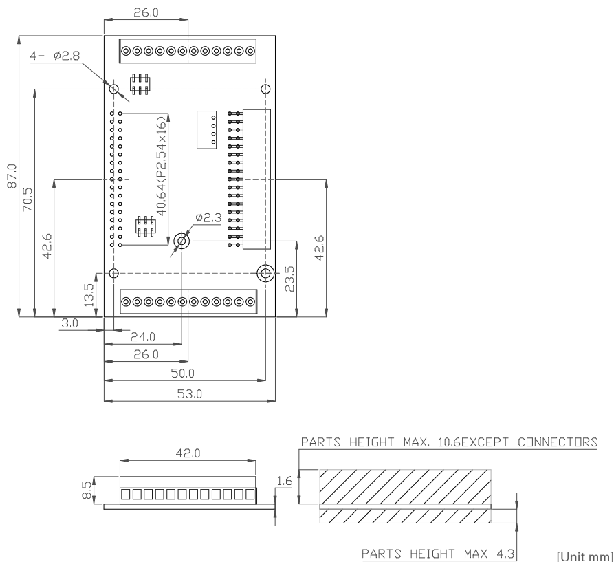
図 6.290 +Di8+Ai4 拡張基板基板形状図
