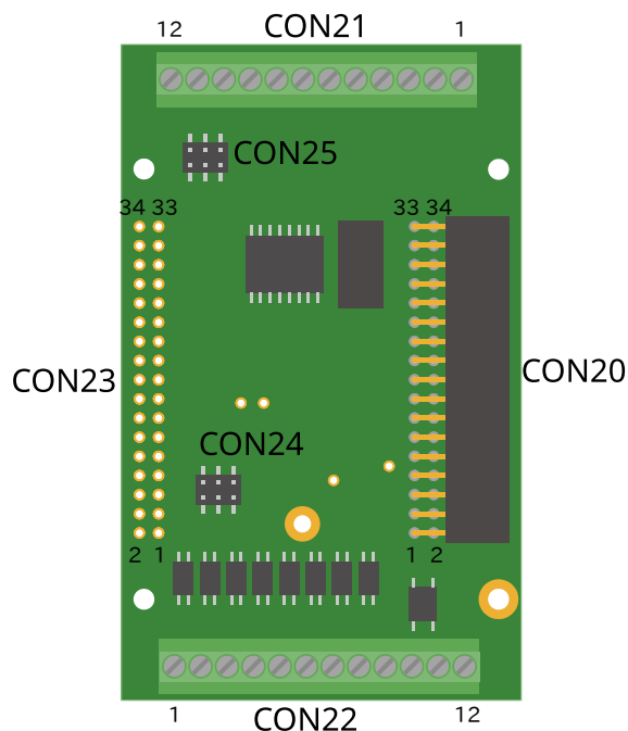
図 6.289 +Di8+Ai4 拡張基板のインターフェースレイアウト
