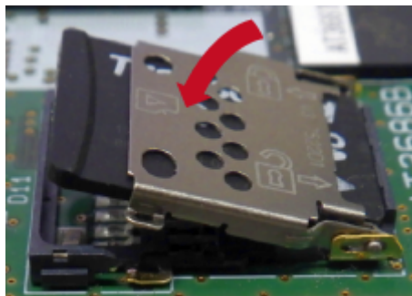
図 3.106 カバーを閉める
