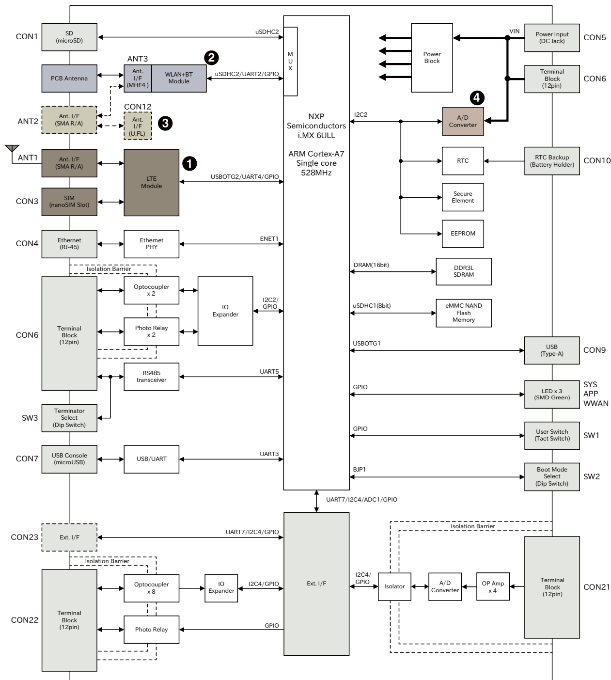
図 2.15 ブロック図 (+Di8+Ai4 タイプ)
