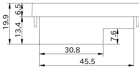
図 6.285 形状図 カバーパーツ B (アンテナ穴無し)
