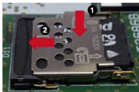
図 3.107 カバーをロックする
