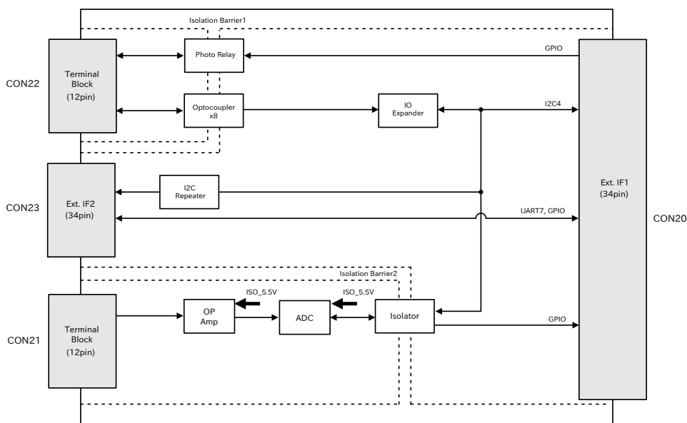
図 6.288 +Di8+Ai4 拡張基板のブロック図
