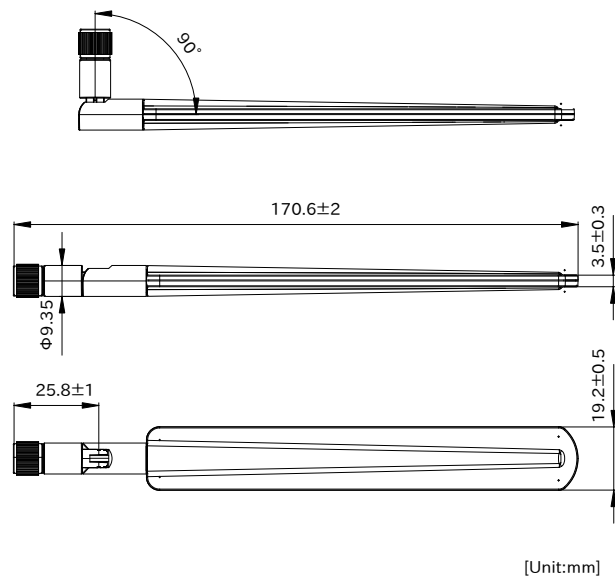
図 3.67 LTE アンテナ形状図
