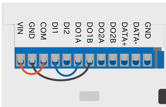
図 3.134 接点入力と接点出力をループバックする接続
