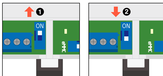
図 3.124 スイッチの状態と終端抵抗の ON/OFF
