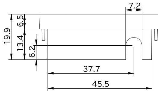
図 6.282 形状図 カバーパーツ A (アンテナ穴有り)
