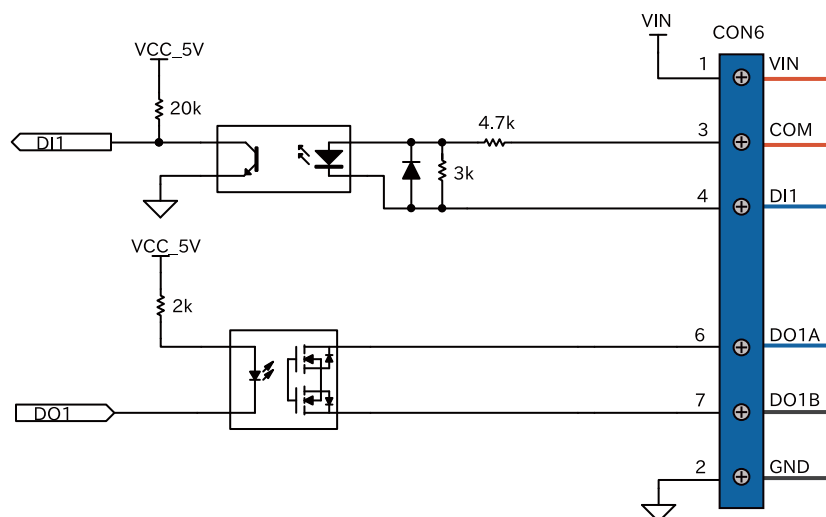
図 3.135 接点入力と接点出力をループバックする際の内部回路
