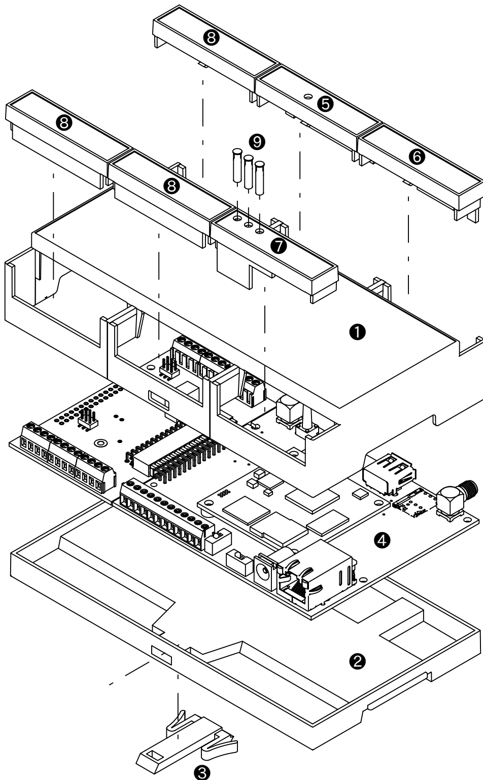
図 3.71 ケースモデル展開図 (+Di8+Ai4 タイプ)
