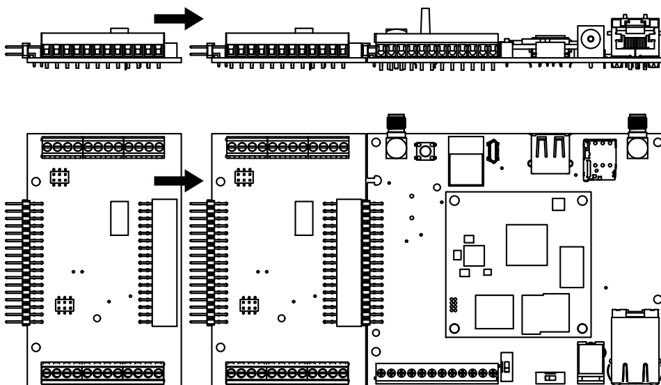
図 6.292 +Di8+Ai4 拡張基板の組付け方法
