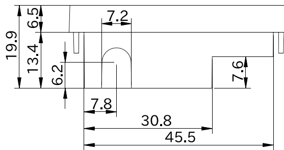
図 6.284 形状図 カバーパーツ B (アンテナ穴有り)
