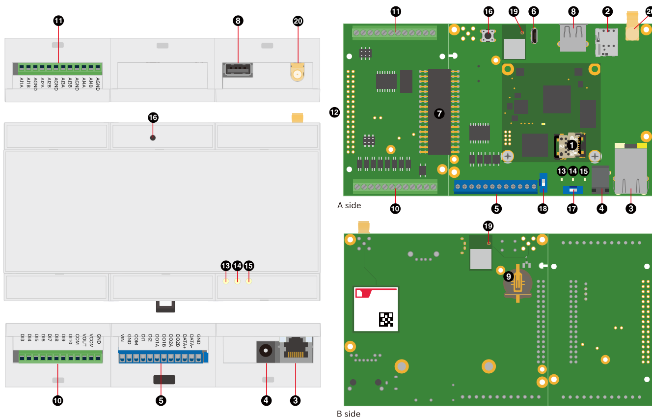
図 2.13 Armadillo-IoT ゲートウェイ A6E インターフェースレイアウト (+Di8+Ai4 タイプ)
