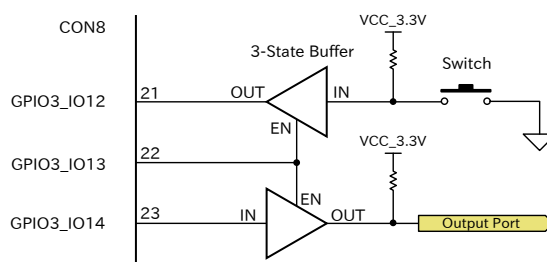
図 3.47 3-State バッファを使用した回路例
