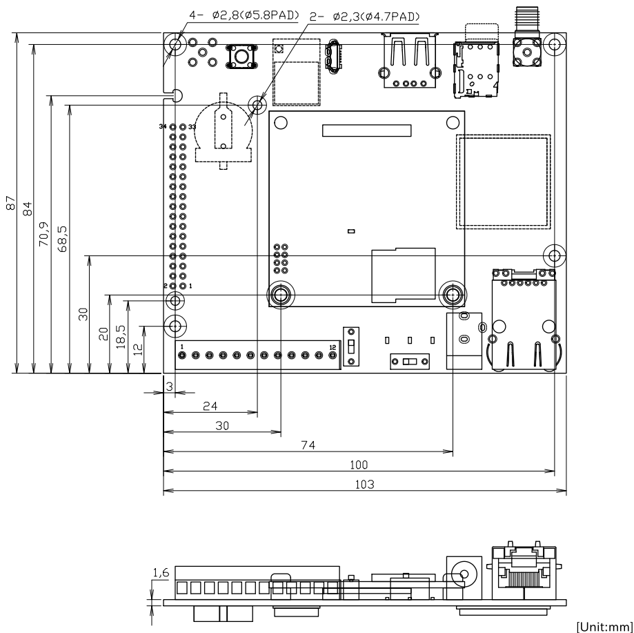
図 3.57 基板形状および固定穴寸法(スタンダードタイプ)
