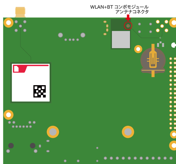
図 3.79 WLAN+BT コンボモジュールのアンテナコネクタの位置 (Cat.1 bis+WLAN モデル)
