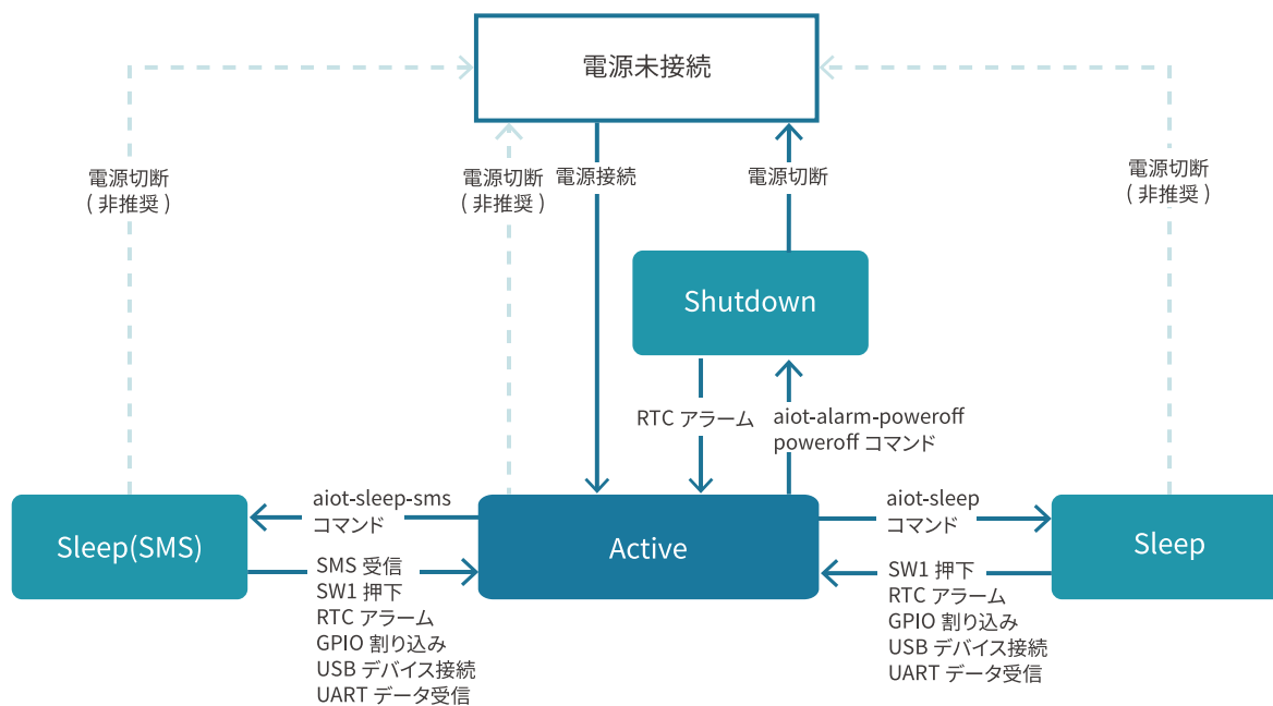
図 3.187 状態遷移図
