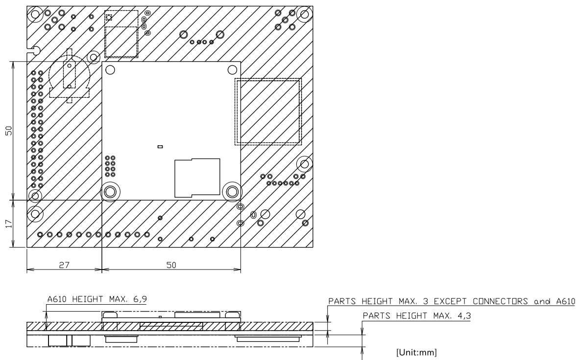
図 3.59 部品高さ(スタンダードタイプ)
