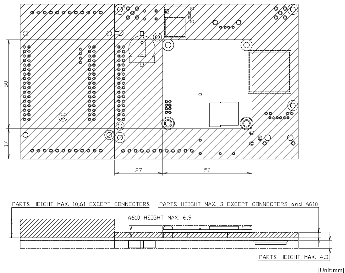
図 3.62 部品高さ(+Di8+Ai4 タイプ)
