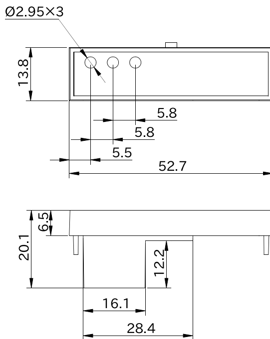
図 6.286 形状図 カバーパーツ C
