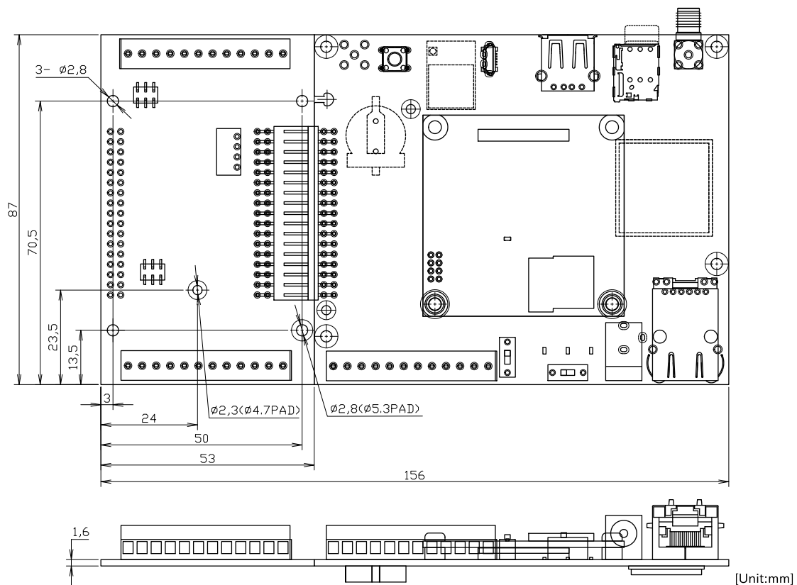
図 3.60 基板形状および固定穴寸法(+Di8+Ai4 タイプ)
