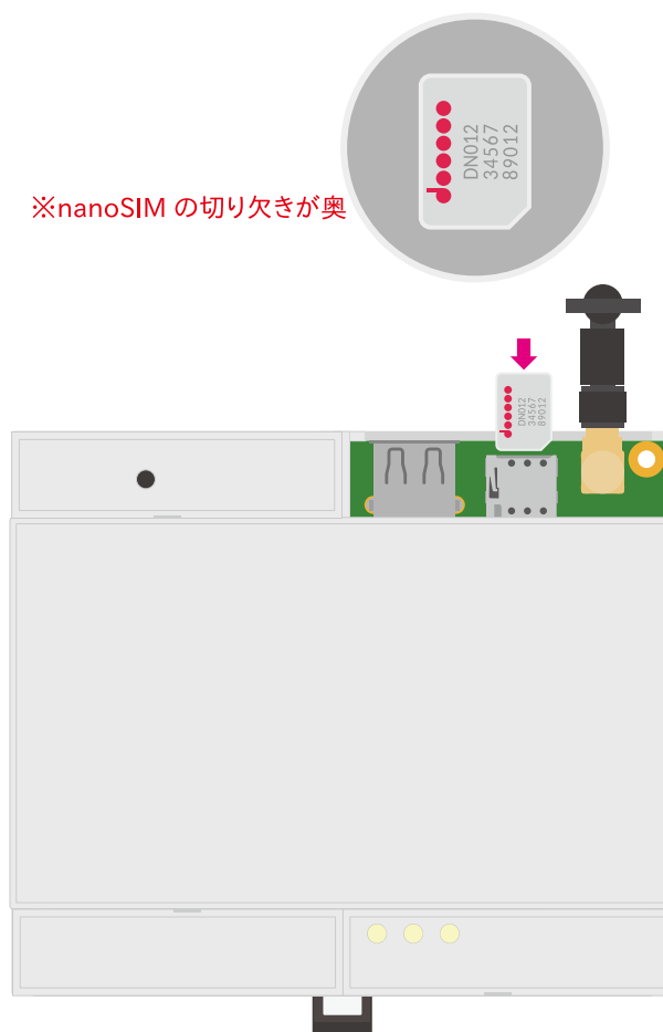
図 3.97 nanoSIM カードの接続例
