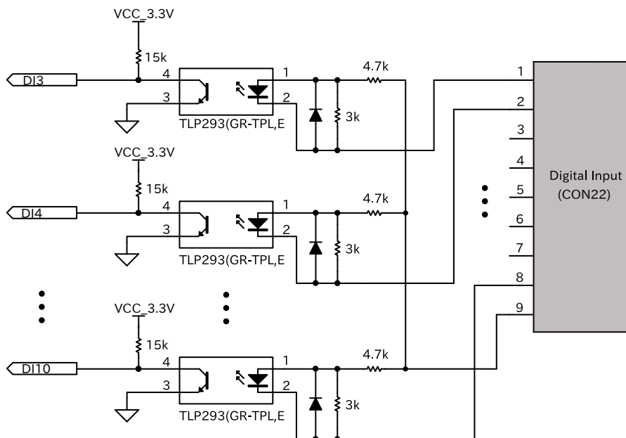
図 3.132 接点入力(CON22) 内部回路
