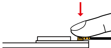
図 3.85 WLAN 基板アンテナの手による取り付け
