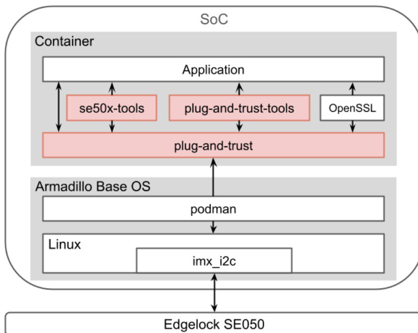
図 6.271 Plug & Trust Middleware の周辺のソフトウェアスタック
