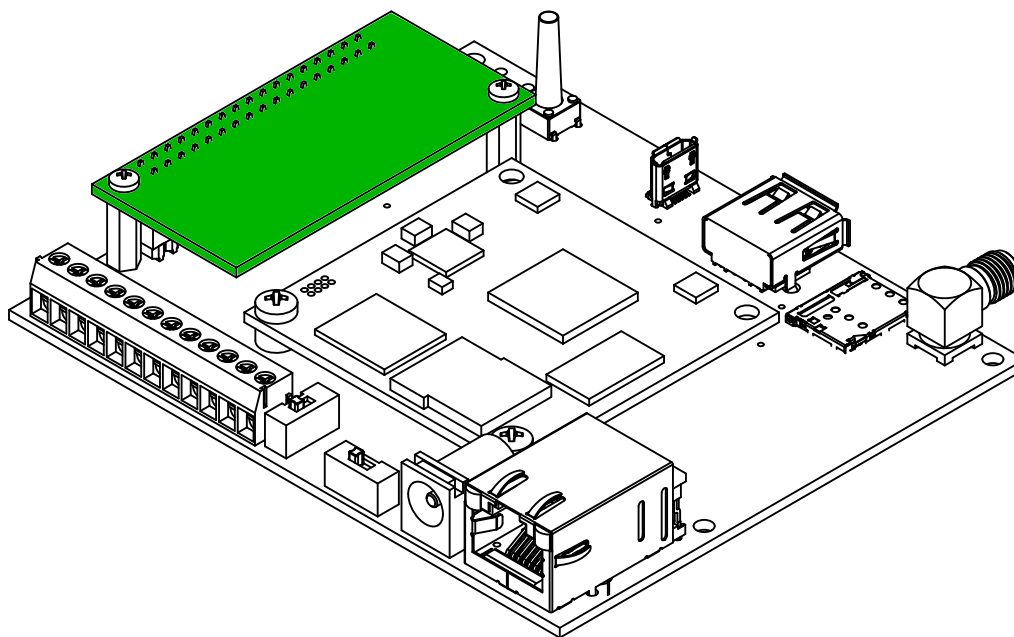
図 3.49 垂直方向に拡張基板を配置した場合の接続例
