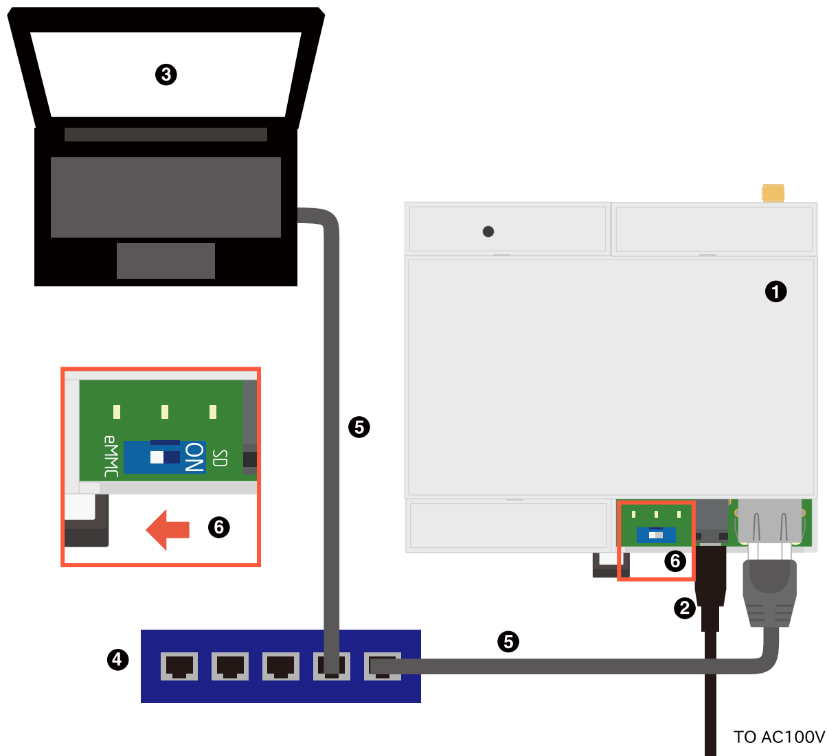
図 3.17 ABOS にアクセスするための接続
