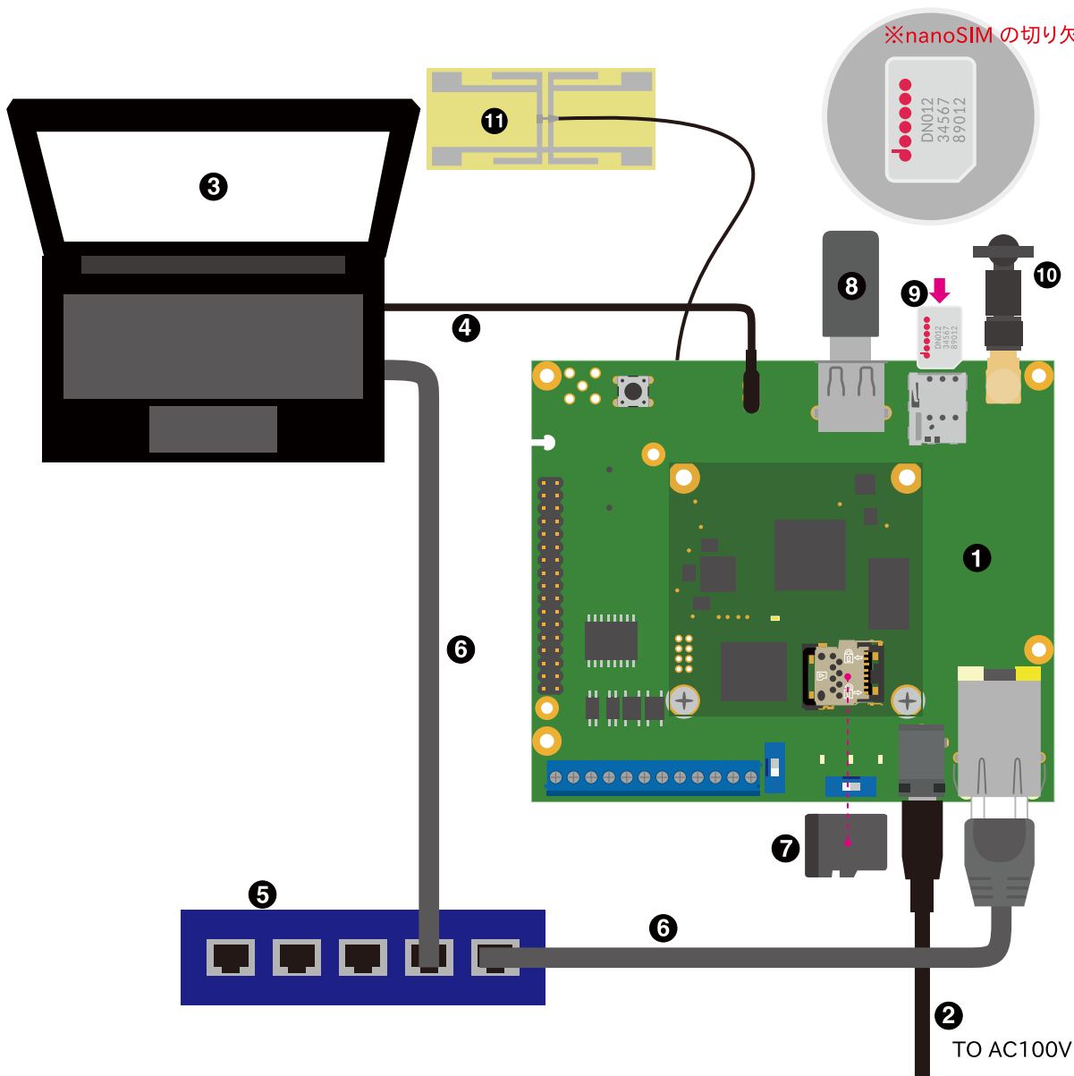
図 3.94 Armadillo-IoT ゲートウェイ A6E の接続例
