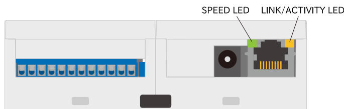
図 3.96 CON4 LAN LED
