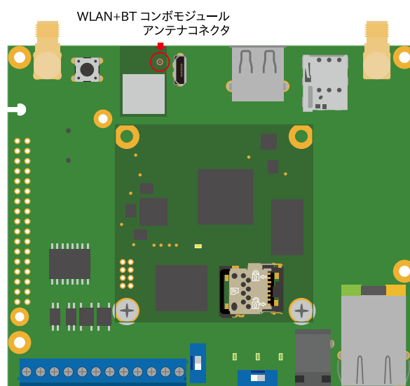
図 3.80 WLAN+BT コンボモジュールのアンテナコネクタの位置 (WLAN モデル)
