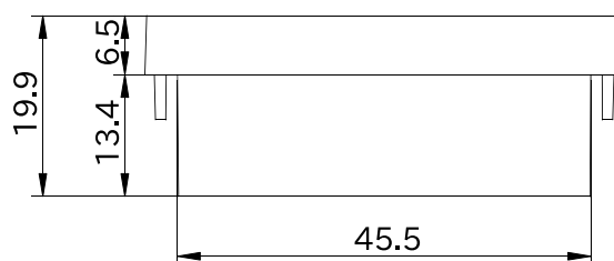
図 6.199 形状図 カバーパーツ A (アンテナ穴無し)
