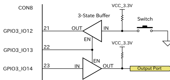
図 3.136 3-State バッファを使用した回路例
