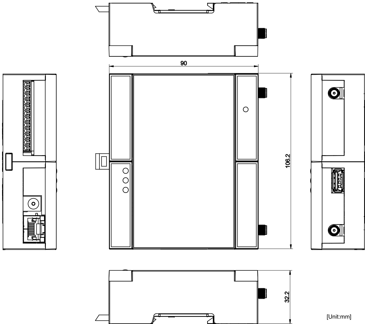
図 3.54 筐体形状
