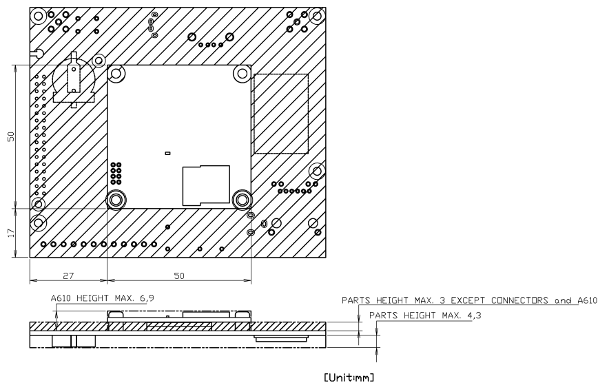
図 3.57 部品高さ
