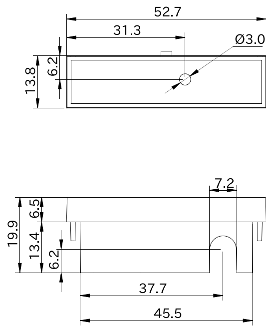
図 6.258 形状図 カバーパーツ A (アンテナ穴有り)
