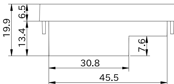
図 6.261 形状図 カバーパーツ B (アンテナ穴無し)
