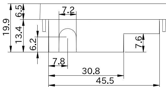
図 6.260 形状図 カバーパーツ B (アンテナ穴有り)
