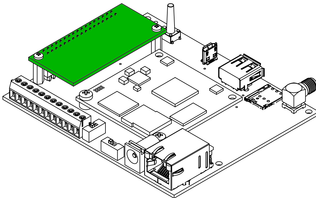
図 3.46 垂直方向に拡張基板を配置した場合の接続例
