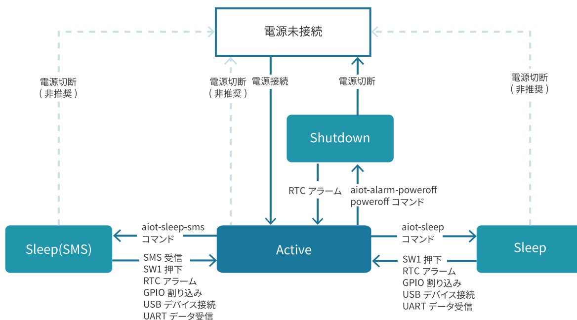
図 3.144 状態遷移図
