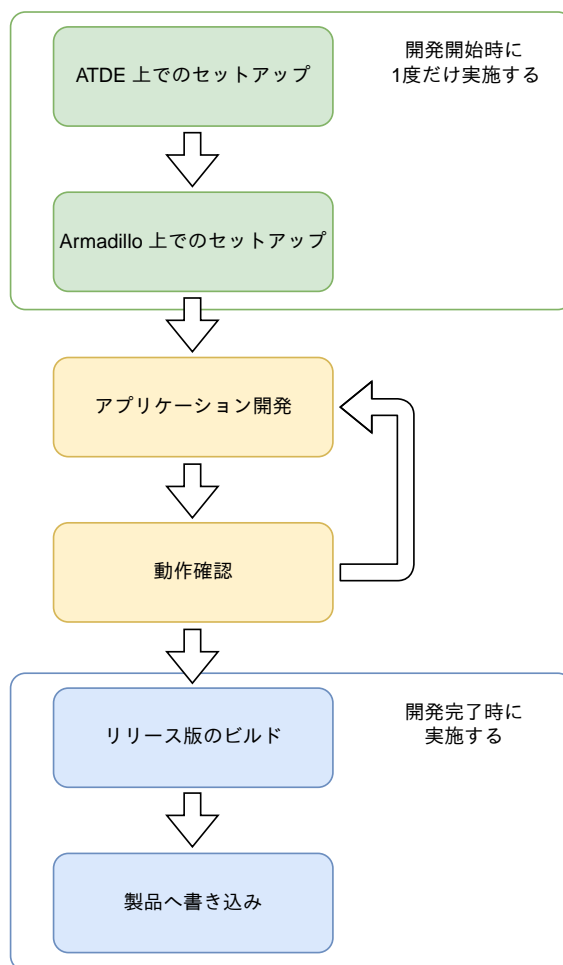
図 3.226 C 言語によるアプリケーション開発の流れ
