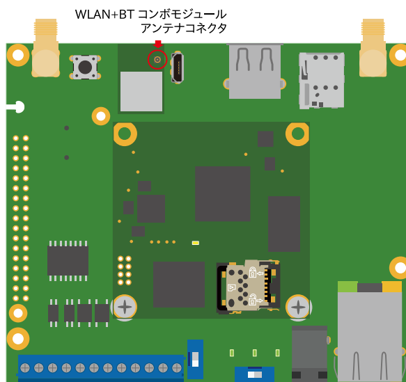
図 3.66 WLAN+BT コンボモジュールのアンテナコネクタの位置
