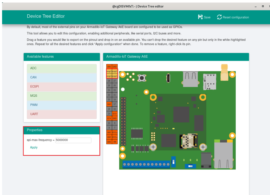
図 6.210 プロパティの設定
