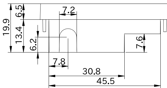
図 6.249 形状図 カバーパーツ B (アンテナ穴有り)
