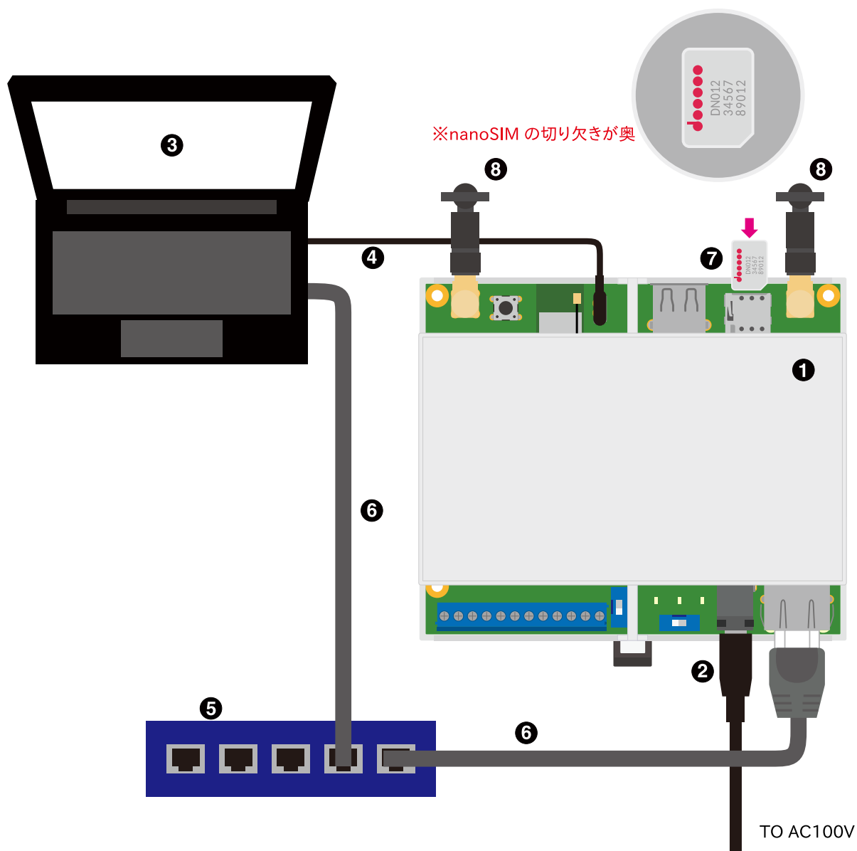
図 3.45 Armadillo-IoT ゲートウェイ A6E の接続例
