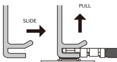
図 3.71 WLAN 基板アンテナの挿抜治具による取り外し
