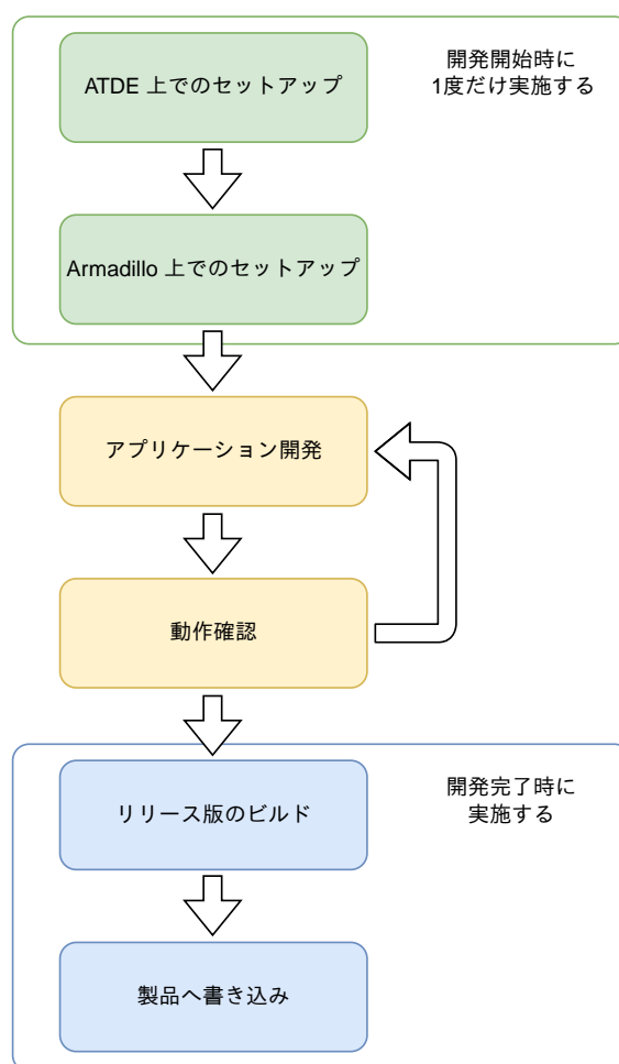
図 3.193 CUI アプリケーション開発の流れ
