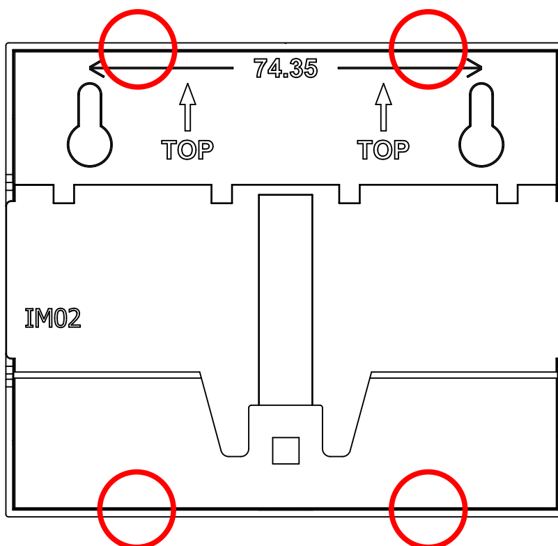
図 3.64 ケースボトムのツメ
