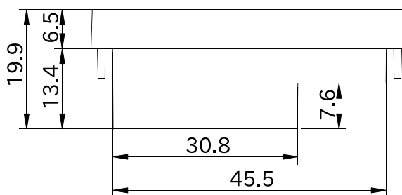
図 6.250 形状図 カバーパーツ B (アンテナ穴無し)
