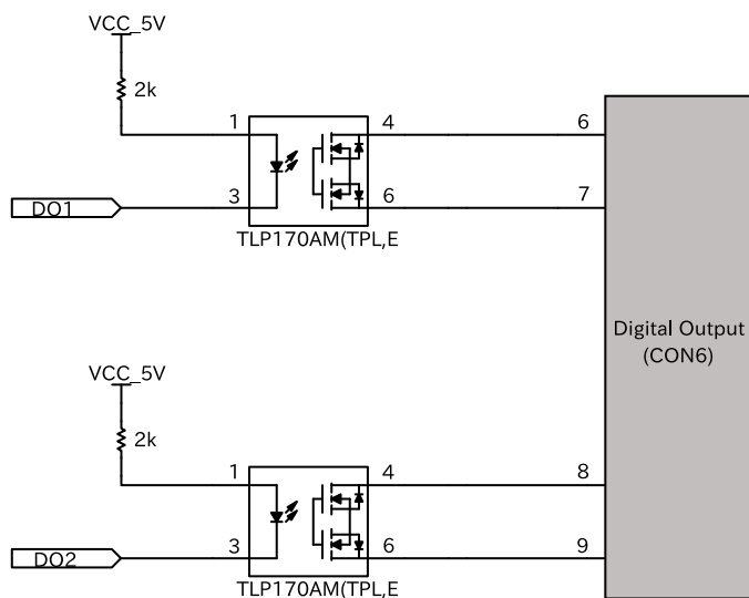
図 3.107 CON6 接点出力周辺回路
