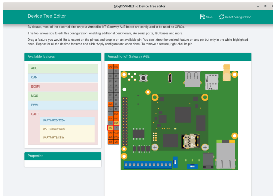
図 6.209 信号名の確認
