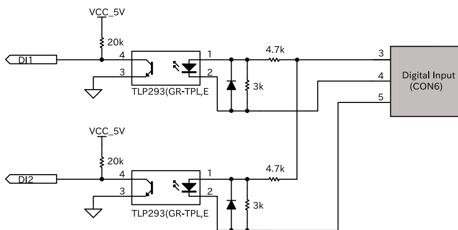
図 3.103 CON6 接点入力周辺回路
