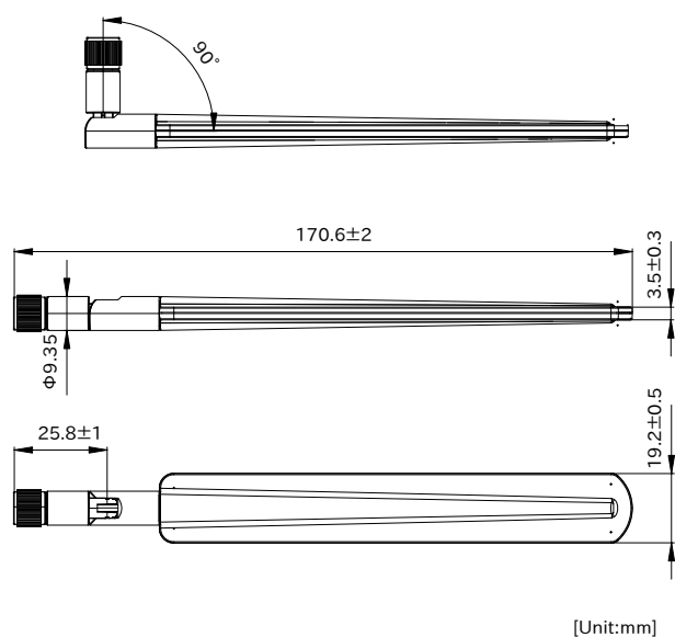
図 3.58 LTE アンテナ形状図
