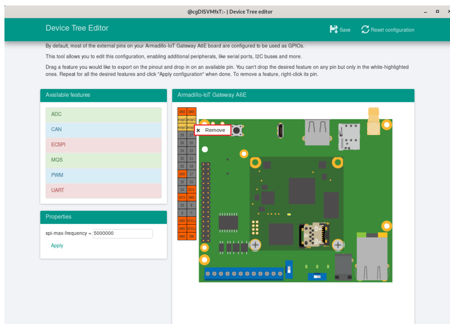
図 6.213 ECSPi1 の削除
