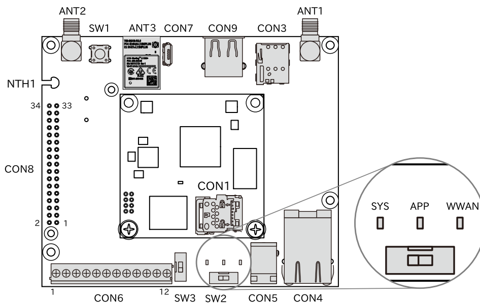
図 3.74 Armadillo-IoT ゲートウェイ A6E のインターフェース 表面
