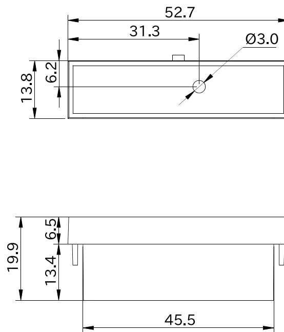
図 6.248 形状図 カバーパーツ A (アンテナ穴無し)
