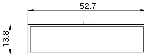
図 6.249 形状図 カバーパーツ B (アンテナ穴有り)
