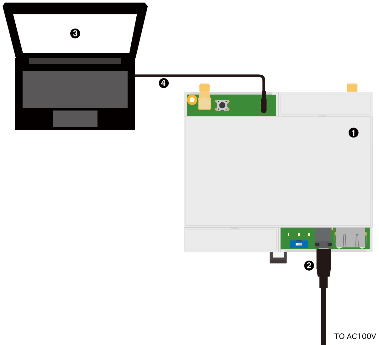
図 3.39 シリアルコンソールを使用する配線例
