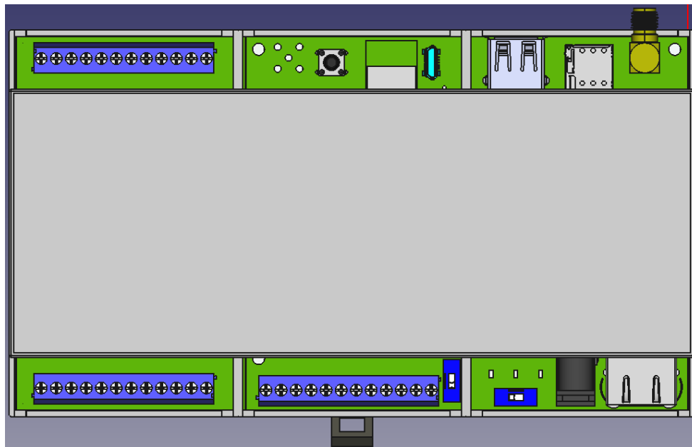
図 3.48 Armadillo-IoT ゲートウェイ A6E 標準ケースセットロング(9M) (OP-CASEA6E-PLA-20) 搭載例
