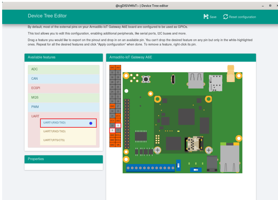
図 6.207 UART1(RXD/TXD) のドラッグ
