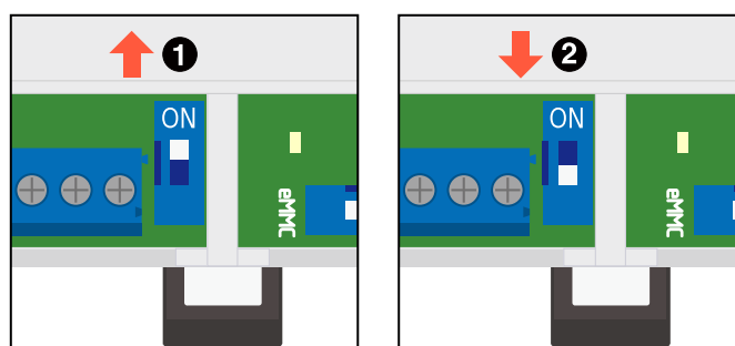
図 3.113 スイッチの状態と終端抵抗の ON/OFF
