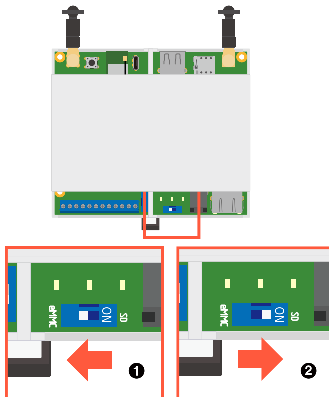
図 3.12 起動デバイス設定スイッチの操作
