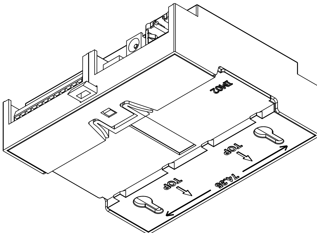
図 3.61 フック取り付け 2
