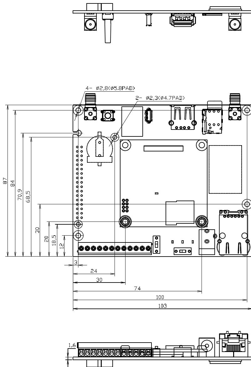
図 3.55 基板形状および固定穴寸法
