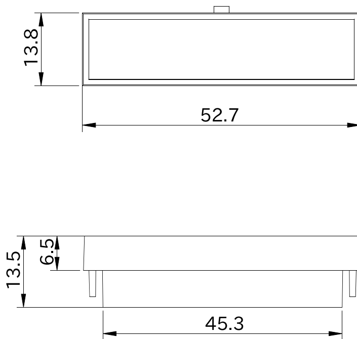
図 6.251 形状図 カバーパーツ C
