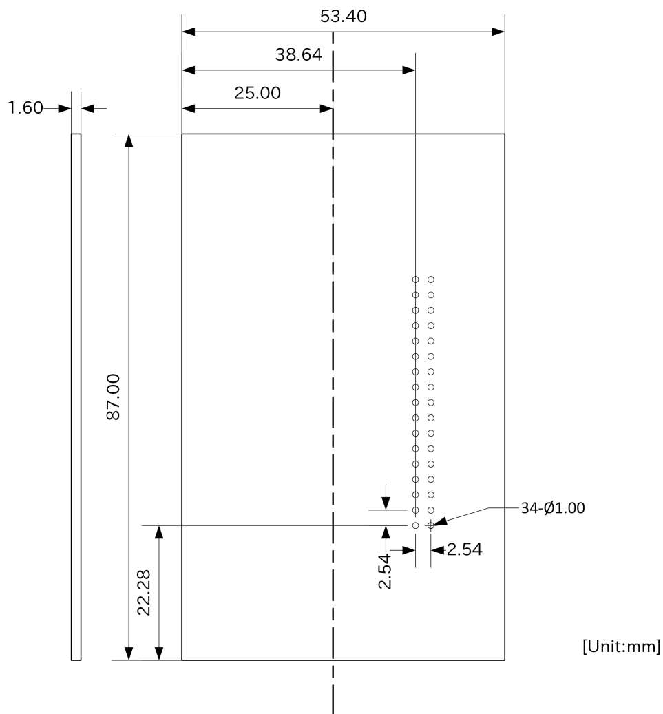
図 3.49 水平方向に拡張する場合の基板形状図
