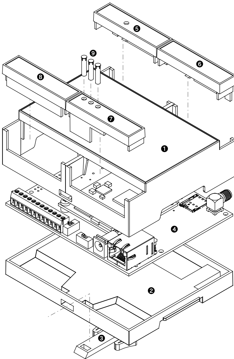
図 3.59 ケースモデル展開図
