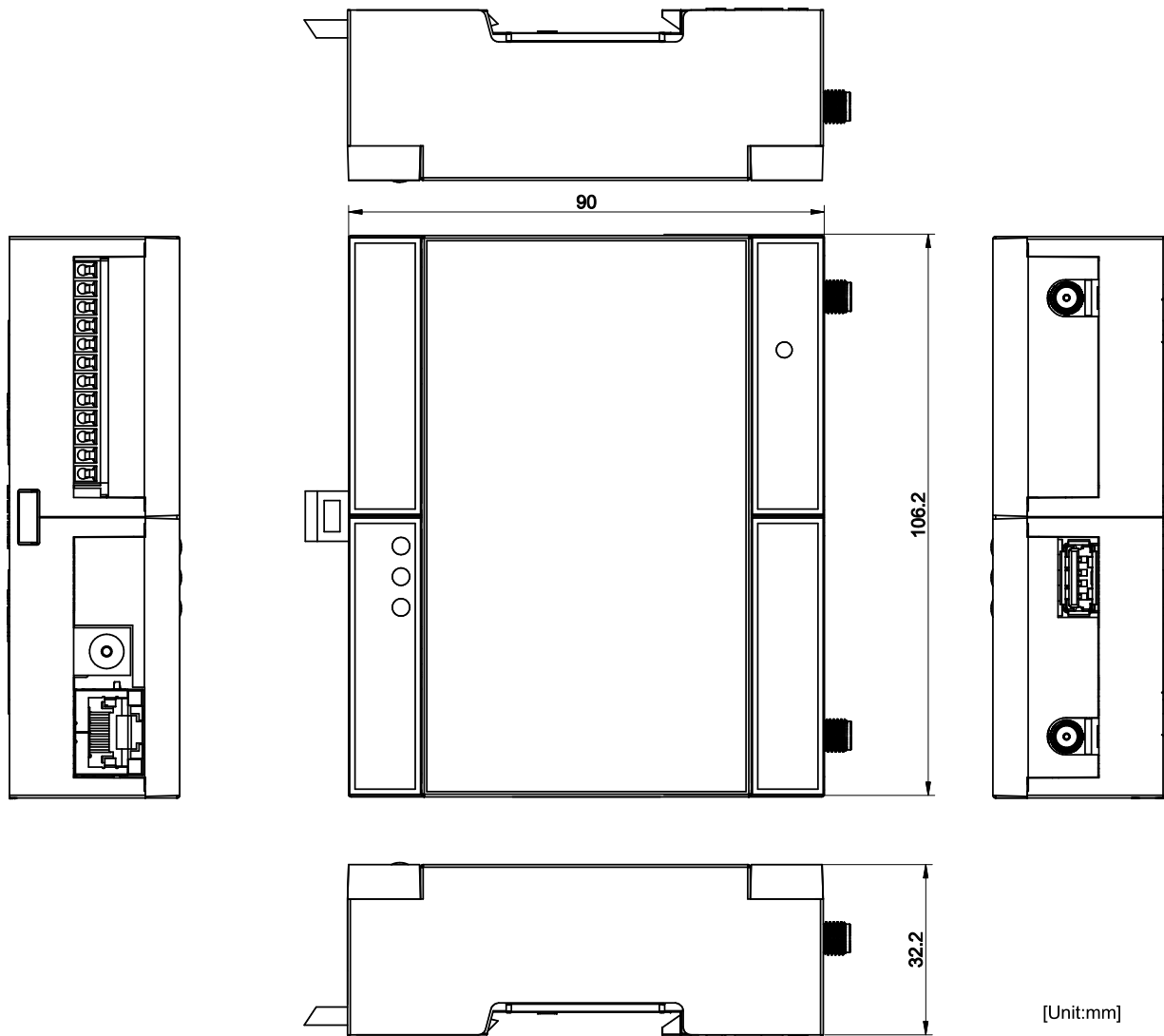
図 3.54 筐体形状
