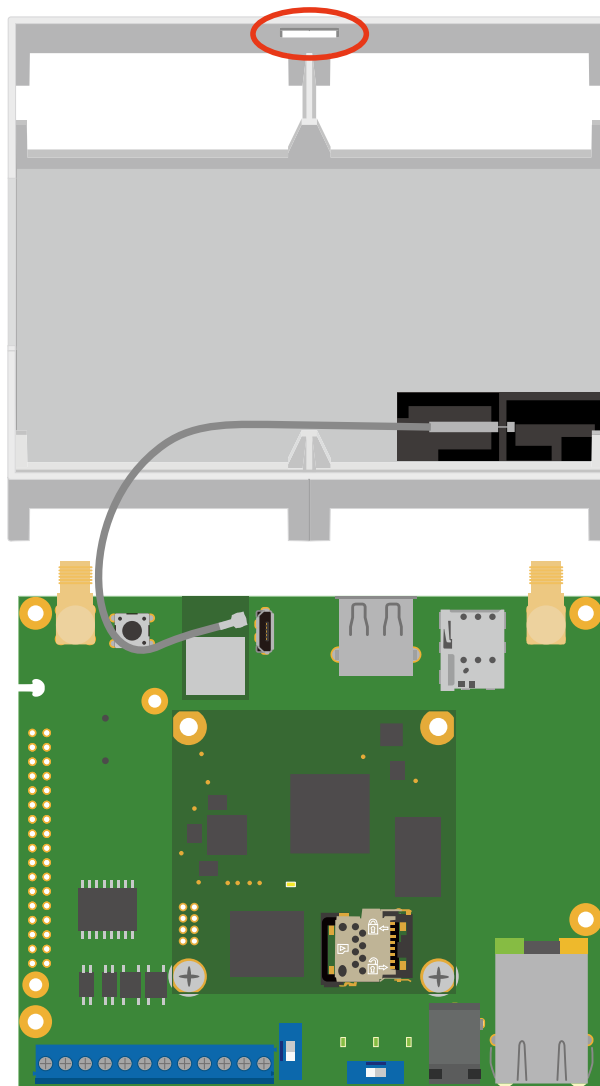
図 3.72 WLAN 基板アンテナの貼り付け位置
