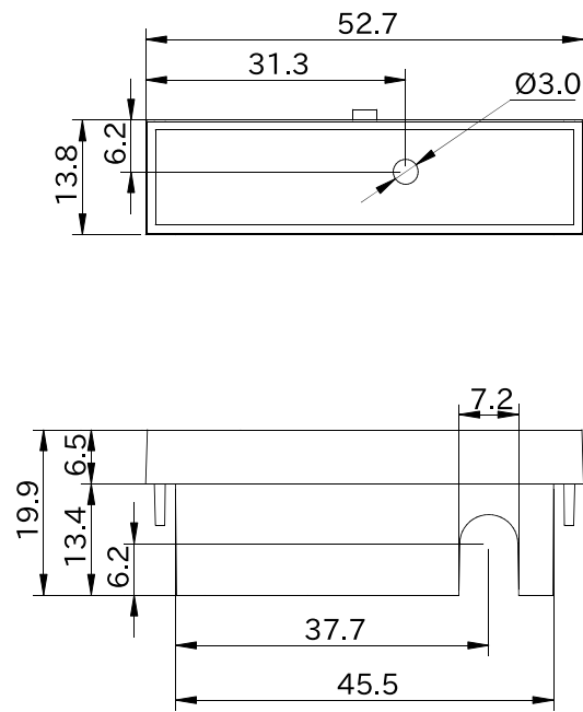
図 6.247 形状図 カバーパーツ A (アンテナ穴有り)
