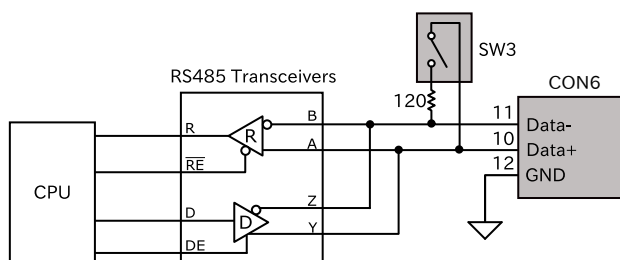
図 3.112 CON6 RS-485 トランシーバ周辺回路
