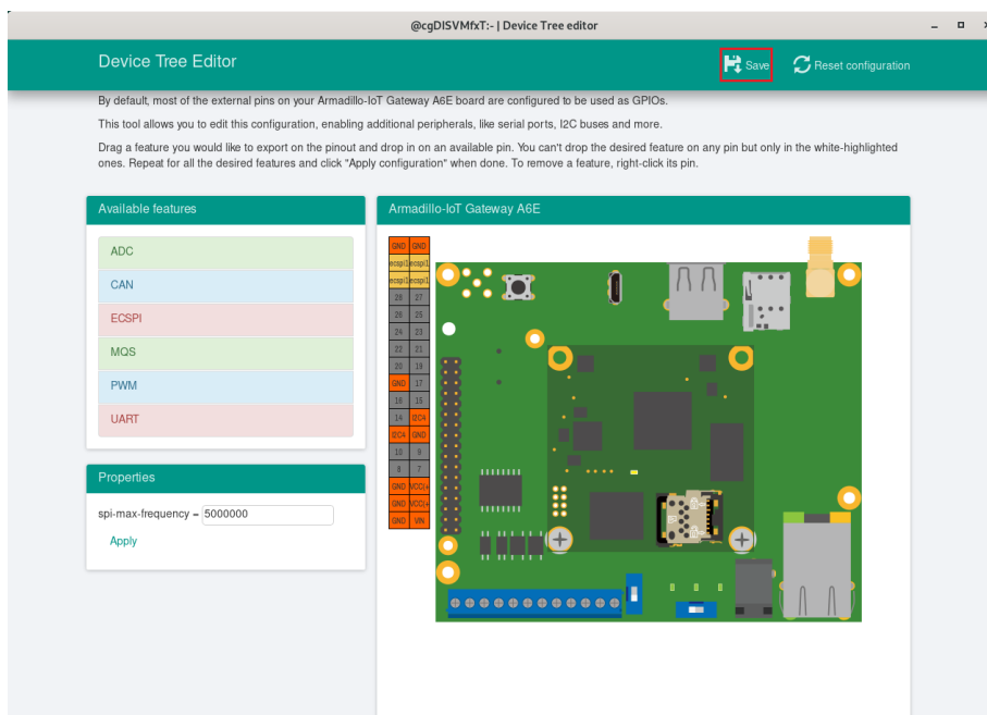
図 6.214 dtbo/desc ファイルの生成
