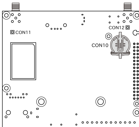
図 3.75 Armadillo-IoT ゲートウェイ A6E のインターフェース 裏面
