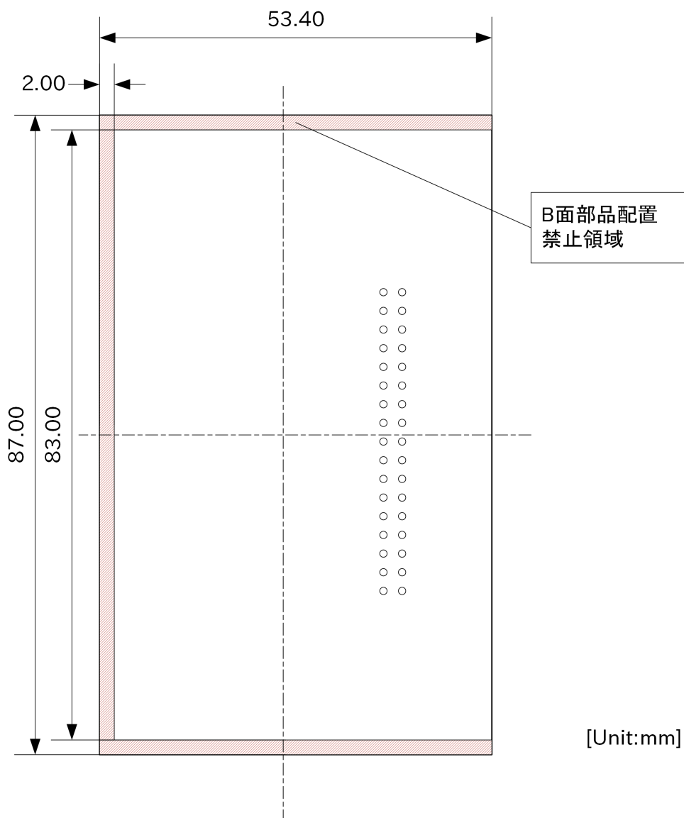
図 3.51 水平方向に拡張する場合の部品搭載制限(B 面側)
