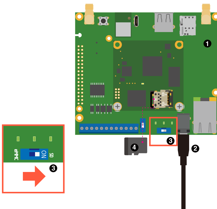
図 3.11 Armadillo-IoT ゲートウェイ A6E を初期化する接続
