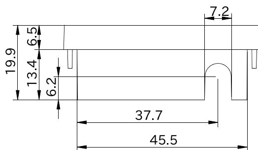
図 6.240 形状図 カバーパーツ A (アンテナ穴有り)
