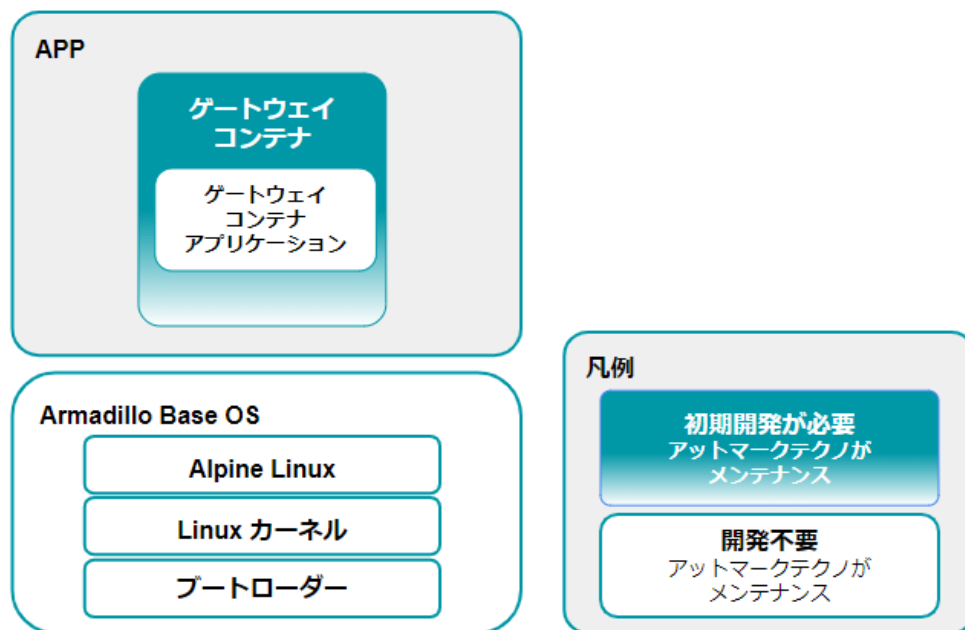
図 3.135 ゲートウェイコンテナ使用時、開発者が開発するもの、開発しなくていいもの
