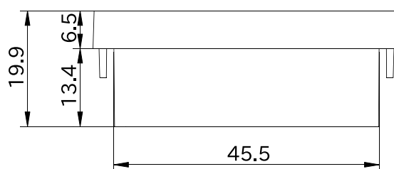
図 6.241 形状図 カバーパーツ A (アンテナ穴無し)
