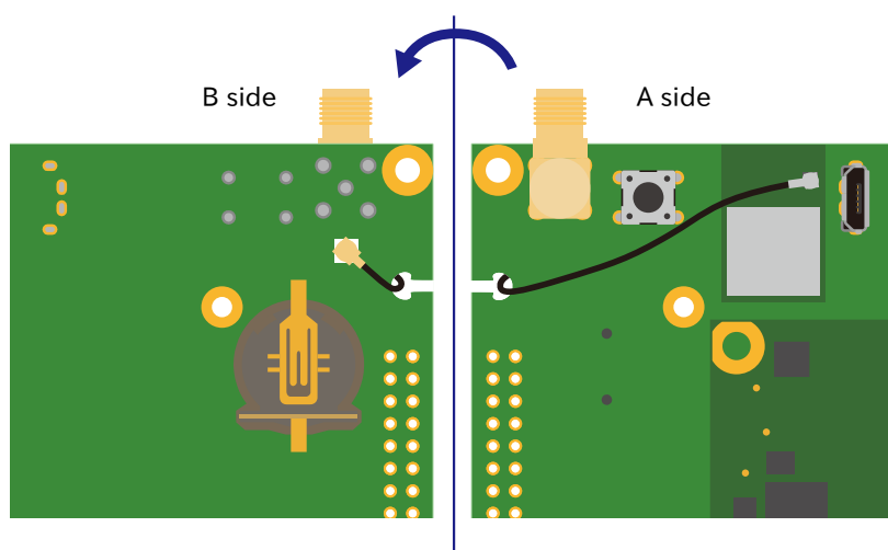
図 3.82 ANT2 カスタマイズ例：同軸ケーブル接続図
