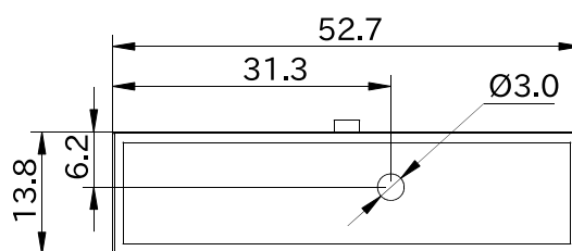
図 6.240 形状図 カバーパーツ A (アンテナ穴有り)
