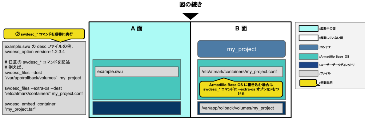
図 6.14 desc ファイルに記述した swudesc_* コマンドを実行
