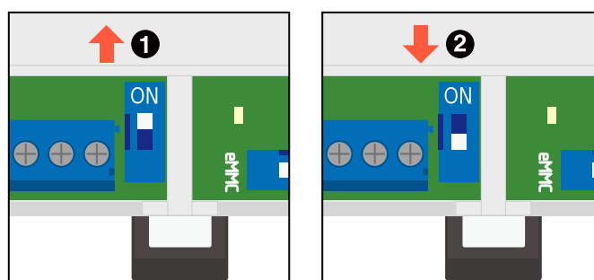
図 3.105 スイッチの状態と終端抵抗の ON/OFF
