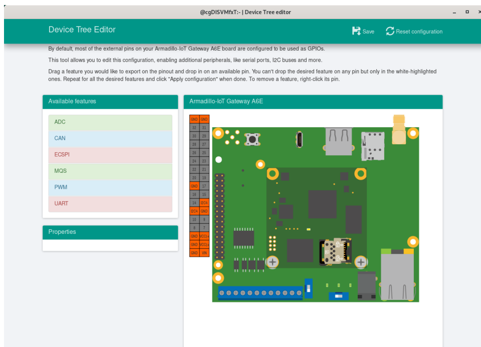
図 6.199 at-dtweb 起動画面
