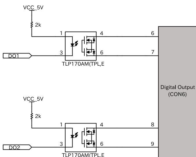
図 3.99 CON6 接点出力周辺回路
