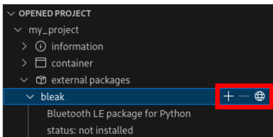
図 3.195 BLE パッケージをインストールする
