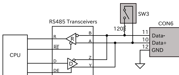
図 3.104 CON6 RS-485 トランシーバ周辺回路
