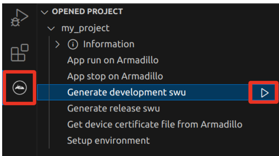
図 3.30 VSCode で SWU イメージの作成を行う
