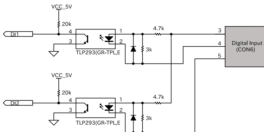
図 3.95 CON6 接点入力周辺回路
