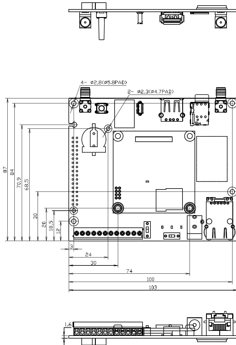
図 3.55 基板形状および固定穴寸法
