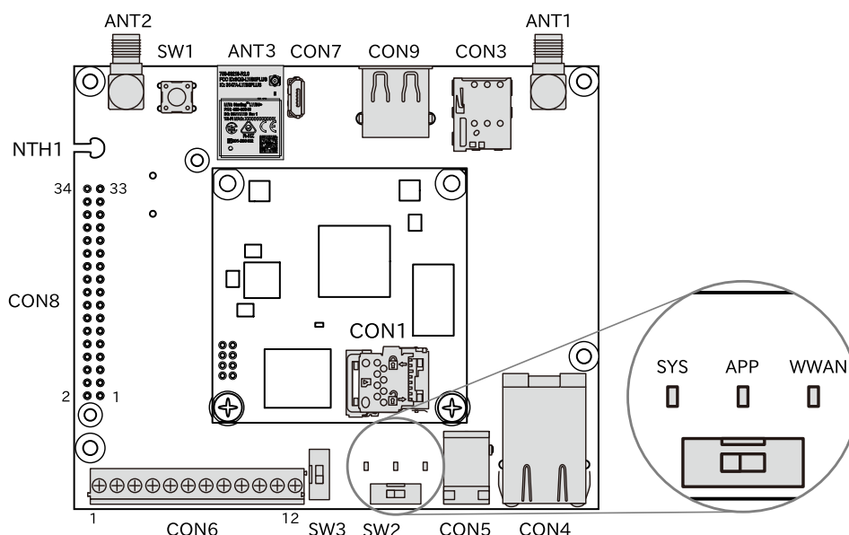
図 3.66 Armadillo-IoT ゲートウェイ A6E のインターフェース 表面
