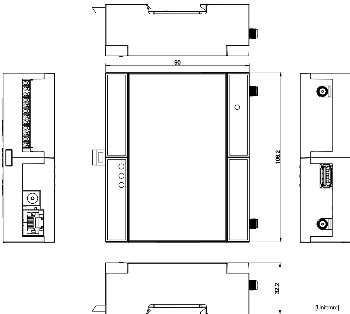
図 3.54 筐体形状
