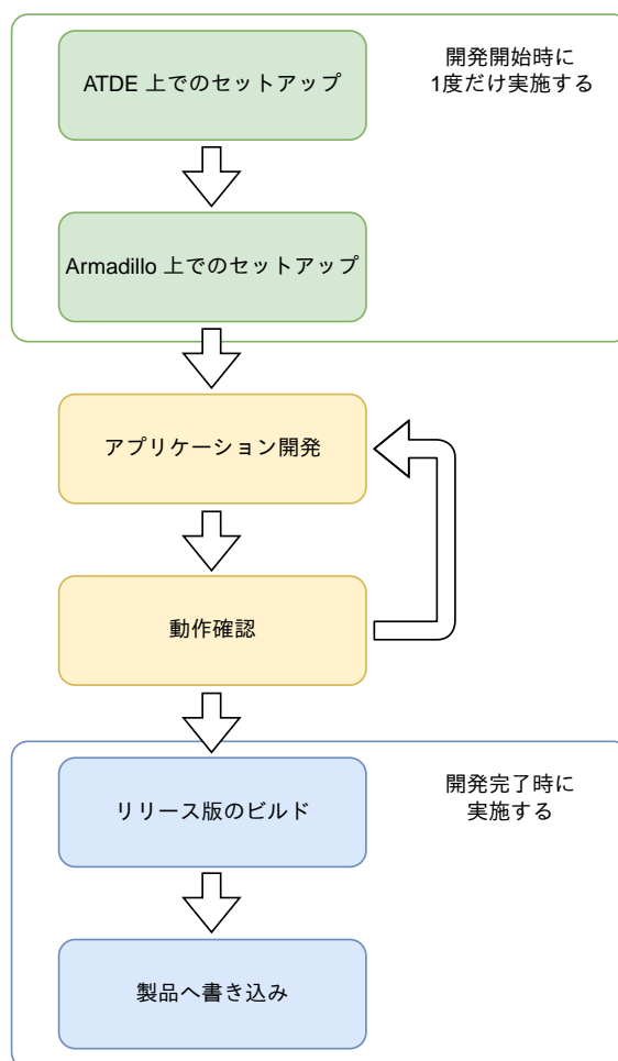
図 3.218 C 言語によるアプリケーション開発の流れ
