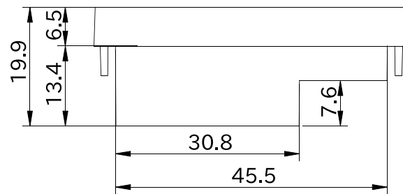
図 6.221 形状図 カバーパーツ B (アンテナ穴無し)
