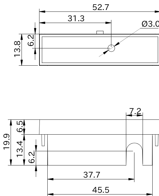
図 6.218 形状図 カバーパーツ A (アンテナ穴有り)
