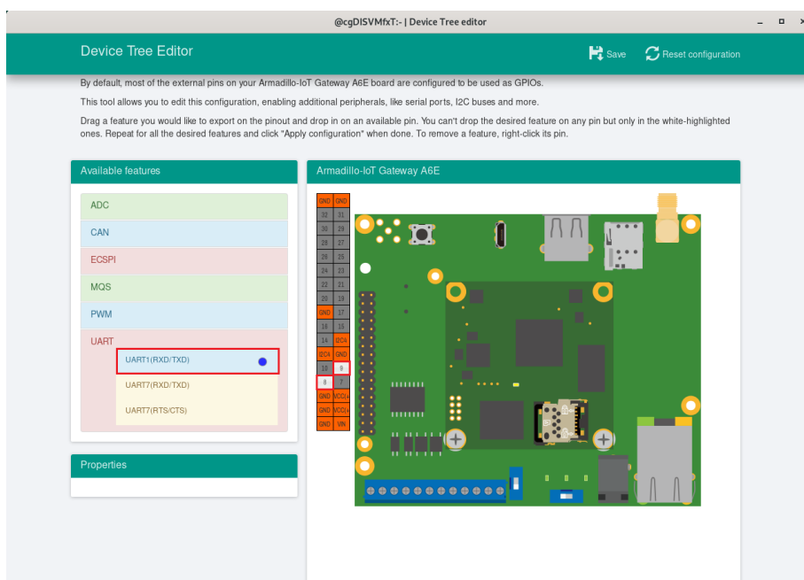
図 6.190 UART1 (RXD/TXD) のドラッグ
