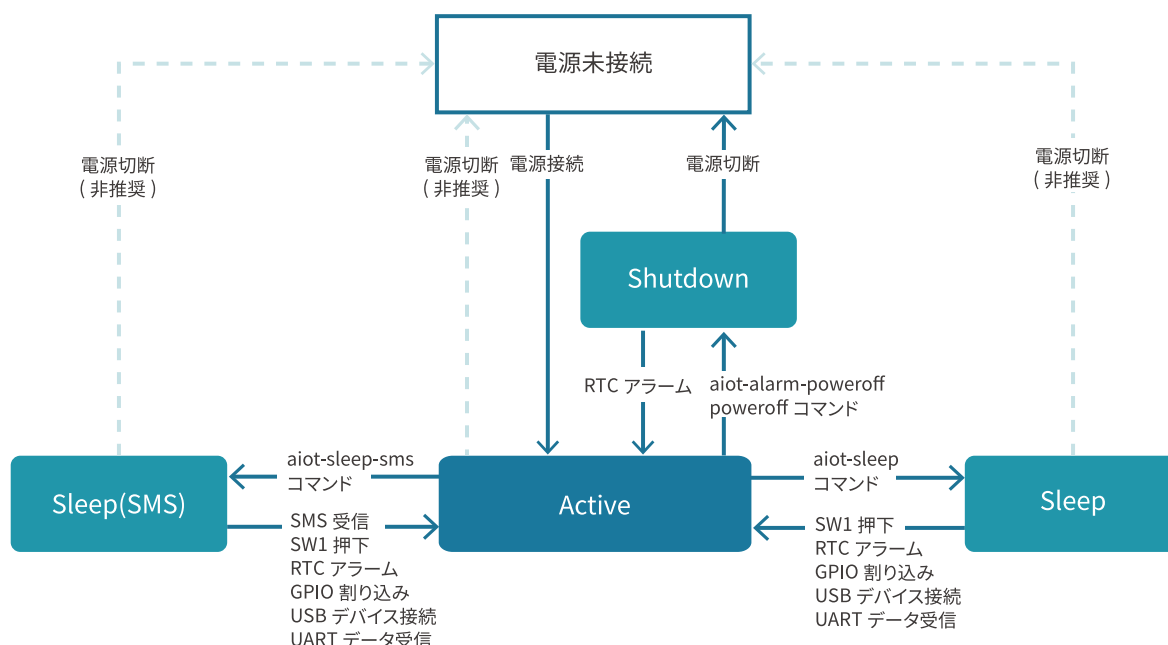
図 3.107 状態遷移図
