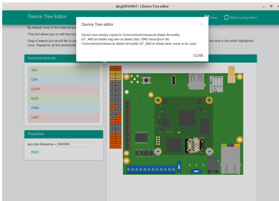
図 6.198 dtbo/desc の生成完了
