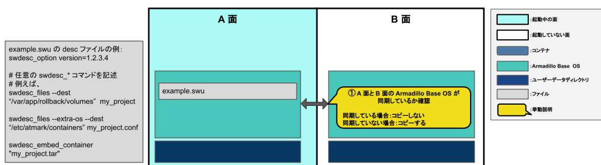
図 6.11 Armadillo Base OS を B 面にコピー
