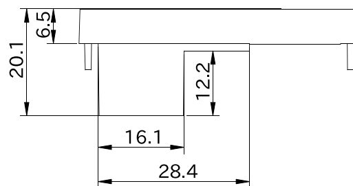
図 6.222 形状図 カバーパーツ C
