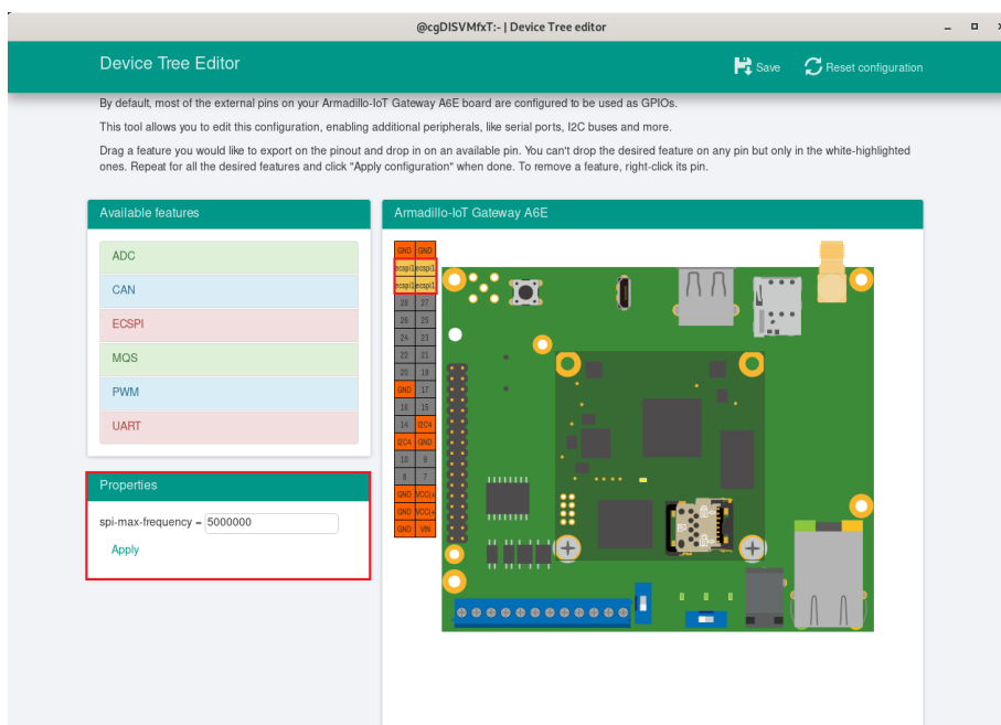
図 6.193 プロパティの設定
