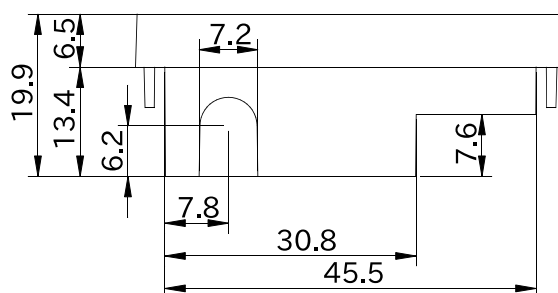
図 6.220 形状図 カバーパーツ B (アンテナ穴有り)
