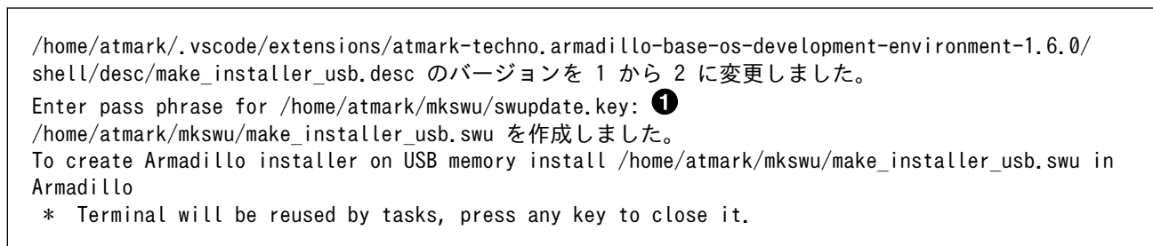
図 4.8 make-installer.swu 生成時のログ
