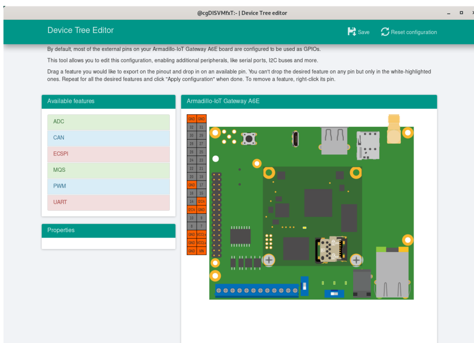
図 6.189 at-dtweb 起動画面
