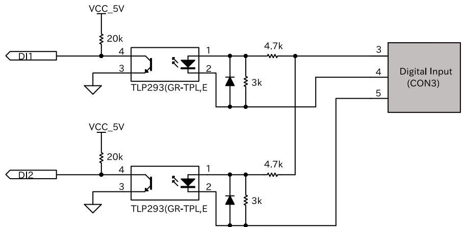
図 3.67 CON6 接点入力周辺回路
