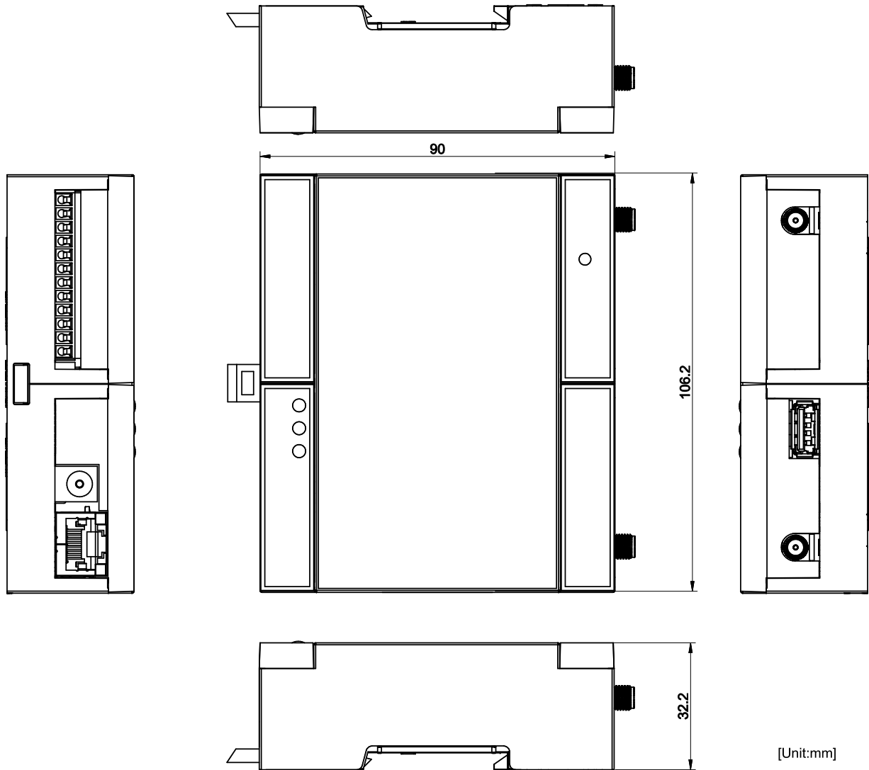
図 6.203 筐体形状
