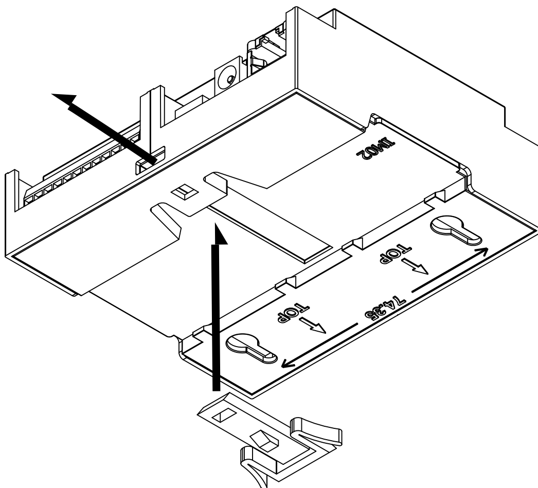
図 3.33 フック取り付け 1
