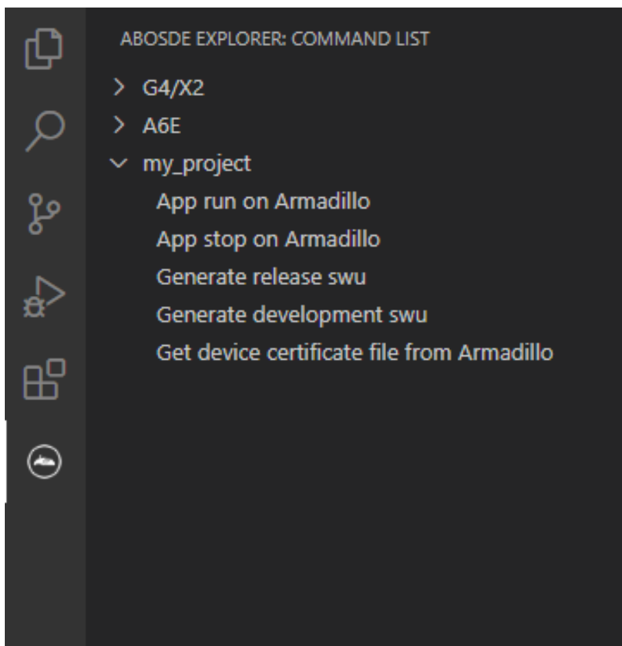
図 3.127 タスク一覧
