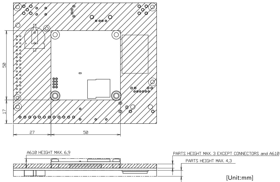
図 14.27 部品高さ
