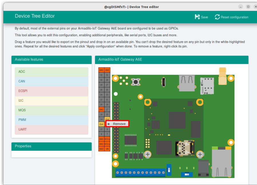
図 10.166 I2C4(SCL/SDA) の削除
