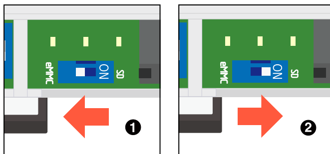
図 14.22 スイッチの状態と起動デバイス
