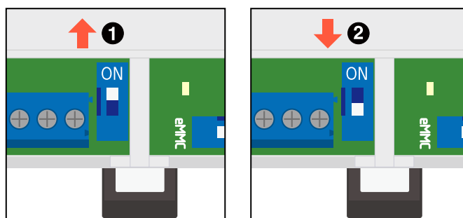
図 14.23 スイッチの状態と終端抵抗の ON/OFF
