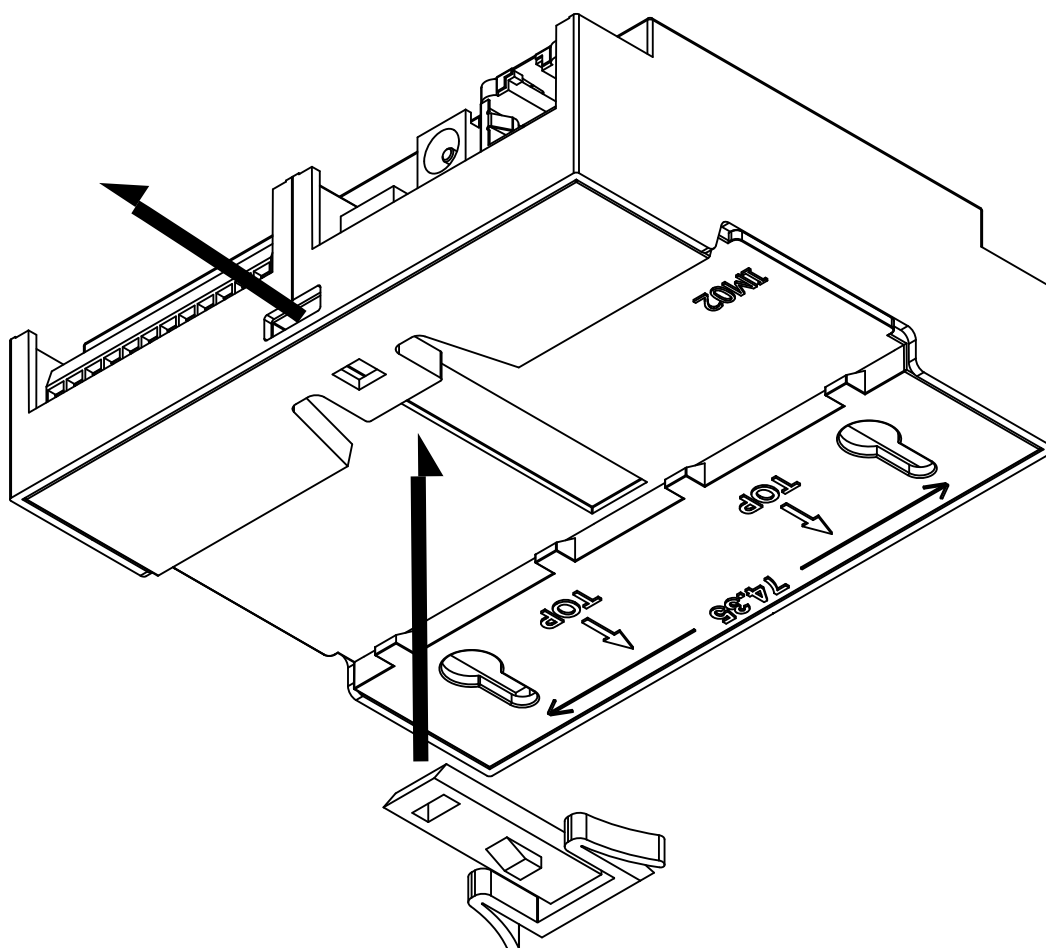
図 14.29 フック取り付け 1
