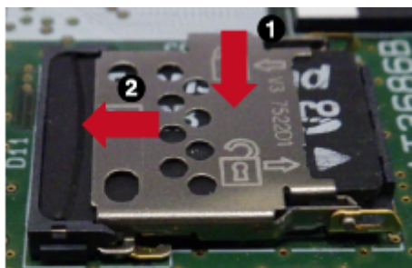
図 3.19 カバーをロックする
