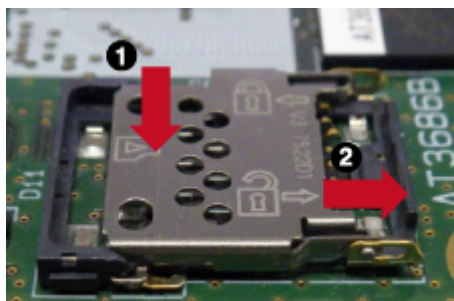
図 3.14 カバーのロックを解除する
