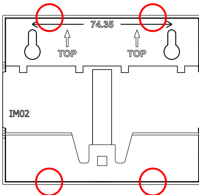
図 3.12 ケースボトムのツメ
