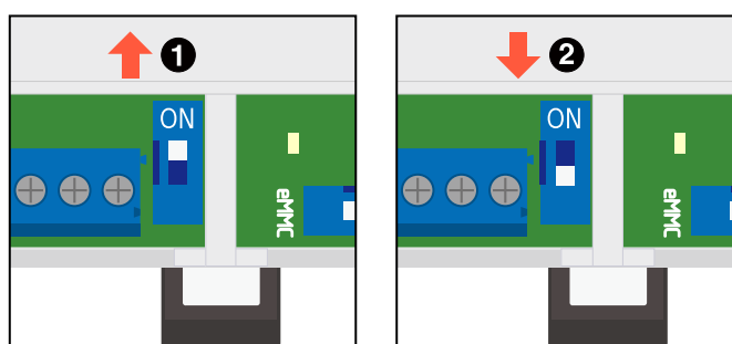
図 4.30 スwitchの状態と終端抵抗の ON/OFF
