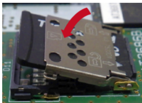
図 3.18 カバーを閉める
