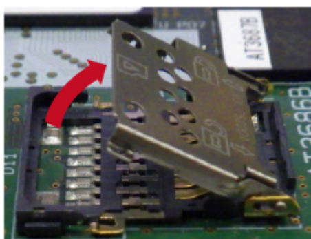
図 3.15 カバーを開ける
