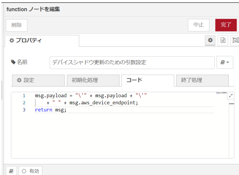
図 4.86 [デバイスシャドウ更新のための引数設定] ノードのプロパティ内容
