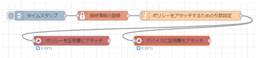
図 4.78 デバイスにポリシーをアタッチするフロー
