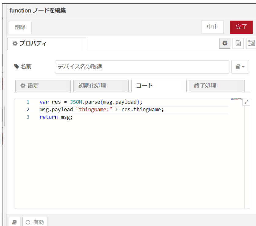
図 4.60 [デバイス名の取得] ノードのプロパティ内容
