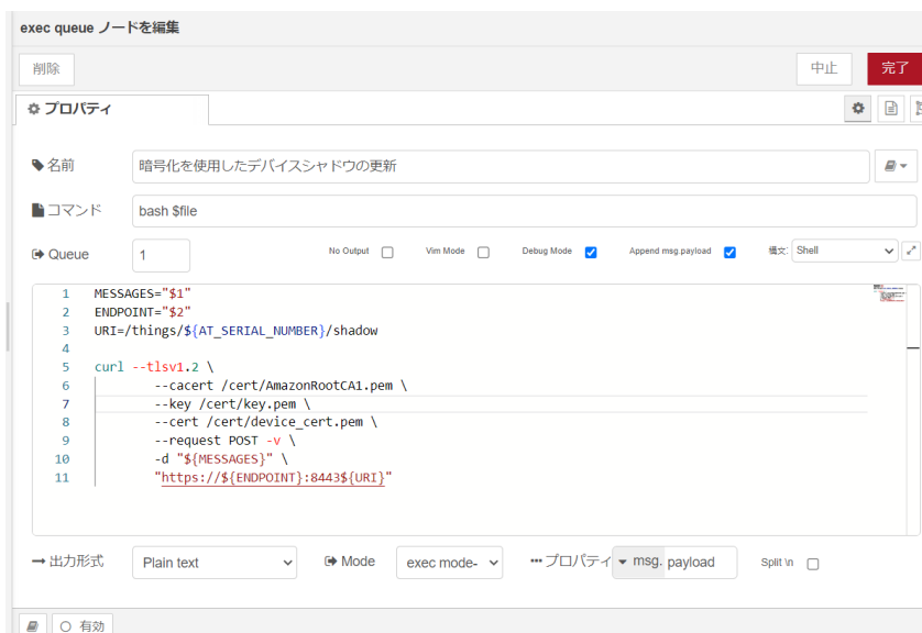
図 4.87 [暗号化を使用したデバイスシャドウの更新] ノードのプロパティ内容
