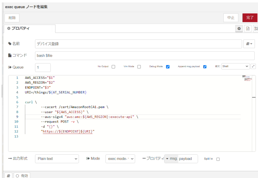
図 4.59 [exec queue] ノードのプロパティ内容
