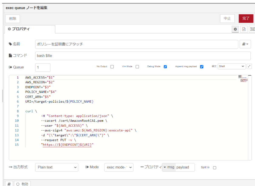
図 4.76 [ポリシーを証明書にアタッチ] ノードのプロパティ内容
