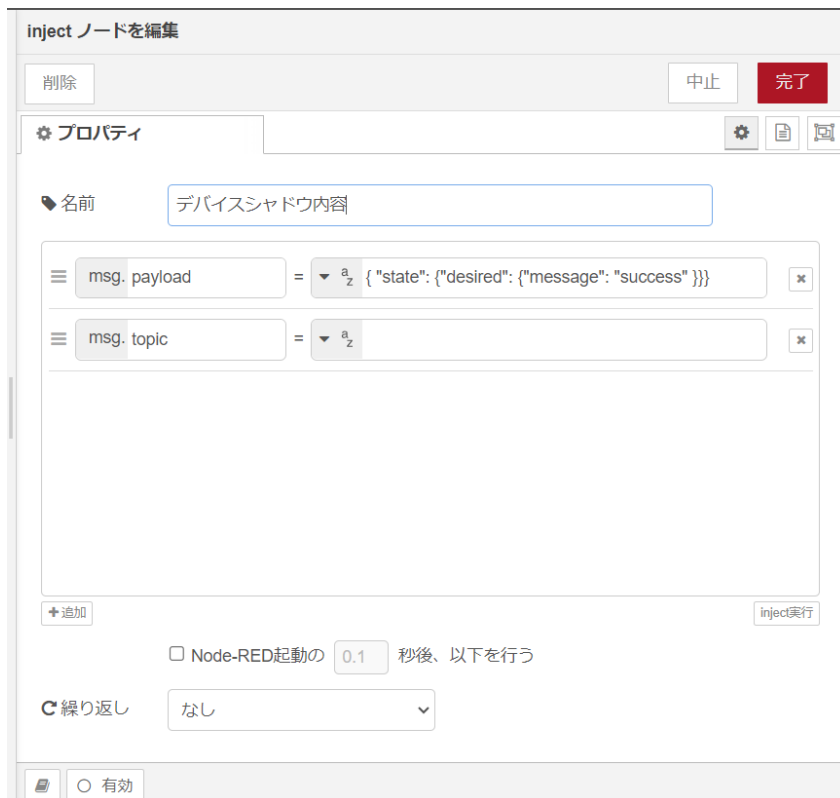
図 4.84 [デバイスシャドウ内容] ノードのプロパティ内容
