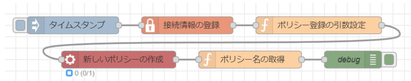
図 4.67 ポリシーを作成するフロー
