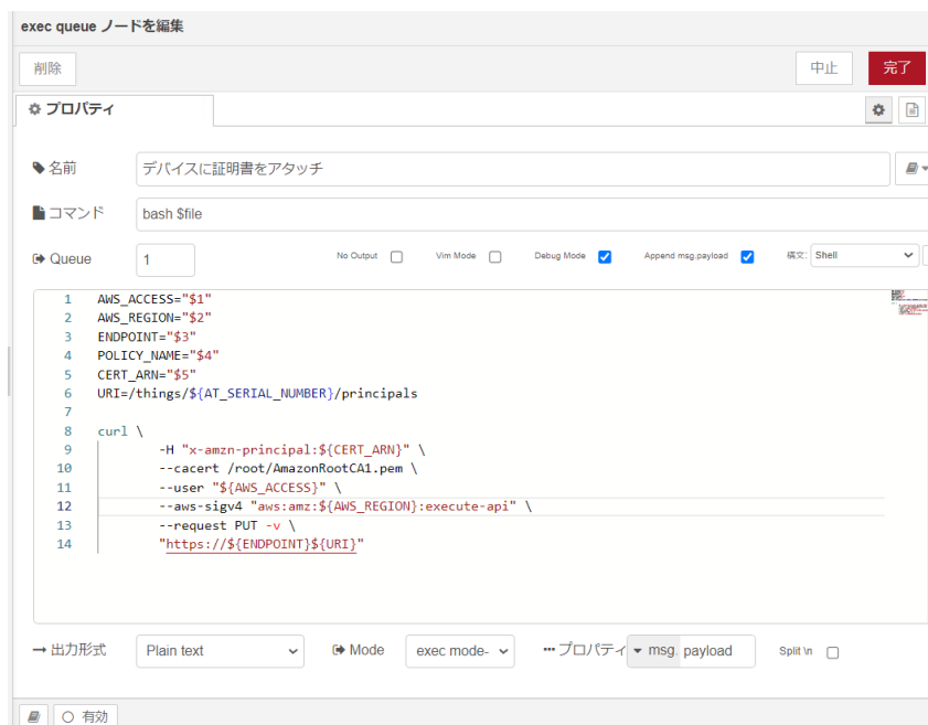
図 4.77 [証明書をデバイスにアタッチ] ノードのプロパティ内容
