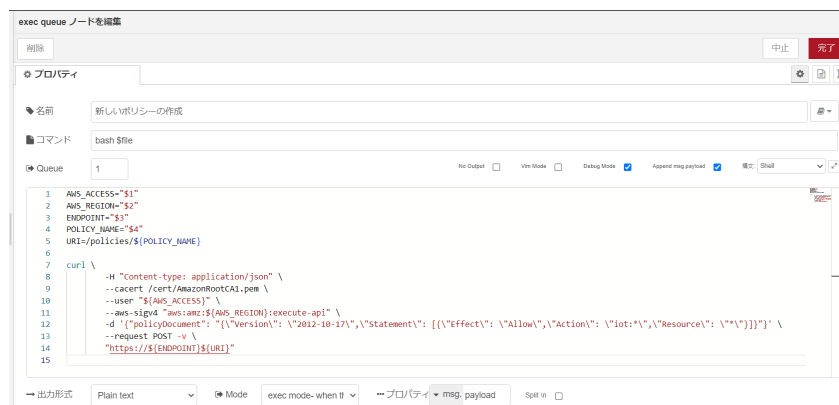
図 4.65 [新しいポリシーの作成] ノードのプロパティ内容
