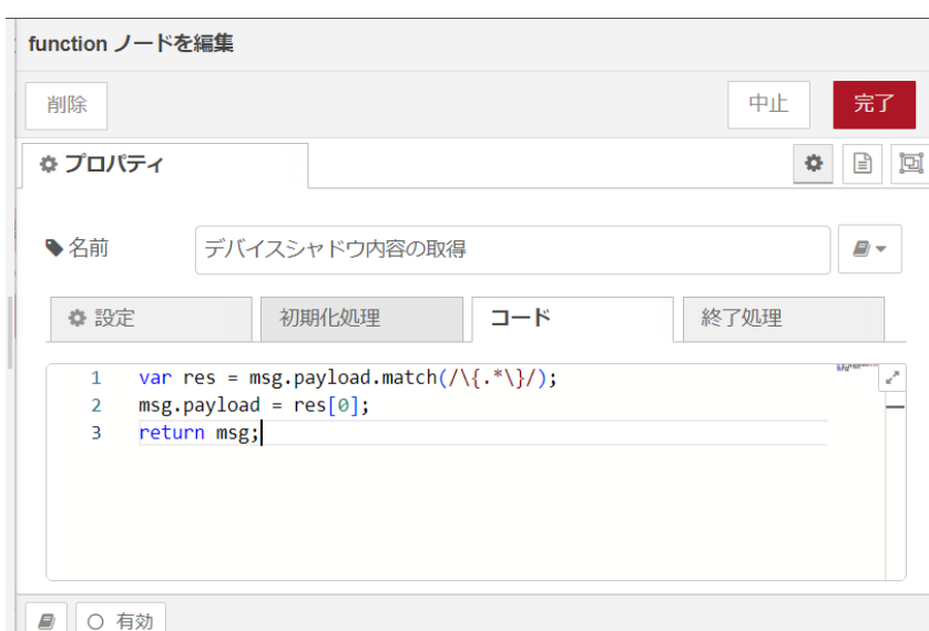
図 4.88 [デバイスシャドウ内容の取得] ノードのプロパティ内容
