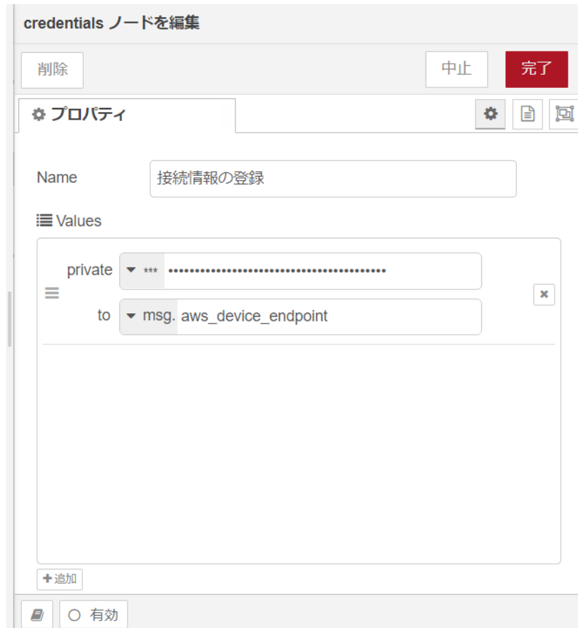
図 4.90 [接続情報の登録] ノードのプロパティ内容
