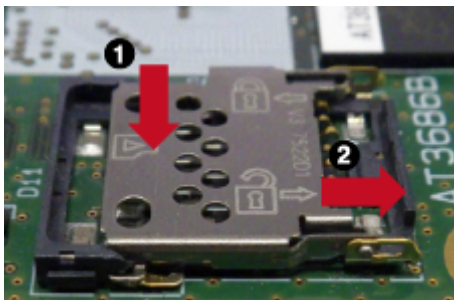
図 3.13 カバーのロックを解除する
