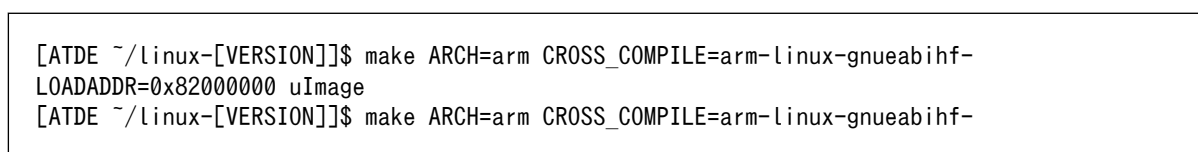
図 6.193 Linux カーネルのビルド
