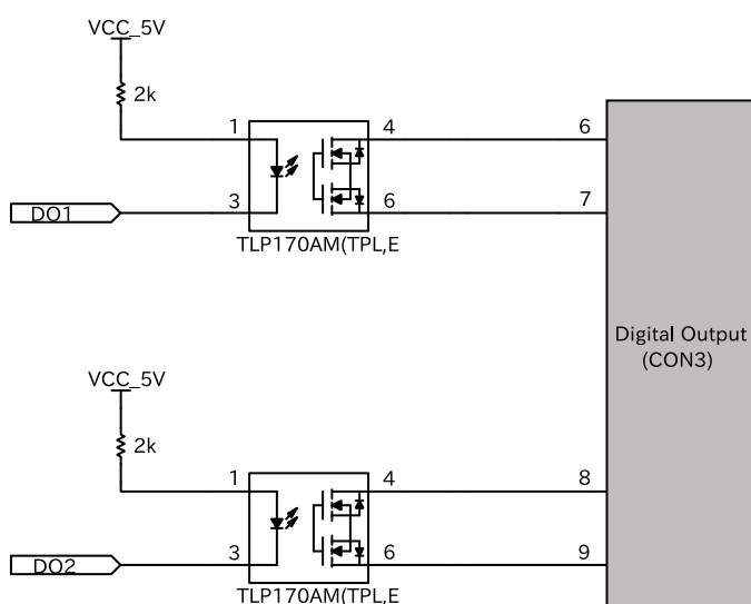
図 3.69 CON6 接点出力周辺回路
