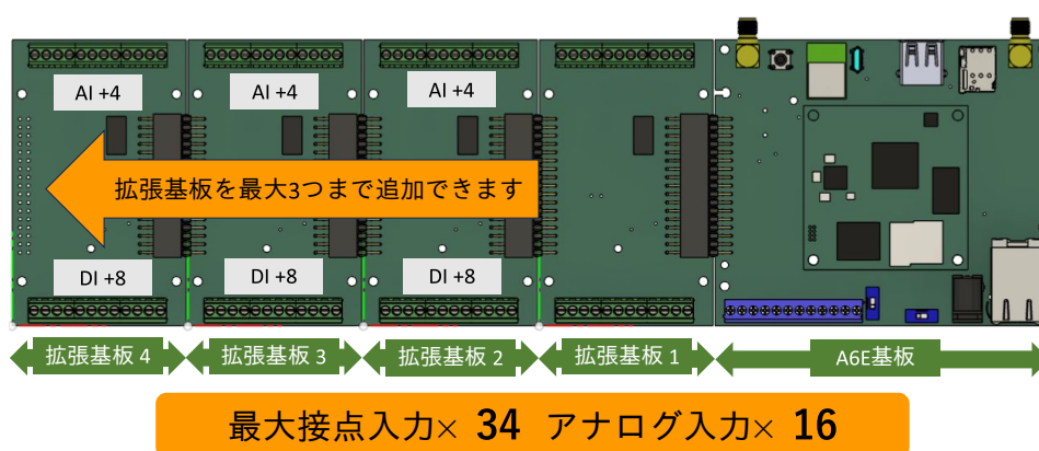
図 3.116 +Di8+Ai4 拡張基板のカスケード接続
