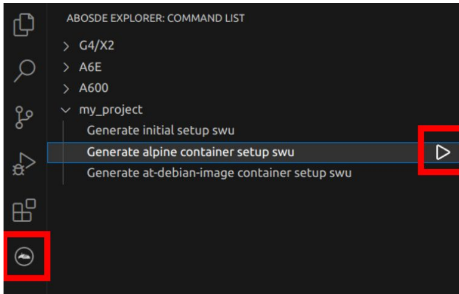
図 6.48 alpine のコンテナイメージをインストールする SWU ファイルを作成する
