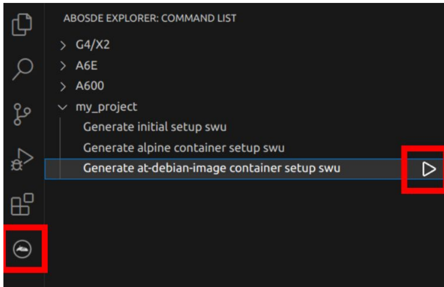
図 6.45 at-debian-image のコンテナイメージをインストールする SWU ファイルを作成する
