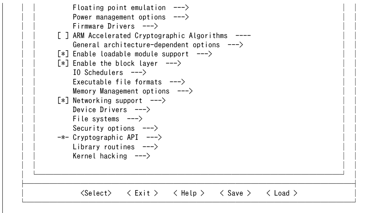
図 6.192 Linux カーネルコンフィギュレーション設定画面
