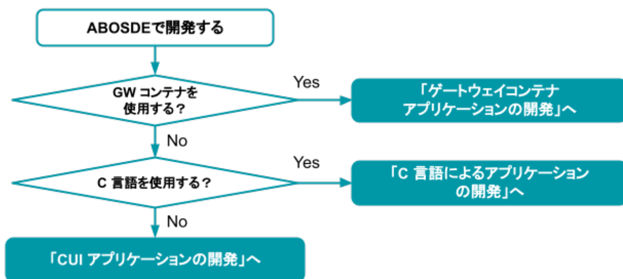
図 3.143 参照する開発手順の章を選択する流れ
