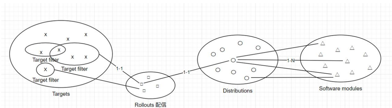
図 5.15 hawkBit が扱うソフトウェアのデータ構造
