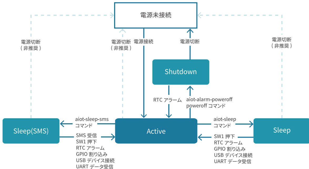
図 3.122 状態遷移図
