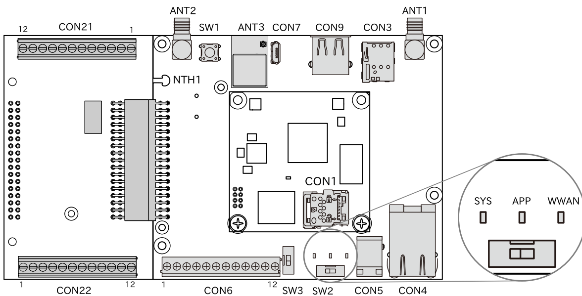
図 3.36 Armadillo-IoT ゲートウェイ A6E +Di8+Ai4 のインターフェース 表面
