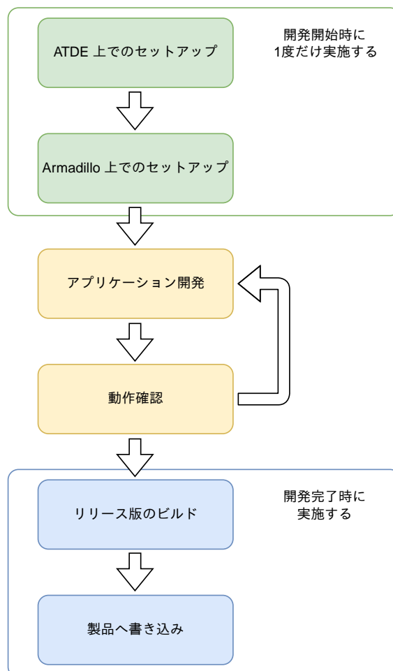
図 3.166 CUI アプリケーション開発の流れ
