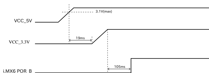
図 3.22 電源シーケンス
