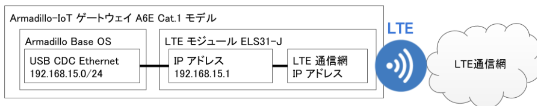
図 6.119 Cat.1 モデル (ELS31-J) LTE ネットワーク構成
