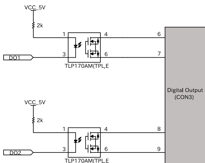
図 3.69 CON6 接点出力周辺回路
