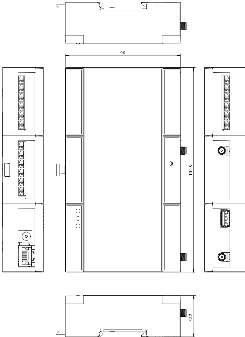
図 3.23 筐体形状
