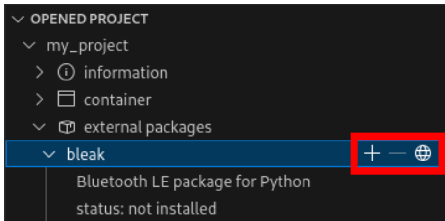
図 3.224 BLE パッケージをインストールする
