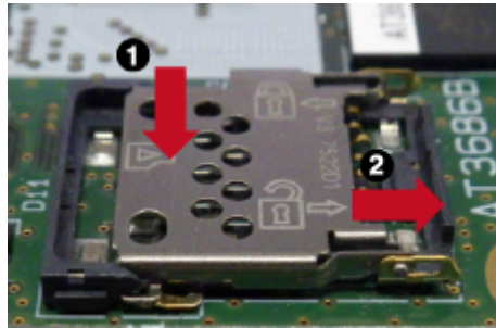
図 3.80 カバーのロックを解除する
