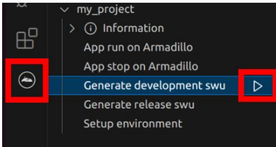
図 3.222 VS Code でコンテナイメージの作成を行う
