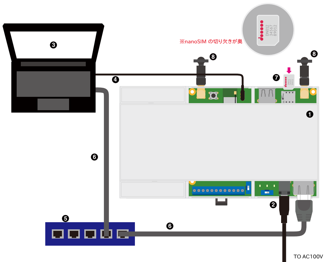
図 3.53 Armadillo-IoT ゲートウェイ A6E +Di8+Ai4 の接続例
