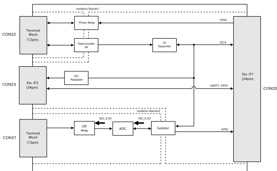
図 6.243 +Di8+Ai4 拡張基板のブロック図
