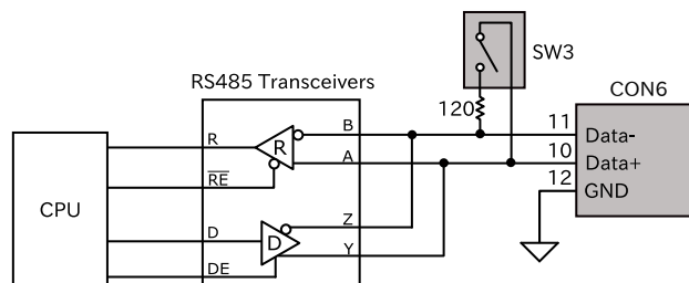
図 3.116 CON6 RS-485 トランシーバ周辺回路
