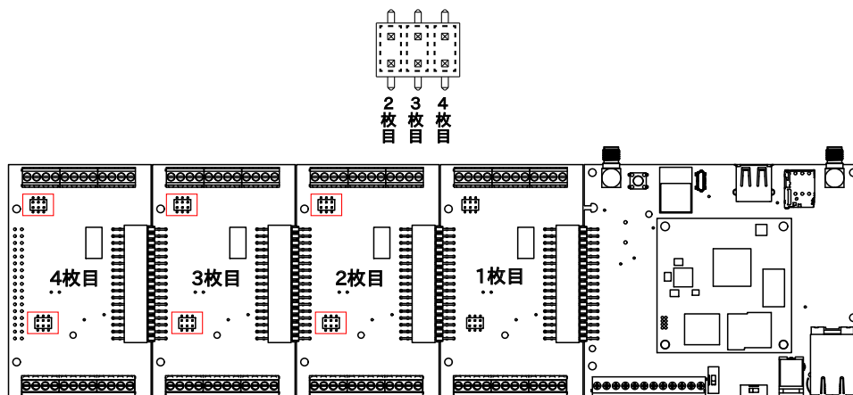
図 3.162 ピンヘッダの位置と設定
