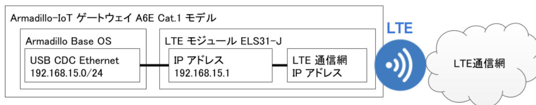
図 6.140 Cat.1 モデル (ELS31-J) LTE ネットワーク構成
