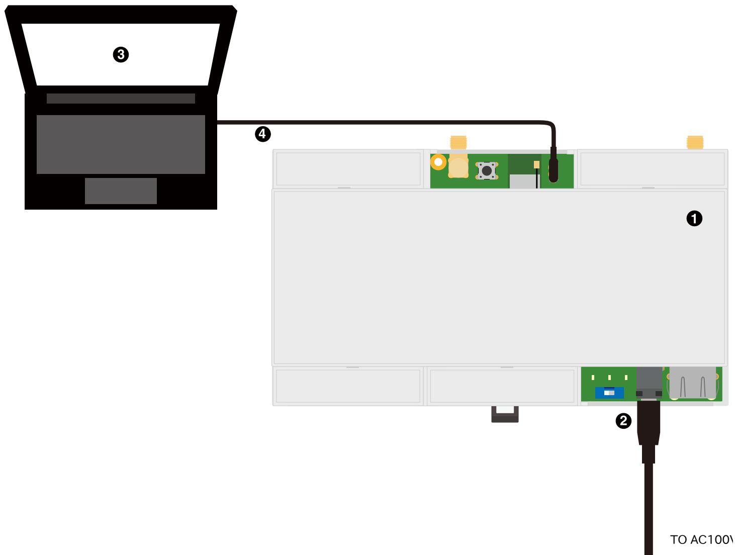
図 3.47 シリアルコンソールを使用する配線例
