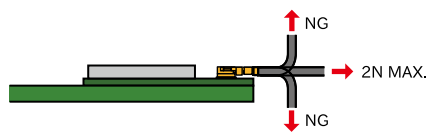
図 3.77 WLAN 基板アンテナのケーブル引き回し
