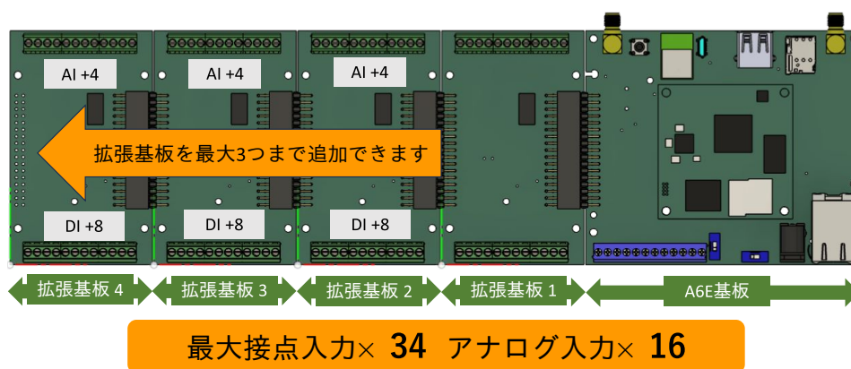
図 3.159 +Di8+Ai4 拡張基板のカスケード接続
