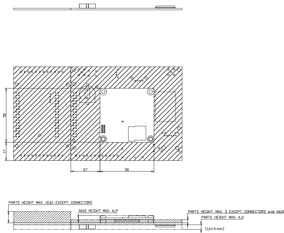
図 3.61 部品高さ
