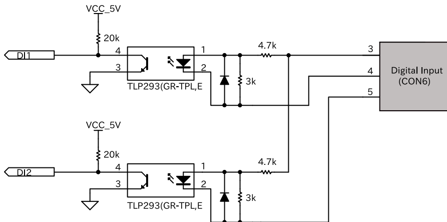
図 3.106 CON6 接点入力周辺回路
