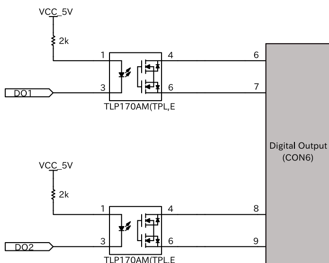
図 3.111 CON6 接点出力周辺回路
