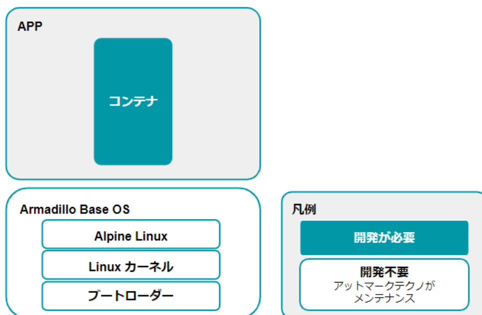
図 3.163 開発者が開発するもの、開発しなくていいもの
