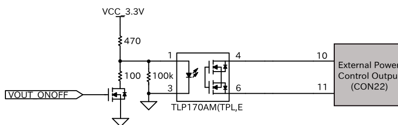
図 3.155 CON22 外部電源制御出力周辺回路
