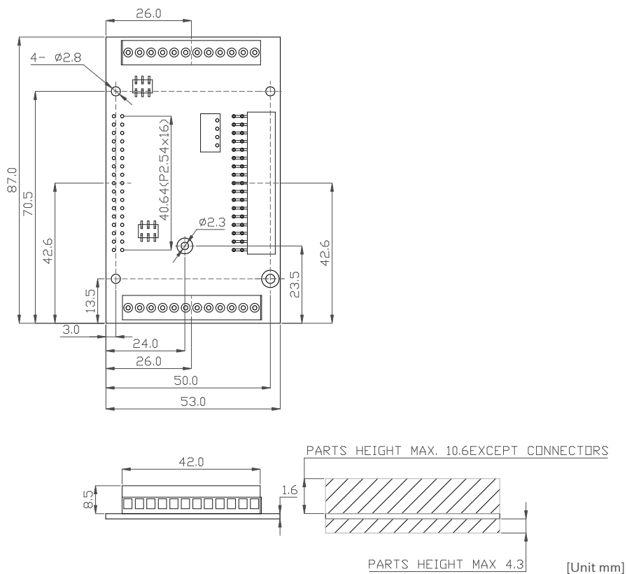
図 6.245 +Di8+Ai4 拡張基板基板形状図
