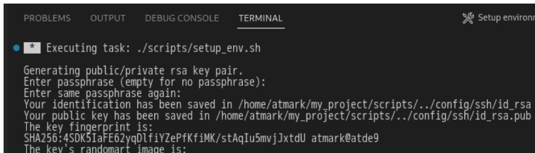
図 3.253 VS Code のターミナル
