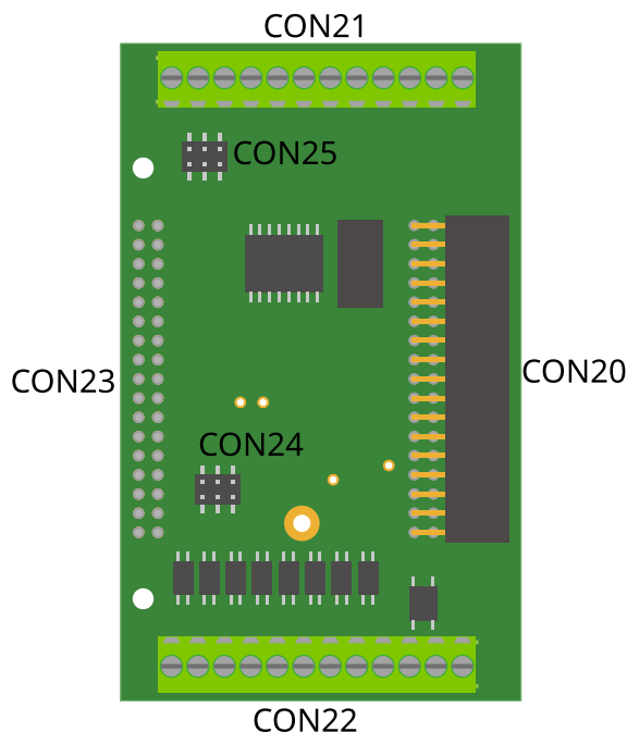
図 6.244 +Di8+Ai4 拡張基板のインターフェースレイアウト
