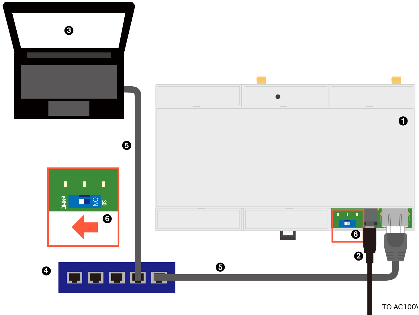
図 3.23 ABOS にアクセスするための接続
