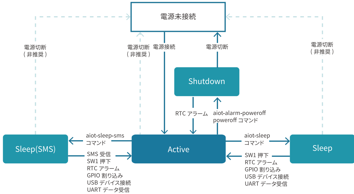
図 3.165 状態遷移図
