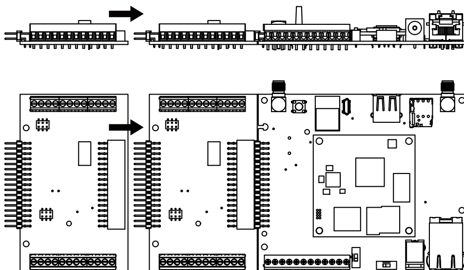
図 3.160 +Di8+Ai4 拡張基板の組付け方法
