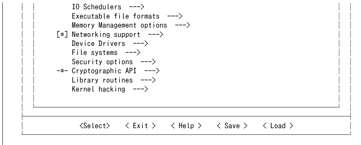
図 6.216 Linux カーネルコンフィギュレーション設定画面
