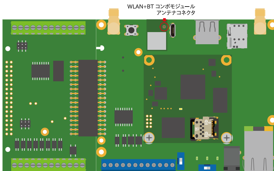
図 3.70 WLAN+BT コンボモジュールのアンテナコネクタの位置
