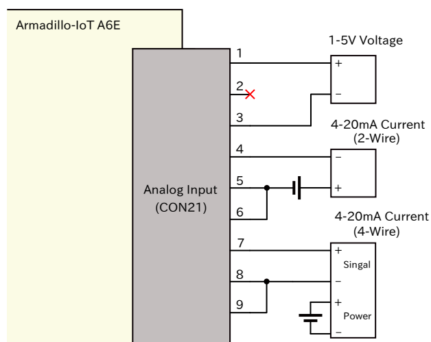
図 3.144 CON21 アナログ入力接続例
