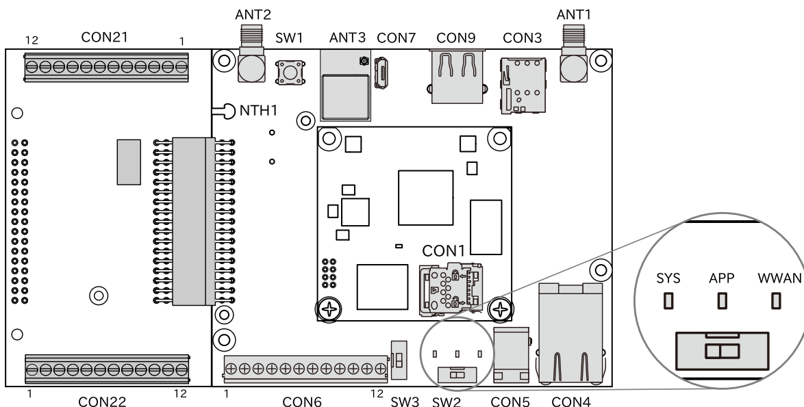
図 3.78 Armadillo-IoT ゲートウェイ A6E +Di8+Ai4 のインターフェース 表面
