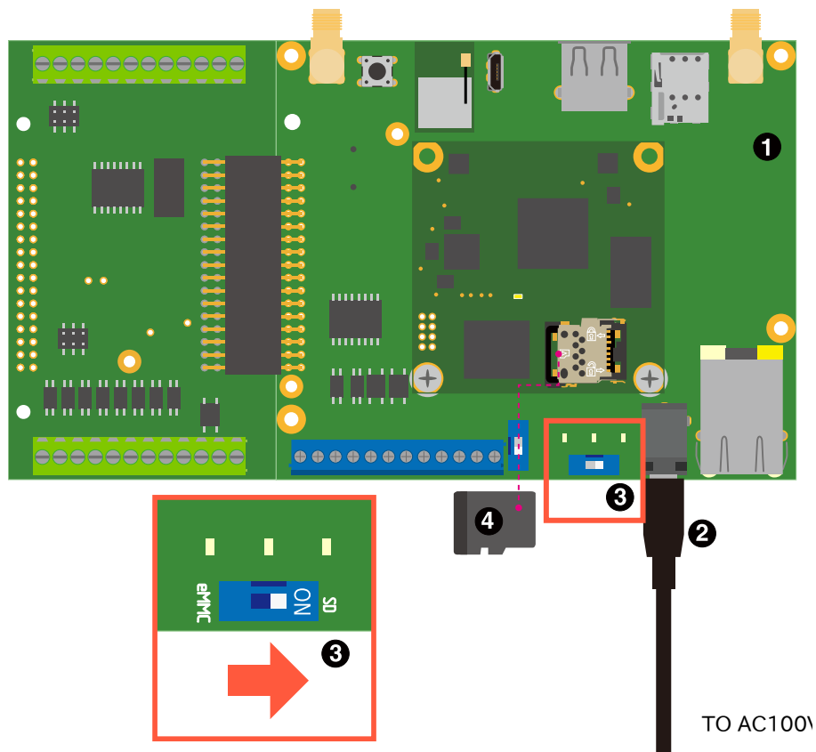
図 3.19 Armadillo-IoT ゲートウェイ A6E +Di8+Ai4 を初期化する接続
