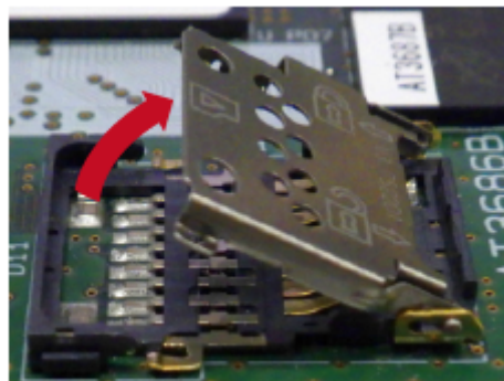
図 3.81 カバーを開ける
