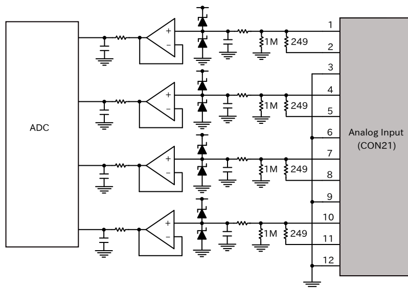
図 3.143 CON21 アナログ入力周辺回路
