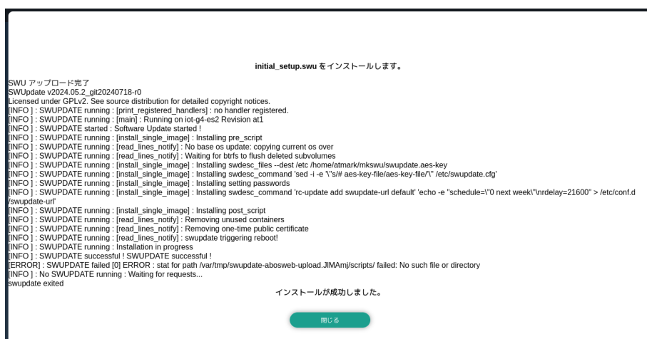
図 3.32 SWU インストールに成功した画面
