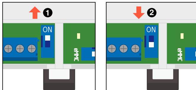
図 3.117 スwitchの状態と終端抵抗の ON/OFF
