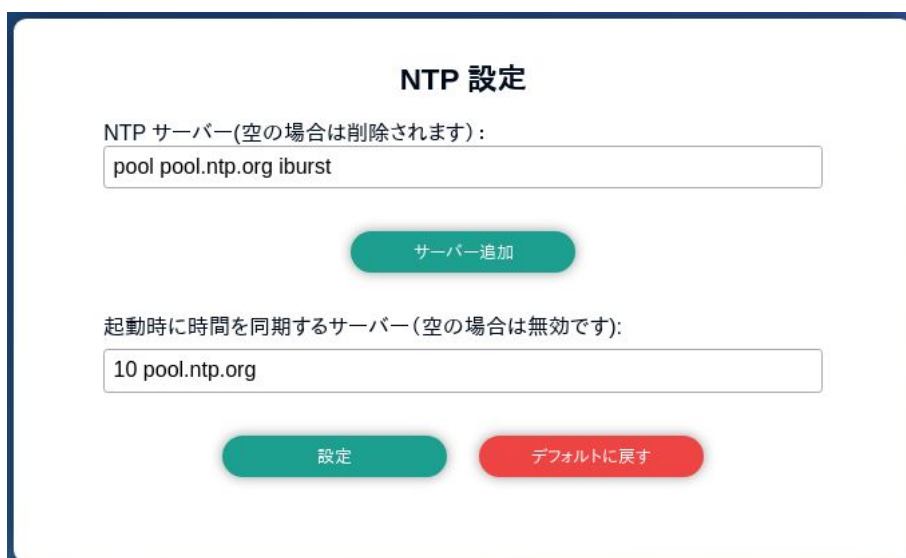
図 6.105 ネットワークタイムサーバーの設定項目
