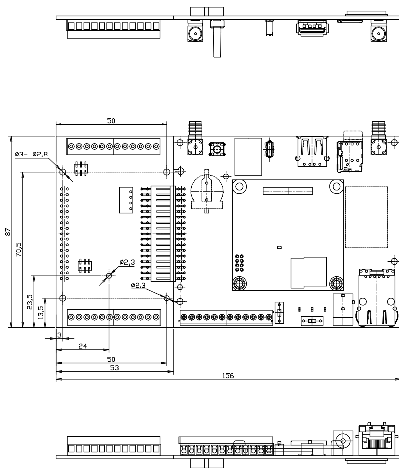
図 3.58 基板形状および固定穴寸法 2
